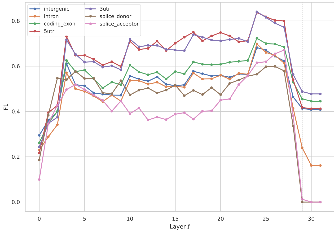
(H4) Per-layer per-class F1 score
