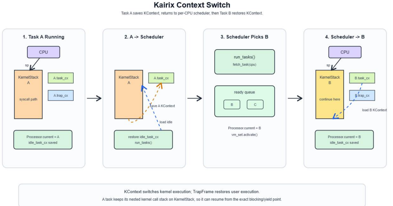
上下文切换示意图
