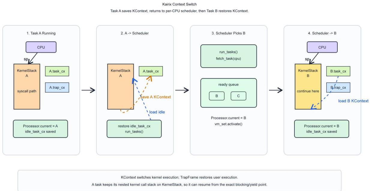
图3-2:switch
