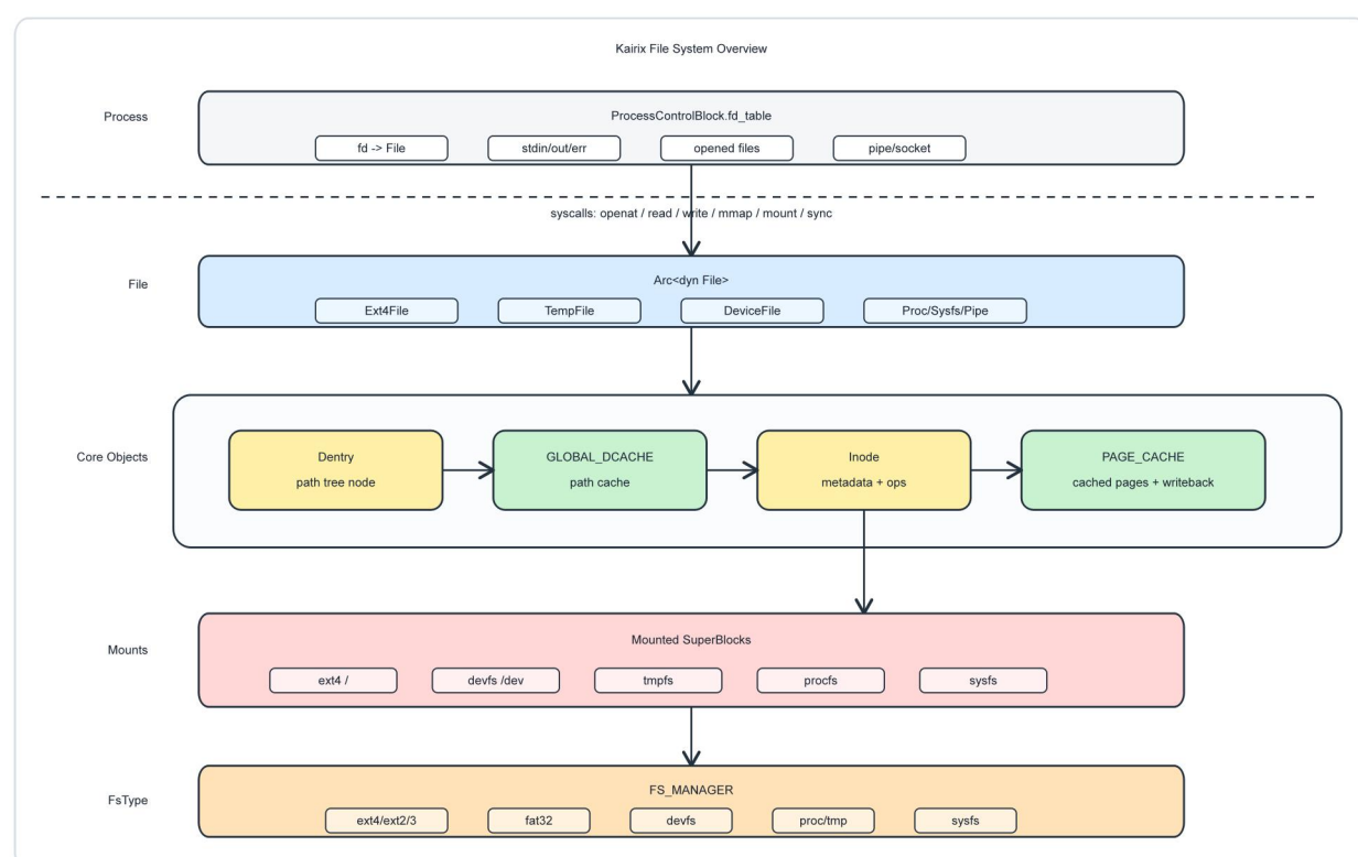
图5-1 VFS总览
