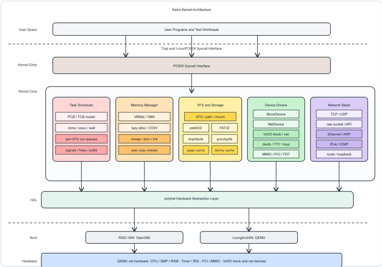
图 1-1: 总体架构
