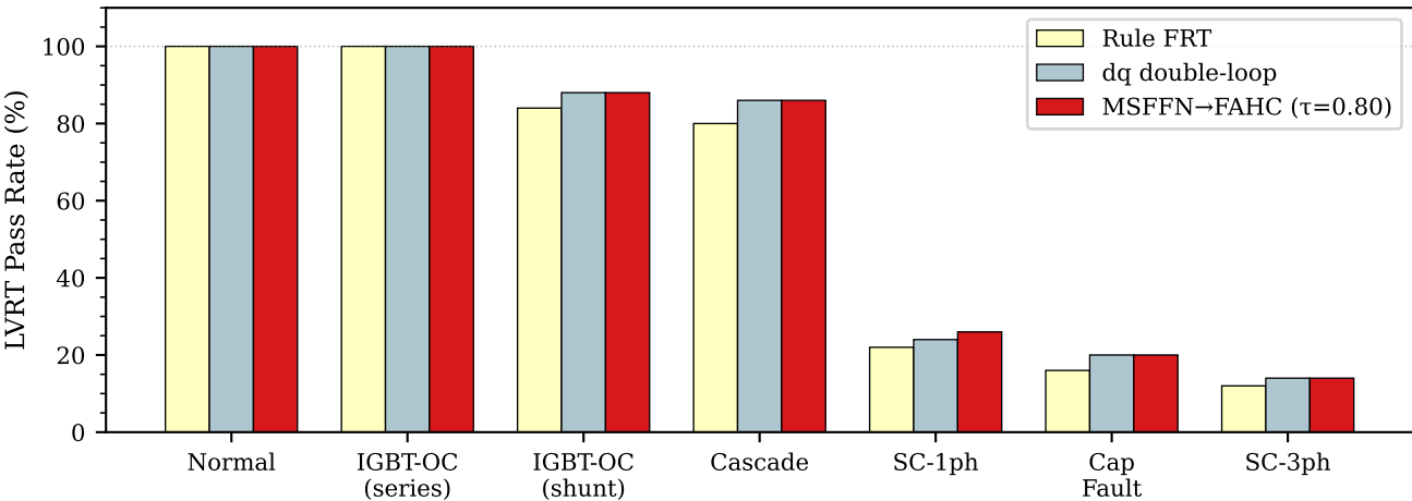
(d) Per-Class LVRT Pass Rate
