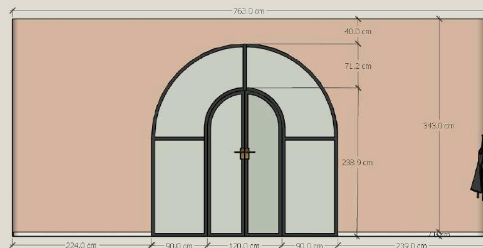
VUE ARRIÈRE
