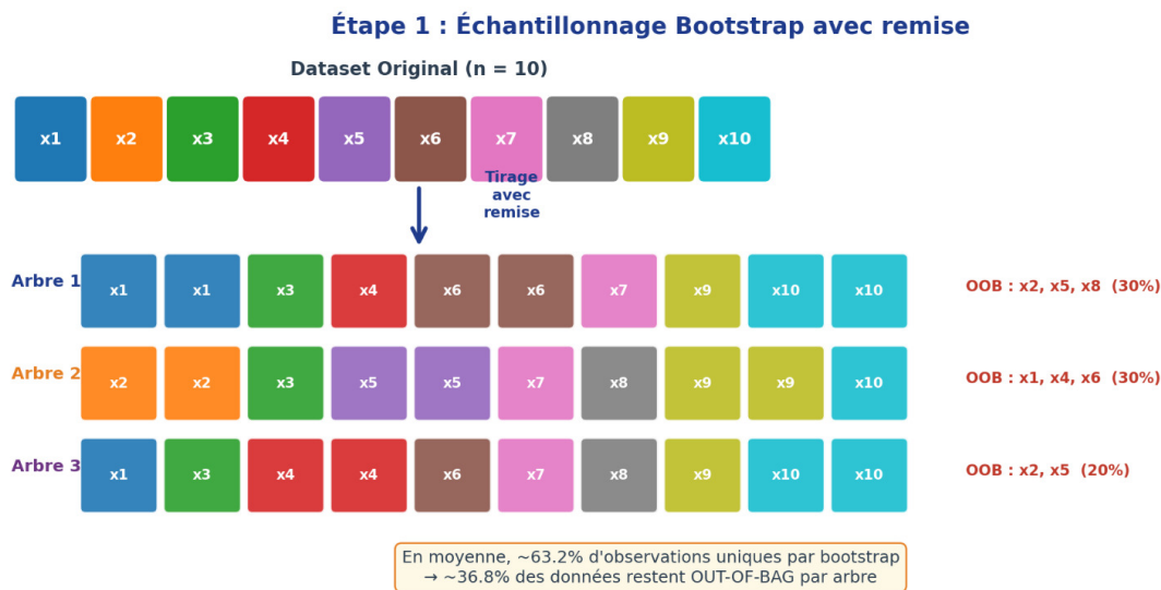
FIGURE 2.11 – L'erreur OOB
