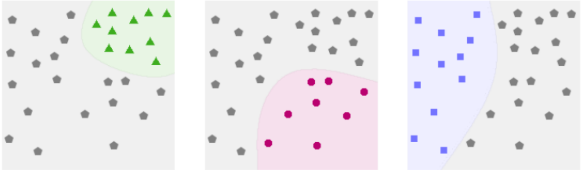
FIGURE 1.10 – À gauche, le SVM spécialisé dans la reconnaissance des guêpes, au centre dans la reconnaissance des frelons et à droite des abeilles (on suppose qu'on a trouvé un kernel trick approprié à chaque fois, afin d'obtenir une frontière non linéaire)
