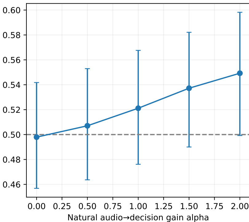
ROC-AUC
