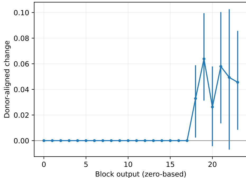
Final-norm logit lens
