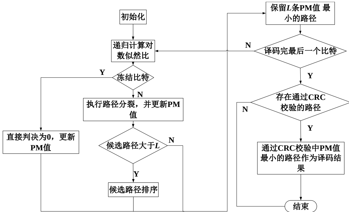
图 2-9 CA-SCL 译码算法流程图
