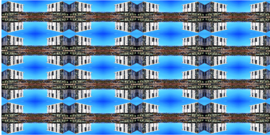
Processus de périodisation d'une image
