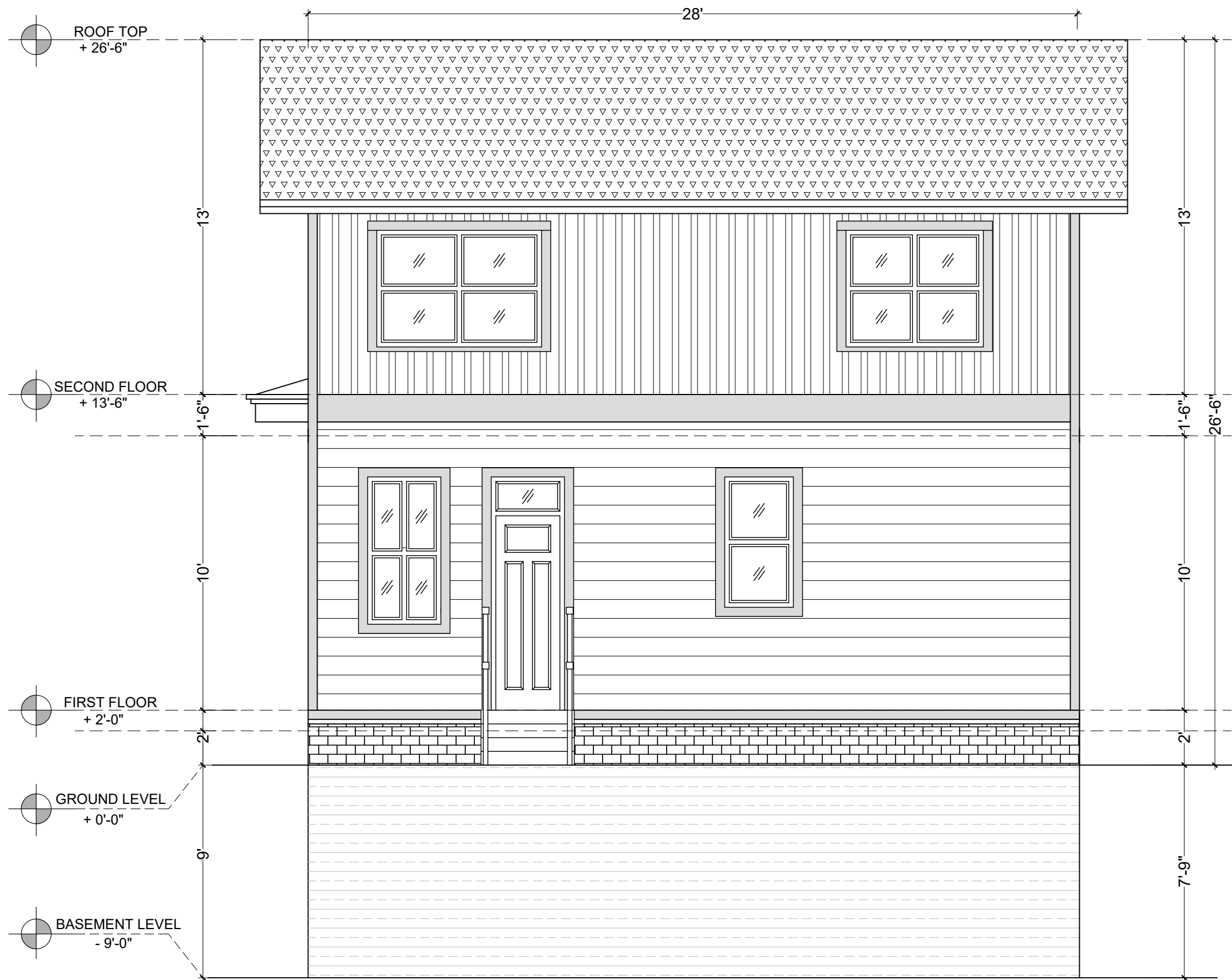
ELEVATION-04 SCALE: 1/4" = 1'-0"
