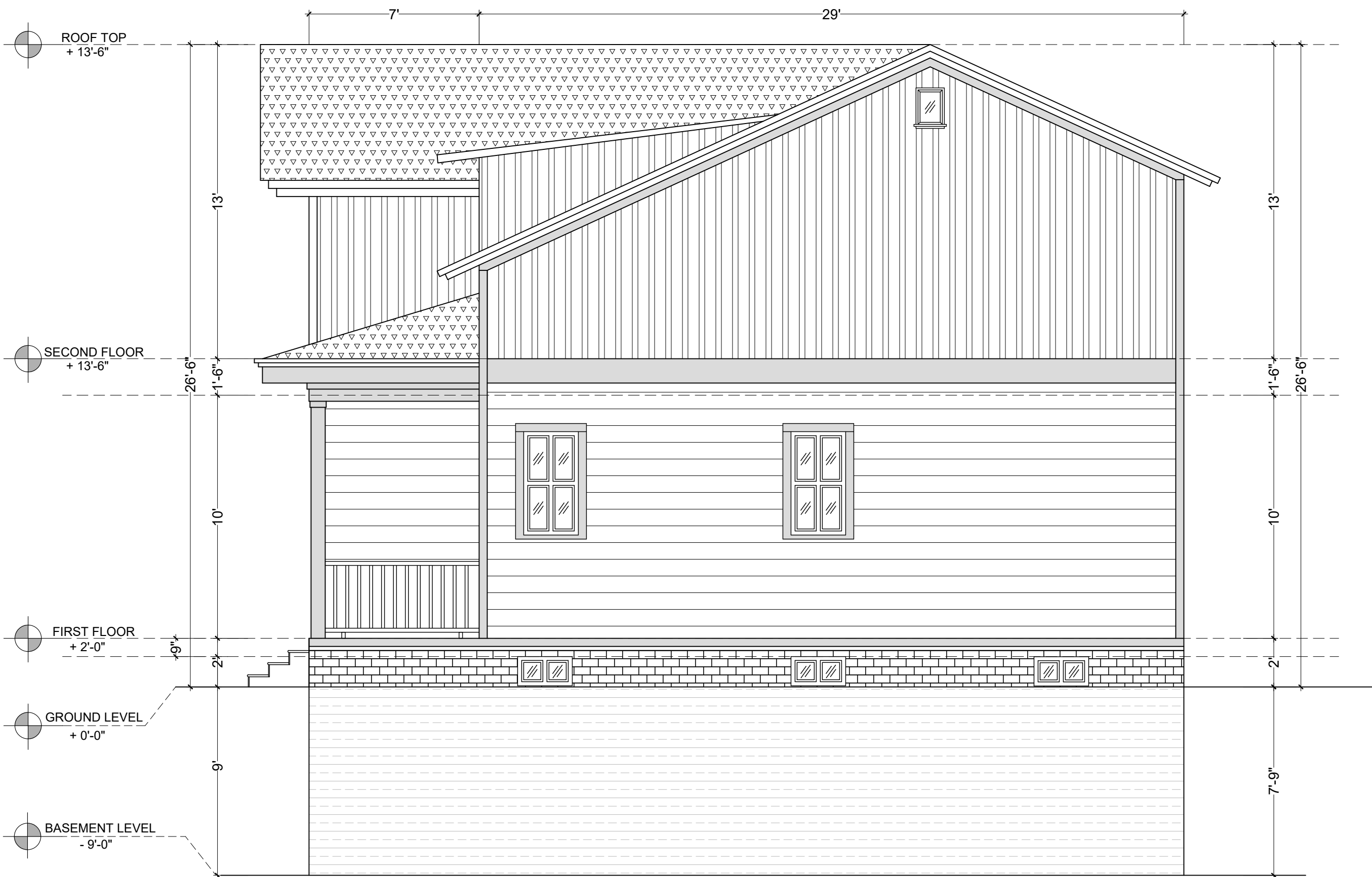
ELEVATION-02 SCALE: 1/4" = 1'-0"
