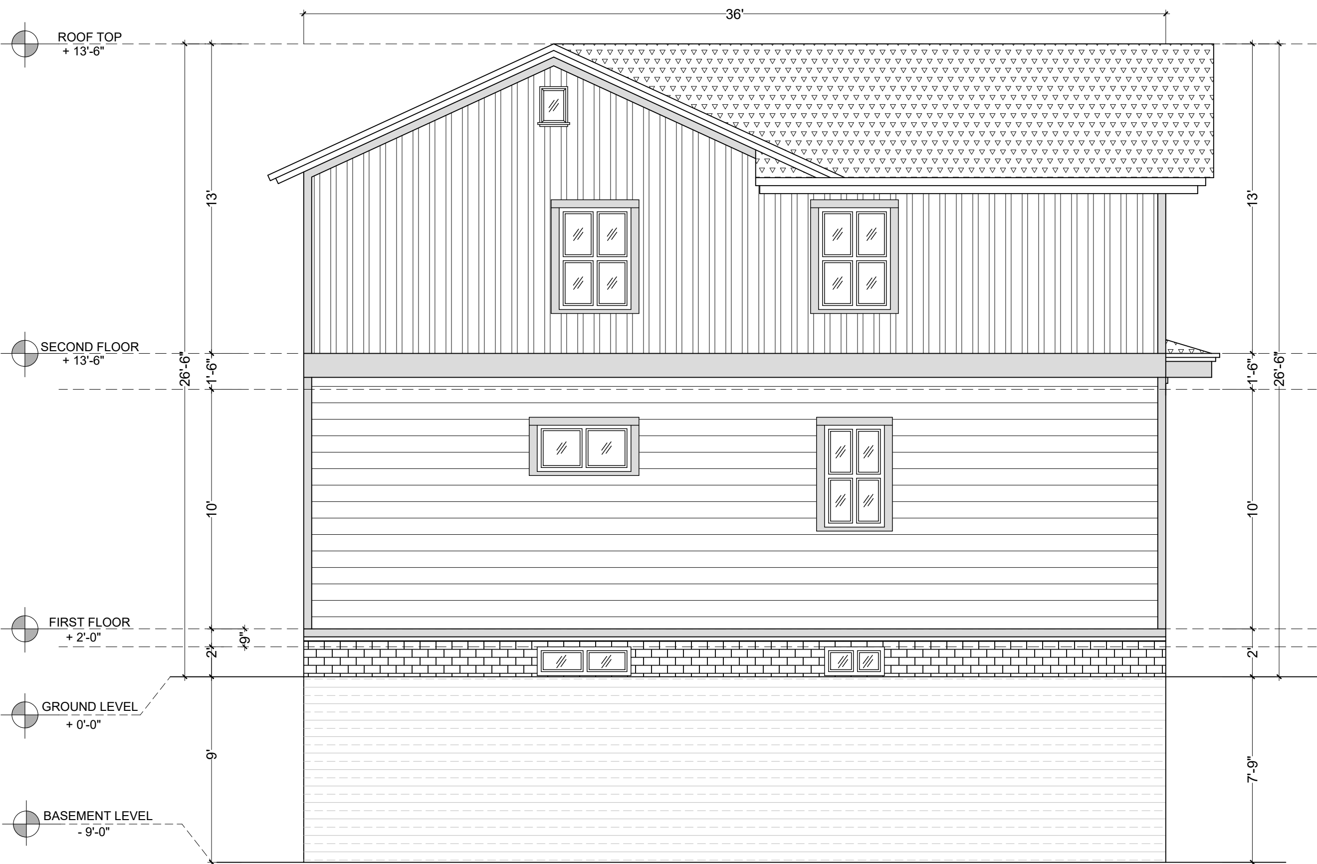
ELEVATION-03 SCALE: 1/4" = 1'-0"
