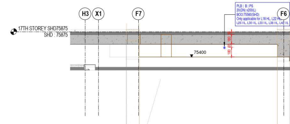
15 Section - 18 1 : 25
