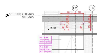
14 Section - 17 1 : 25
