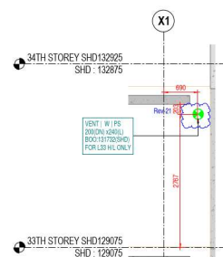
22 Section - 31 1 : 50
