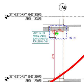
21 Section - 30 1 : 50
