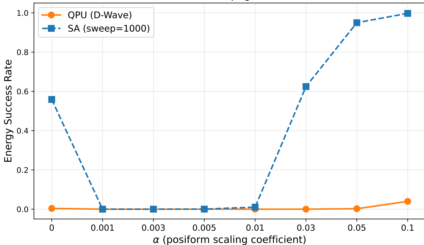
QPU vs SA — pegasus, lin2
