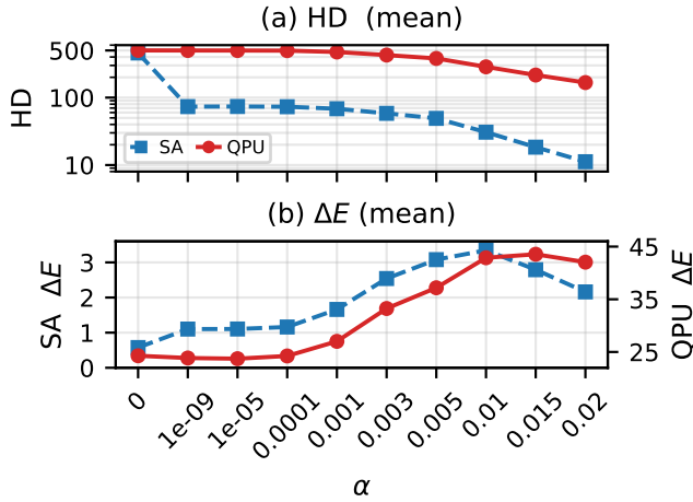
Fig. 1. 동일한 100 개 최난해 인스턴스의 실패-조건부 난이도(표시된 모든 \alpha 에서 집단이 합산 읽기의 \geq 91\% 를 실패). 파랑: SA; 빨강: D-Wave Advantage 어닐러. (a) HD는 로그축 – 둘 다 단조 감소하나 0에 닿지 않아 실패는 비트로는 멀다. (b) \Delta E = \Delta R + \alpha \Delta P , 좌우 분리 축(좌 SA, 우 QPU): 작은 \alpha 구간에서 \Delta R 바닥이 평탄하다가 \alpha P 가 두드러지며 \alpha=10^{-2} 부근에서 비단조 정점. 어닐러가 한 자릿수 큰 절대 바닥 위에서 같은 정성적 형태를 재현한다.
