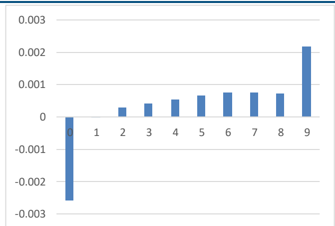
图 13:因子分组平均收益
