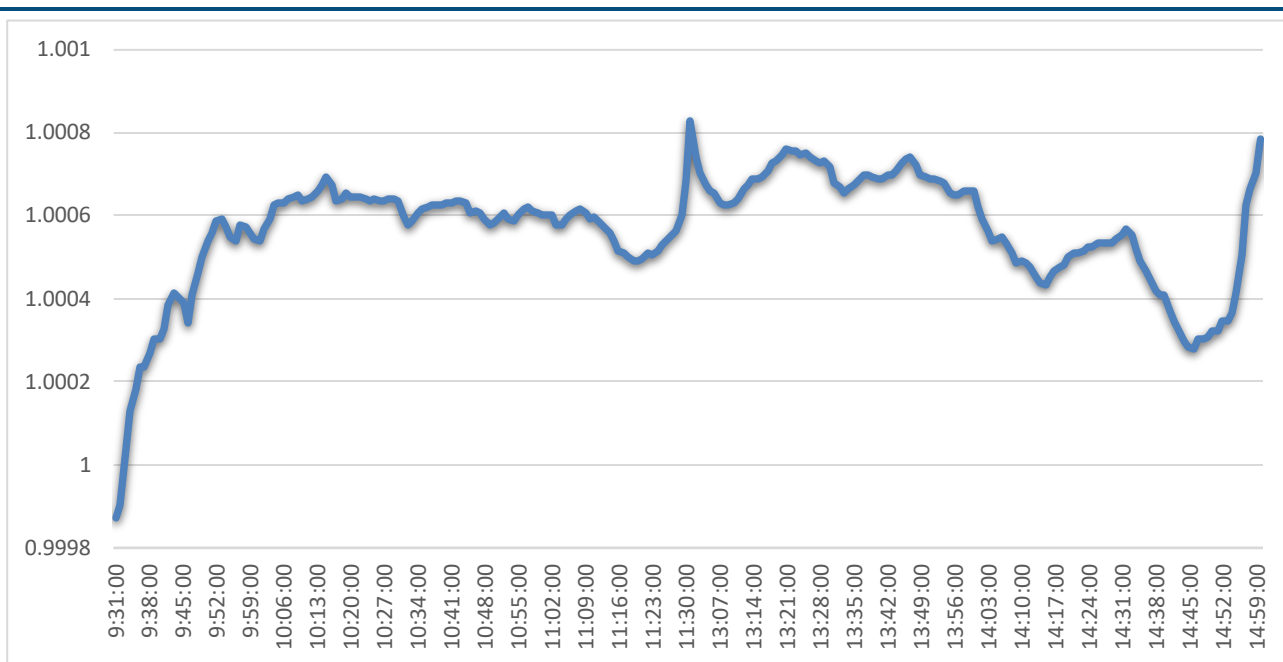
图 1: 日内股价形态
