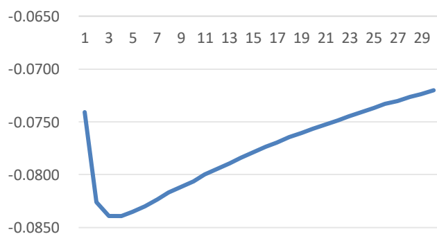
图 6: 不同频率收益率上行波动率因子 IC
