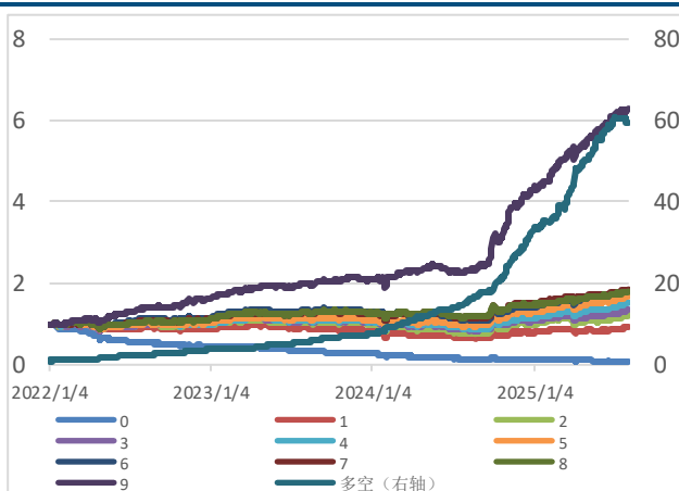
图 12:因子分组累计净值
