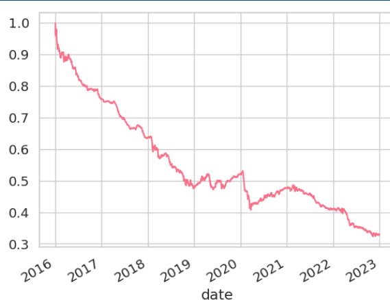
图 3:沪深 300 隔夜累计净值
