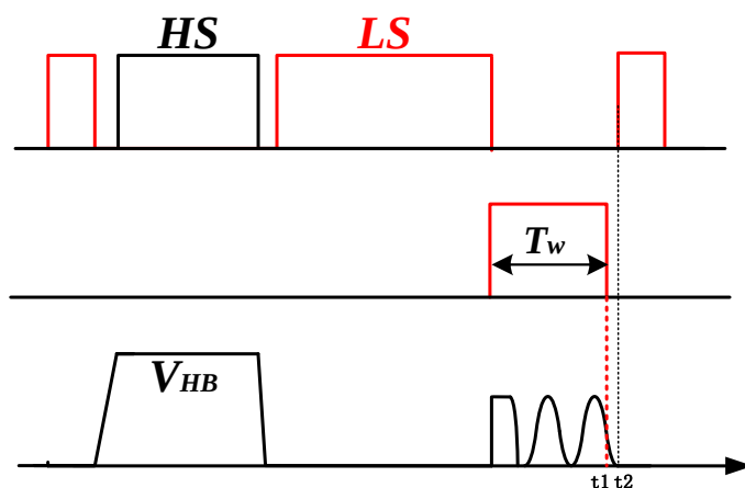
图 3.7 谷值锁定波形 1
