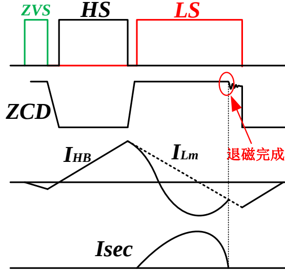
图 3.14 退磁时间谐振波形图
