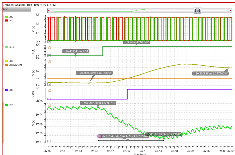
图 5.7 负载 2.5-5A 跳变仿真波形图
