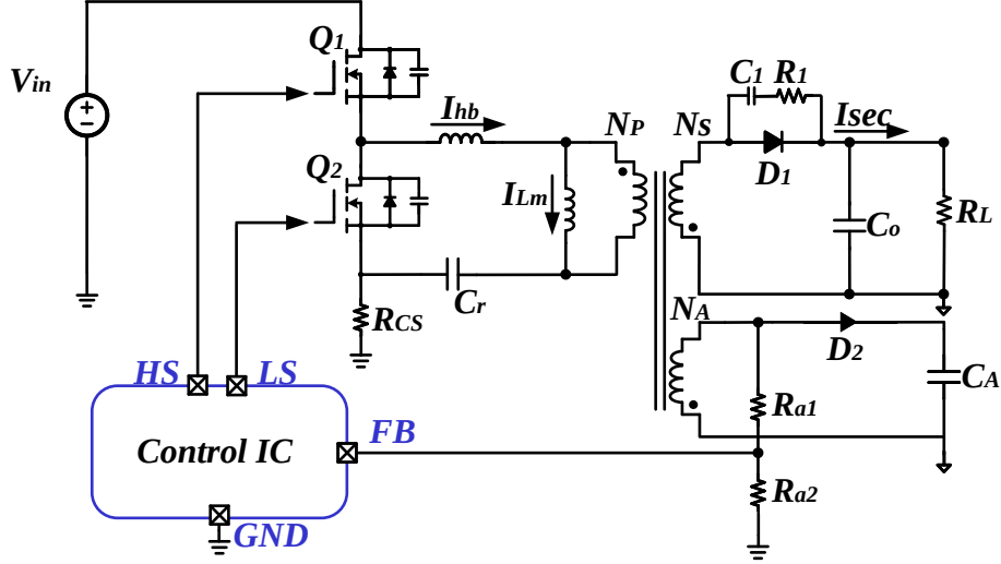
图 2.12 原边反馈电路电路图
