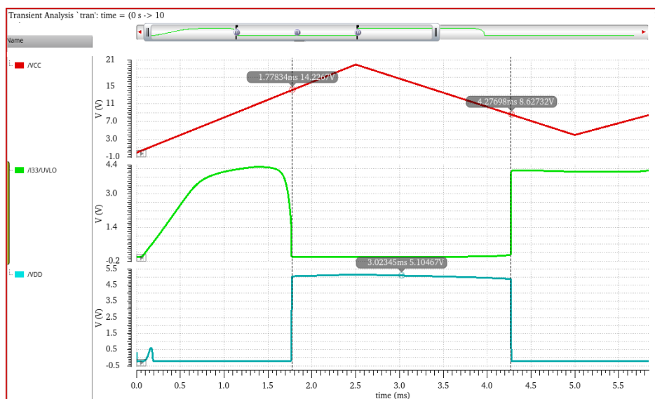
图 4.2 压锁定和电压调整电路仿真波形图
