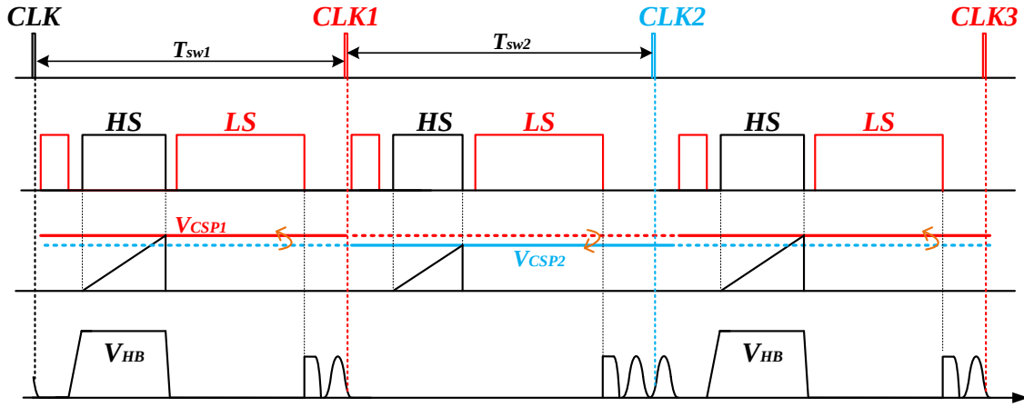
图 3.8 跳谷现象波形图
