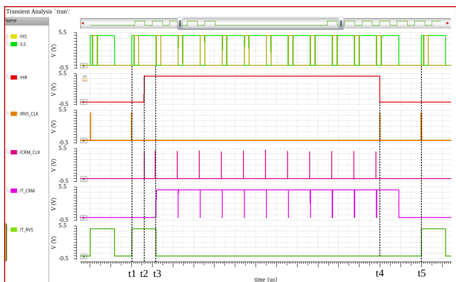
图 4.40 逻辑控制电路具体仿真波形图
