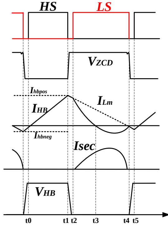
图 2.4 CRM 工作模式波形图
