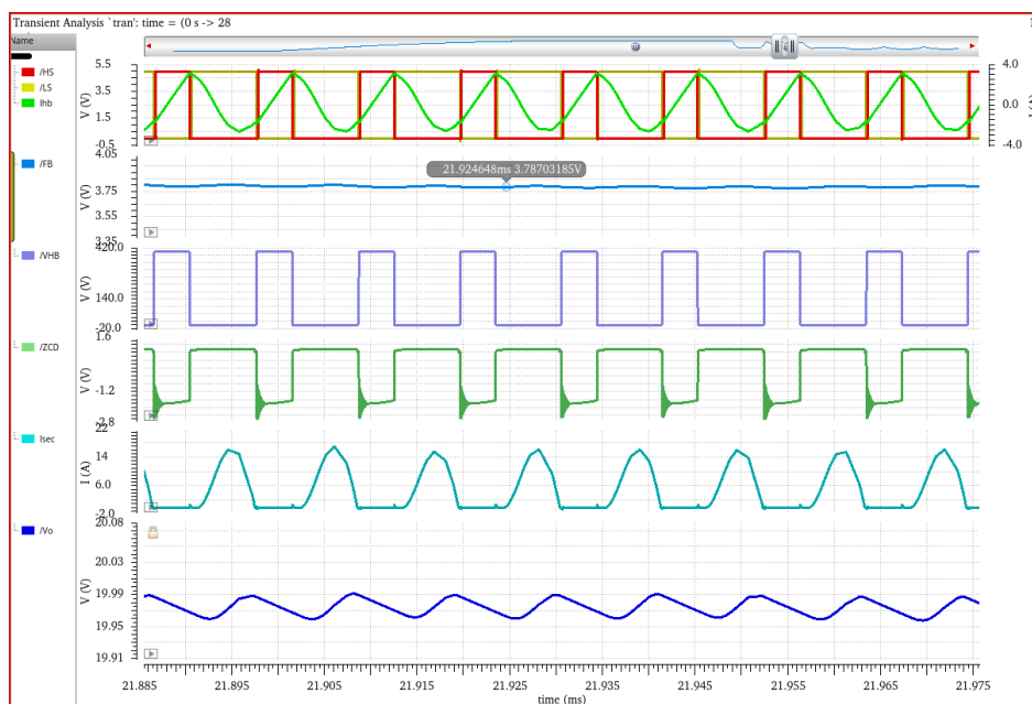
图 5.3 满载电路仿真波形图
