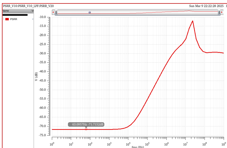
图 4.7 带隙基准电路 PSRR 仿真波形图
