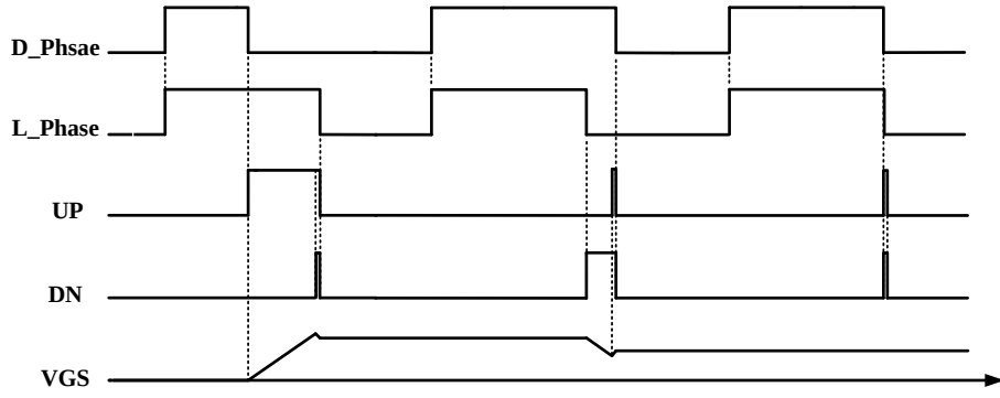
图 4.23 鉴相鉴频器电荷泵波形图
