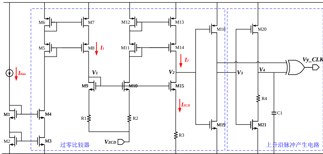
图 4.8 过零检测电路原理图
