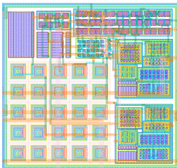
图 5.9 带隙基准电路版图
