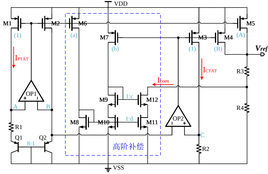
图 4.3 带隙基准电路原理图
