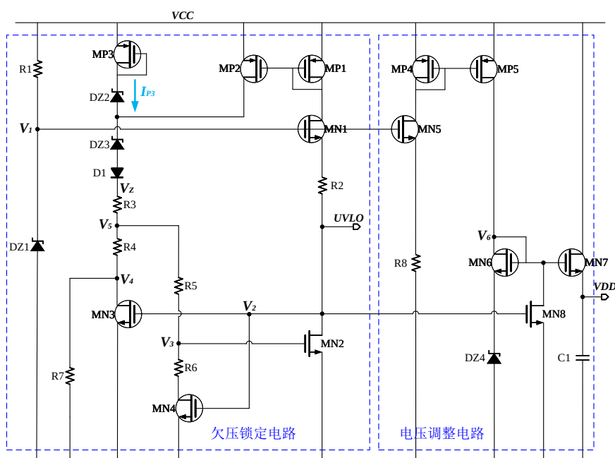
图 4.1 欠压锁定和电压调整电路原理图
