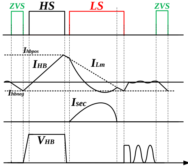
图 3.4 ZV-RVS 工作模式波形图
