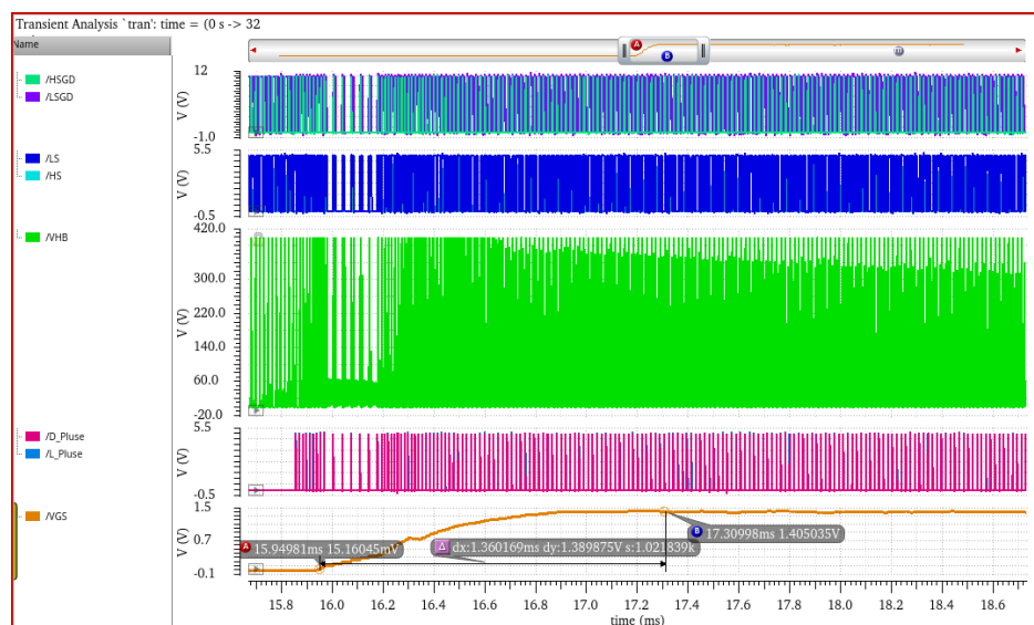
图 4.26 精确谷底导通电路相关波形仿真图
