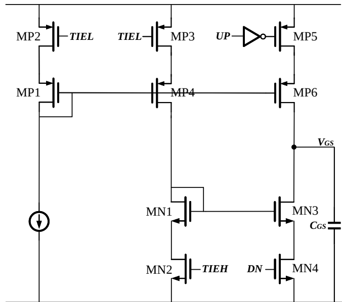
图 4.24 电荷泵电路图
