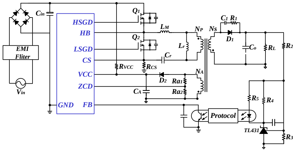
图 3.1 非对称半桥反激式外围拓扑结构图
