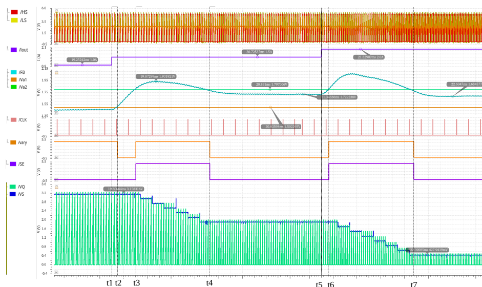
图 4.15 多周期谷值锁定电路波形图
