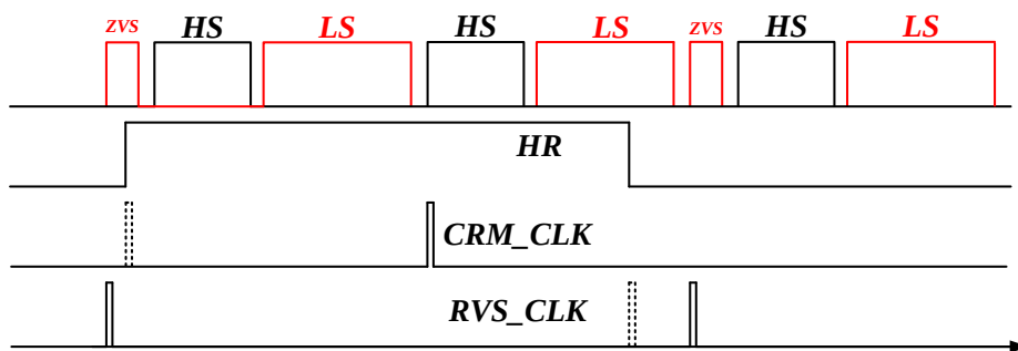
图 4.39 不同工作模式切换波形图
