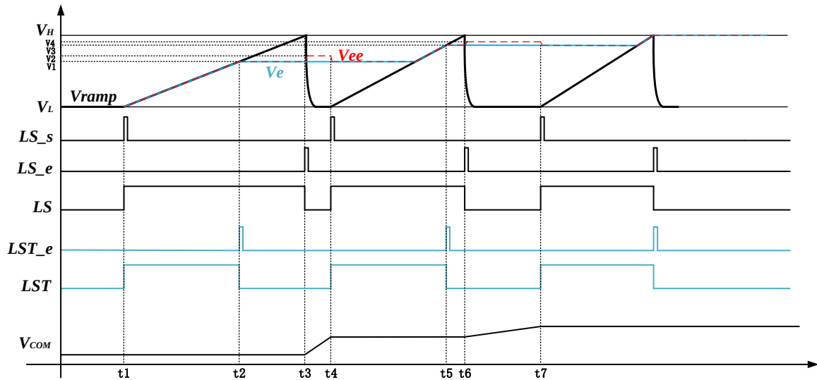
图 4.32 动态校准模块工作波形图
