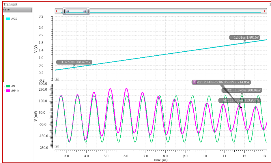
图 4.21 压控高通滤波器仿真波形图
