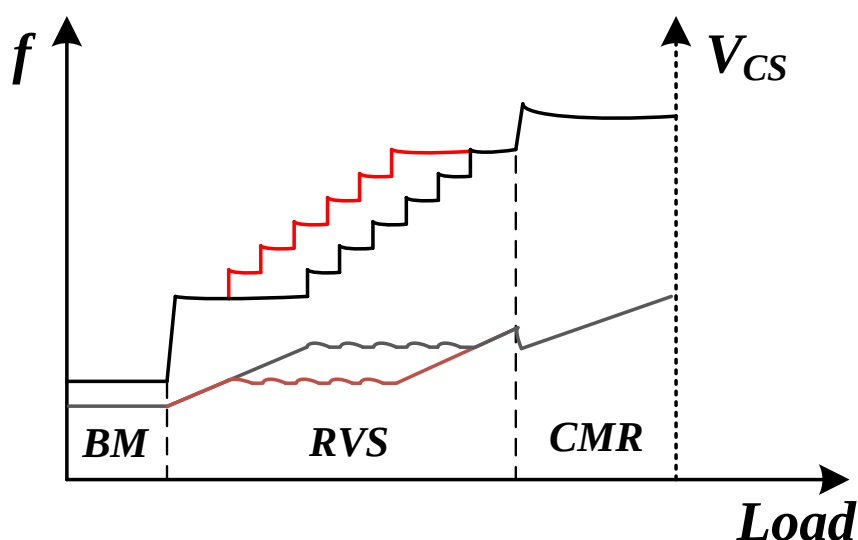
图 3.6 多模式频率变化图
