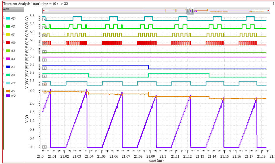
图 4.14 DAC 电路仿真波形图
