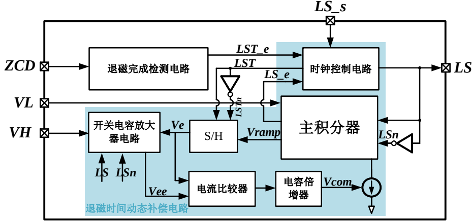
图 4.28 退磁时间动态校准模块框图
