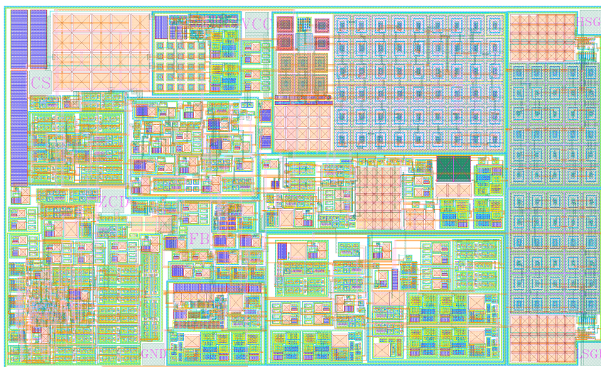
图 5.10 整体电路版图
