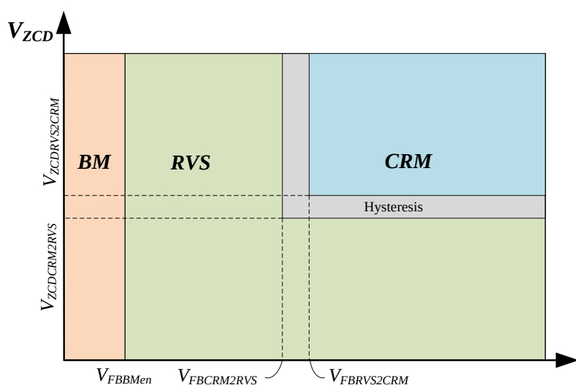
图 3.5 多模式切换图
