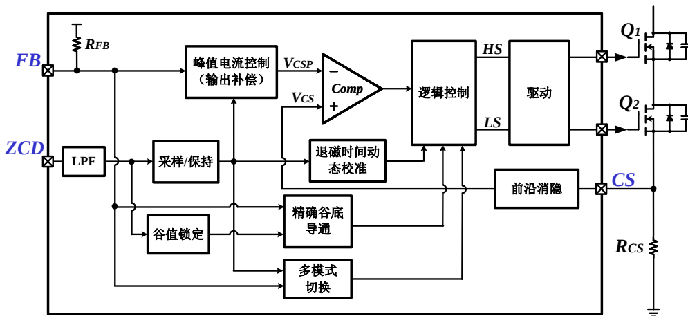
图 3.13 恒压控制模式框图
