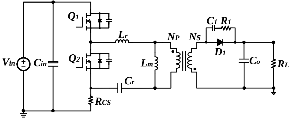
图 2.3 非对称半桥反激式拓扑图
