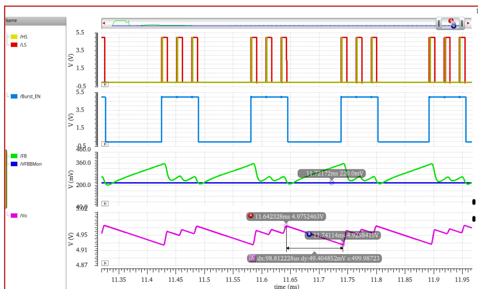
图 5.6 空载电路仿真波形图
