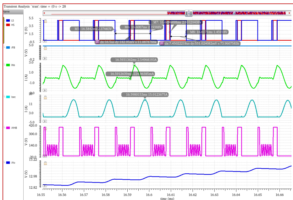
图 5.2 恒流控制模式仿真波形图
