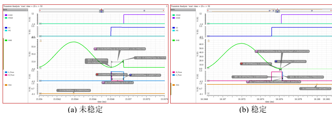
图 4.27 谷底导通放大仿真图
