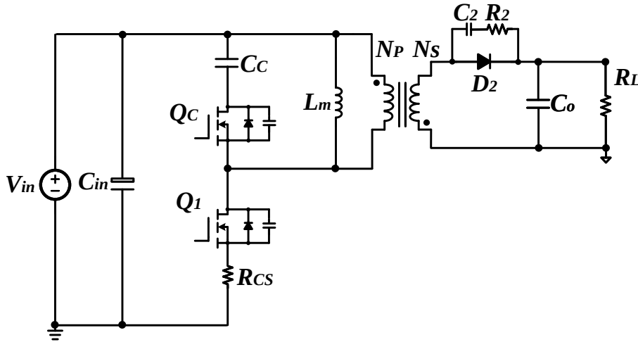
图 2.2 有源钳位反激式拓扑图
