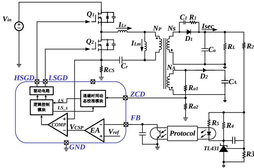
图 3.15 退磁时间动态校准技术框图
