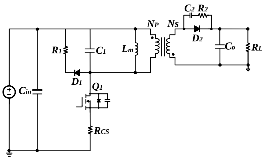
图 2.1 传统反激式拓扑图
