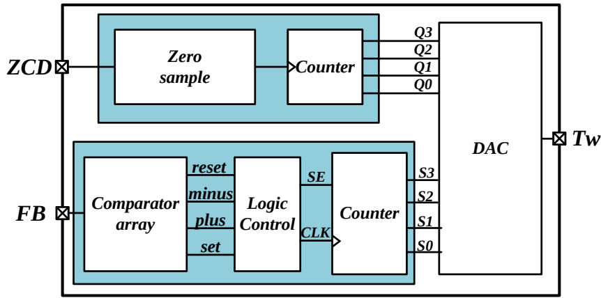
图 3.10 谷值锁定电路框图
