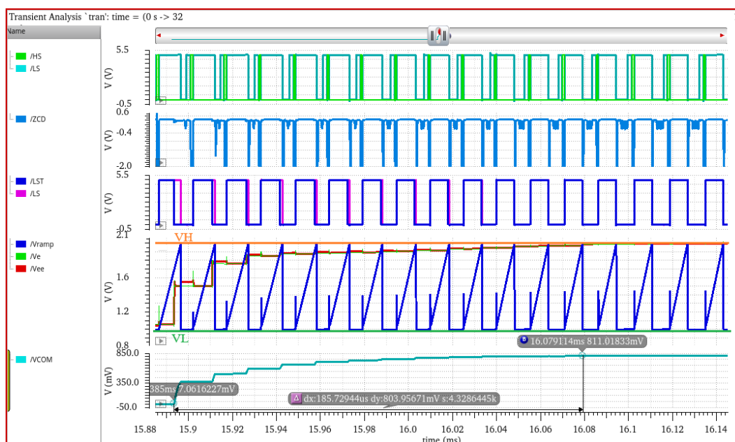
图 4.33 退磁时间动态校准电路仿真波形图
