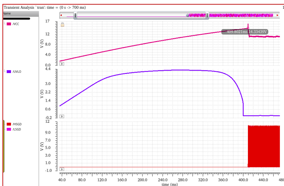
图 5.1 启动阶段仿真波形图
