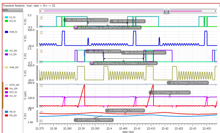
图 4.37 宽输出电压补偿峰值电流控制电路仿真波形图
