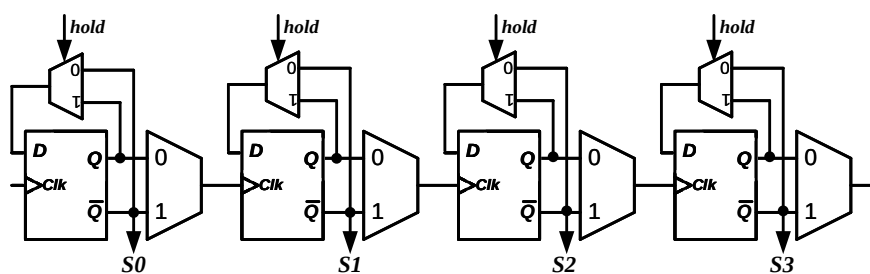
图 4.11 双向计数器原理图
