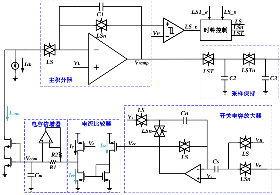
图 4.31 动态校准闭环补偿电路
