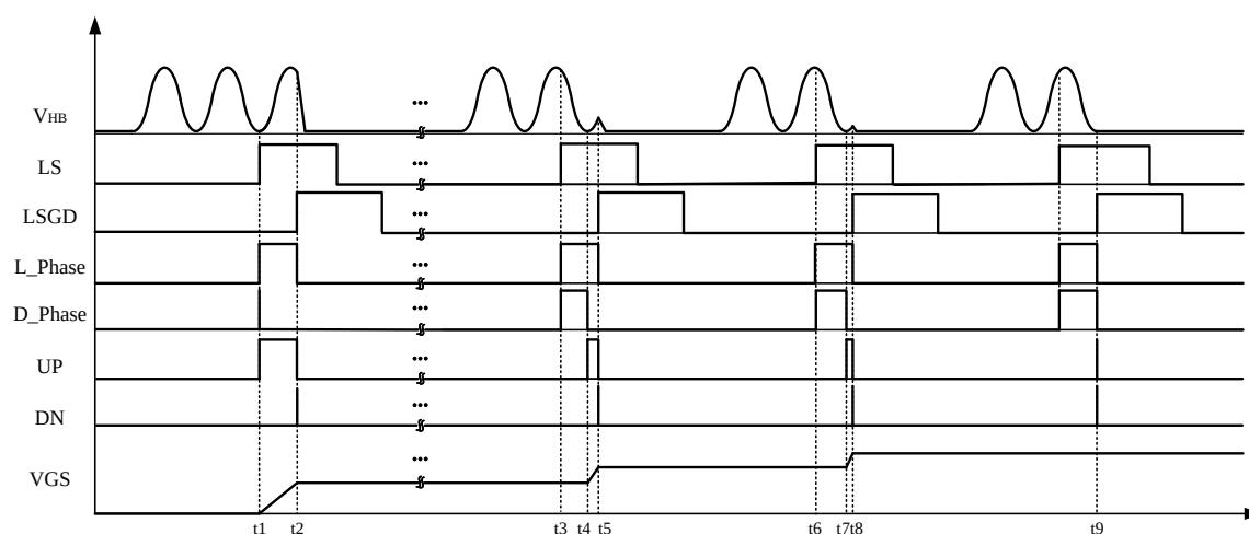
图 4.25 精确谷底导通电路工作波形图
