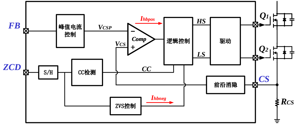
图 3.11 恒流控制模式框图
