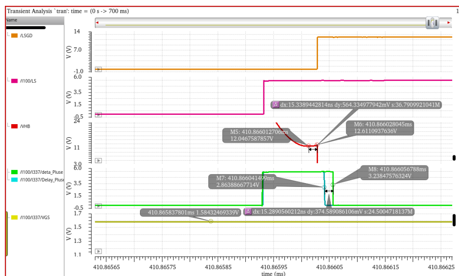
图 5.12 精确谷底导通模块后仿真波形图
