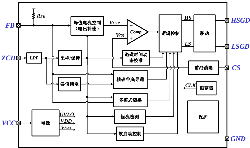
图 3.2 芯片内部结构图
