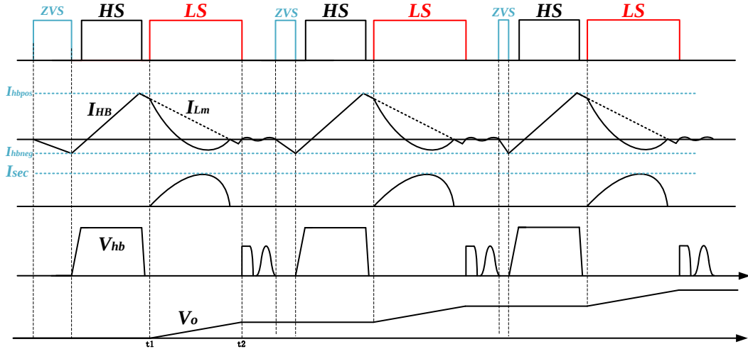
图 3.12 恒流控制模式波形图
