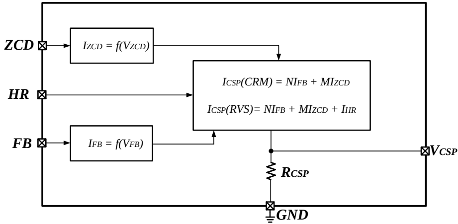
图 4.35 峰值电流控制模块结构框图
