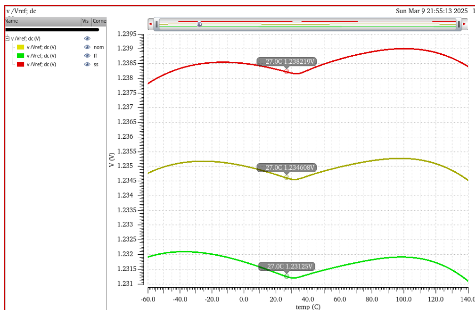
图 4.6 多工艺角带隙基准电路仿真波形图
