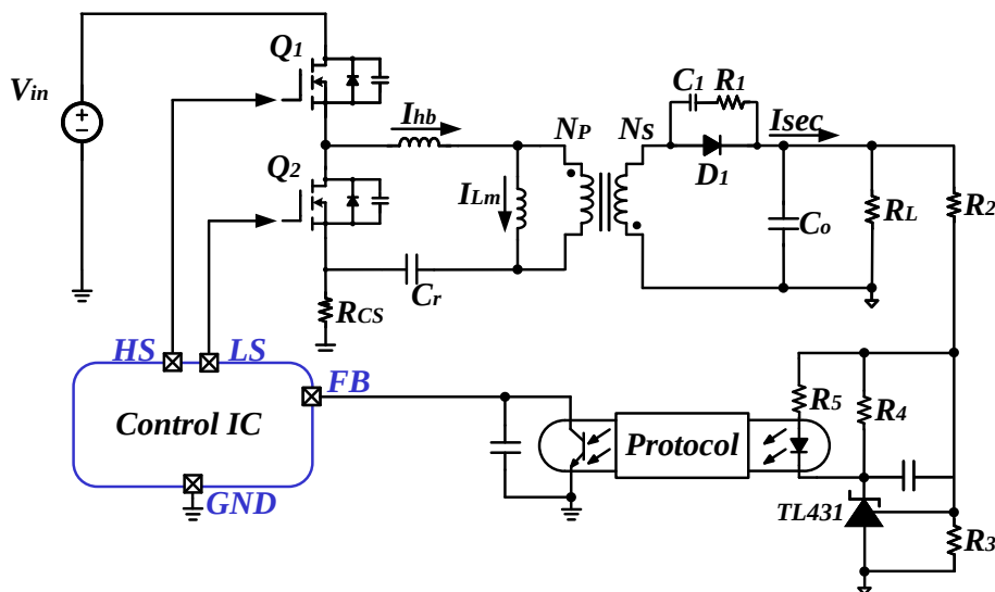
图 2.13 副边反馈电路电路图
