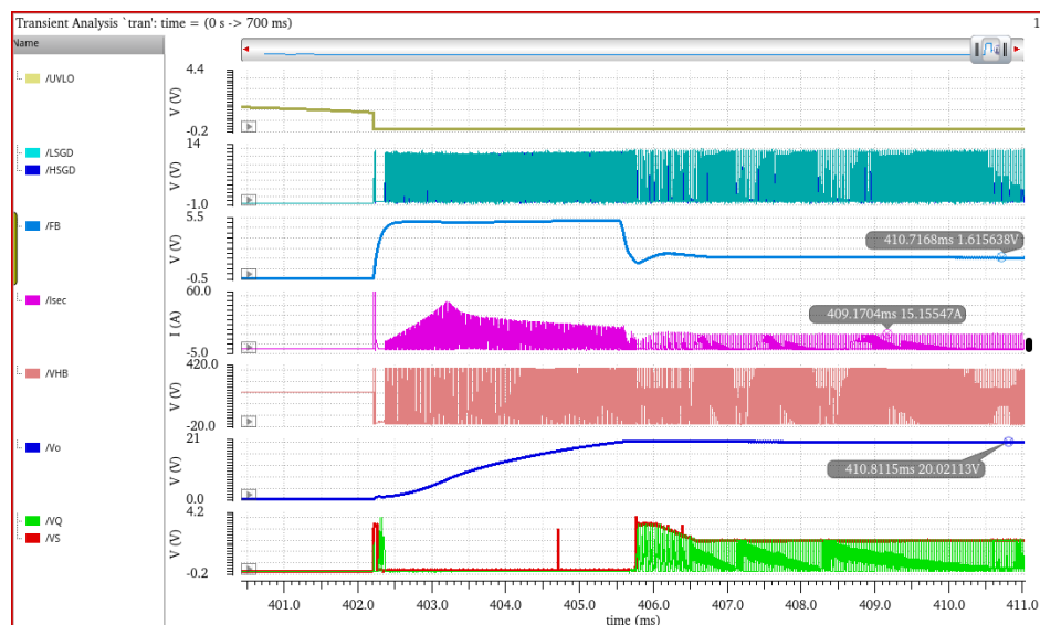
图 5.11 20V/2A 后仿真波形图
