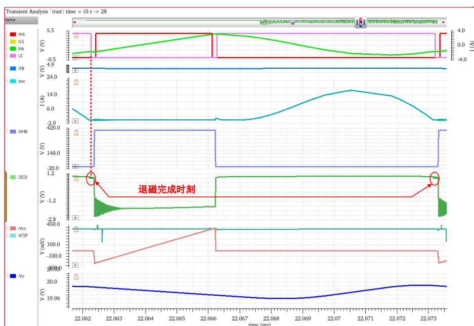
图 5.4 满载电路单周期仿真波形图
