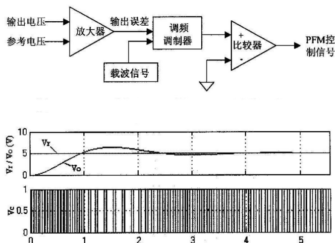
图 2.9 PFM 调制原理图
