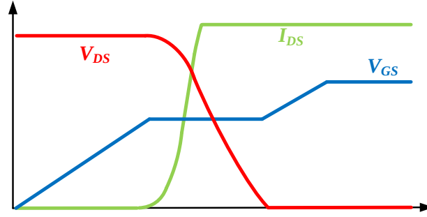
图 3.3 功率管开通损耗波形图
