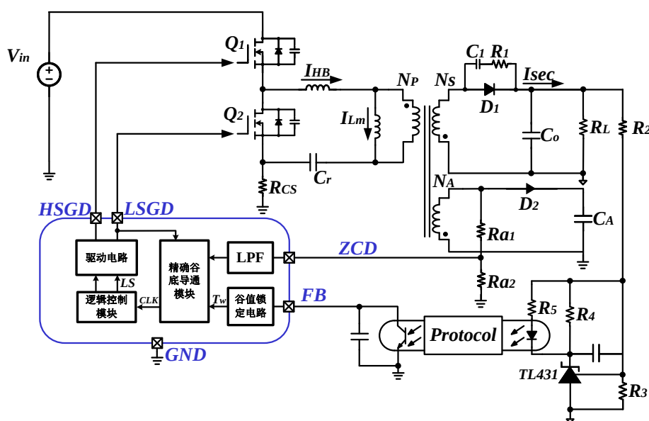
图 3.16 精确谷底导通技术框图
