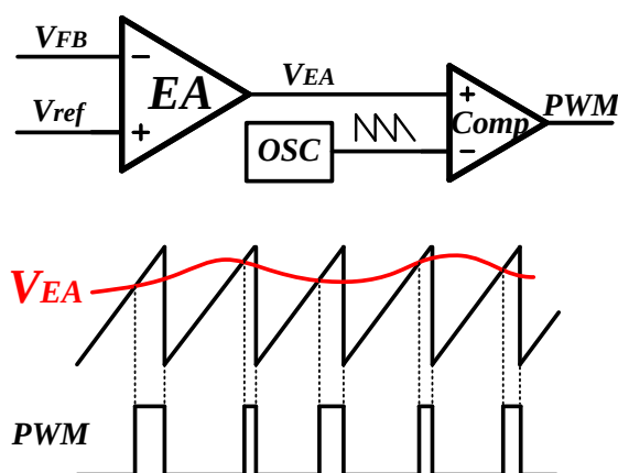
图 2.8 PWM 调制原理图
