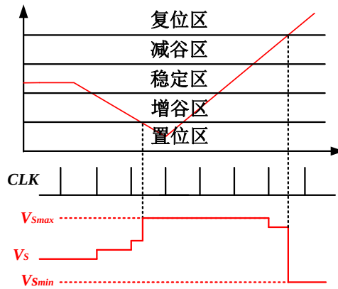
图 3.9 谷值变化策略图
