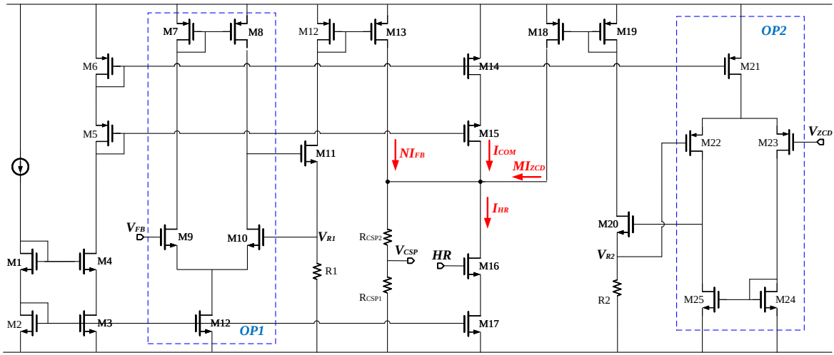
图 4.36 峰值控制电路电路图
