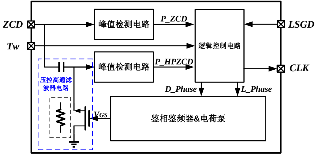
图 4.18 精确谷底导通模块框图
