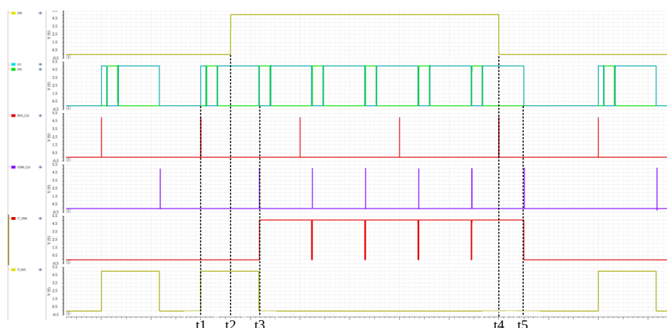
图 4.31 逻辑控制电路具体仿真波形图
