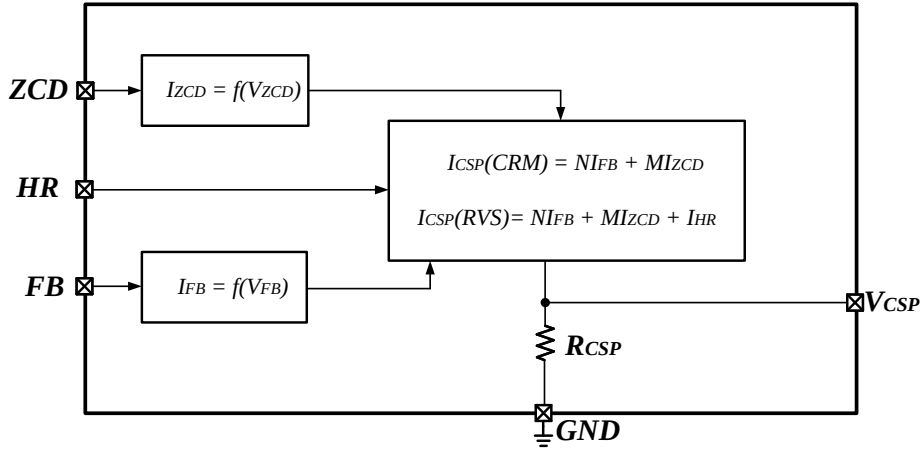
图 4.3 峰值电流控制电路框图
