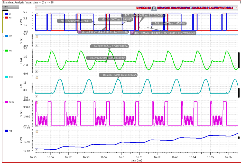
图 4.32 恒流控制模式仿真波形图
