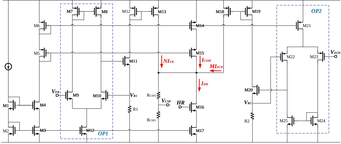
图 4.5 峰值控制电路电路图
