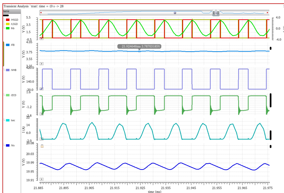
图 4.33 满载电路仿真波形图
