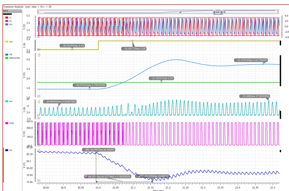
图 4.36 负载 2.5-5A 跳变仿真波形图
