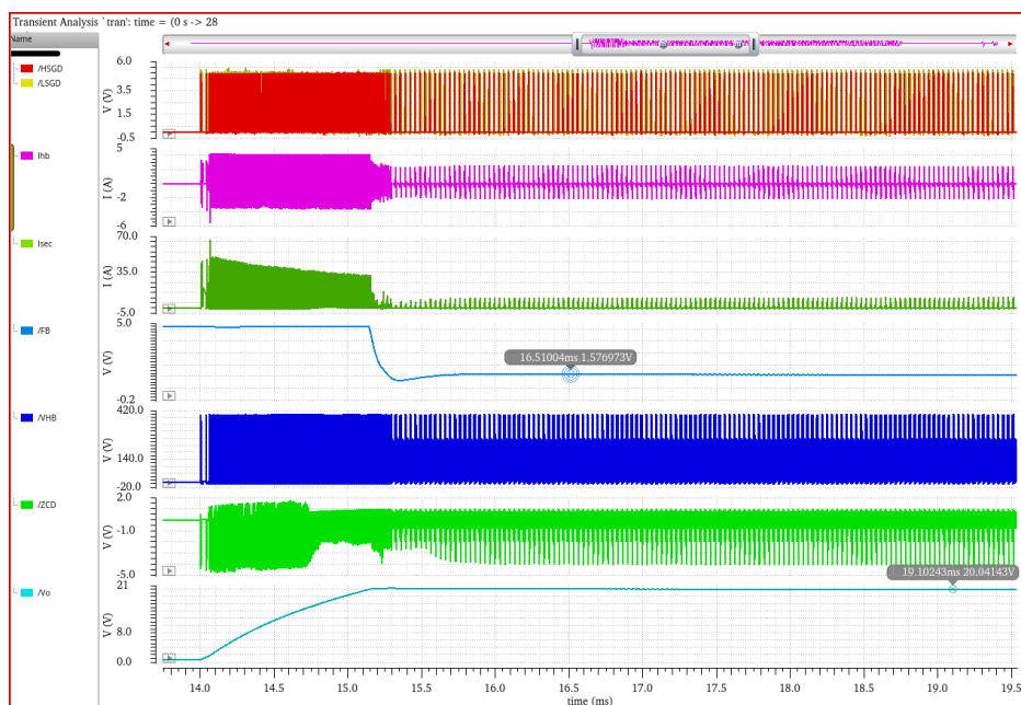
图 4.35 轻载电路仿真波形图
