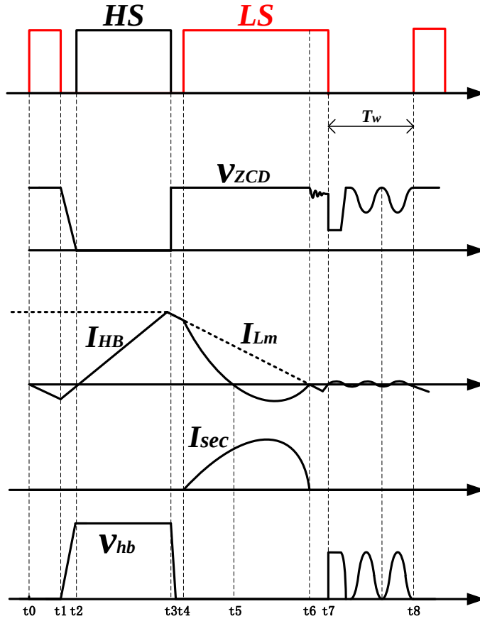
图 3.5 RVS 工作模式波形图
