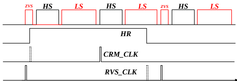
图 4.30 不同工作模式切换波形图
