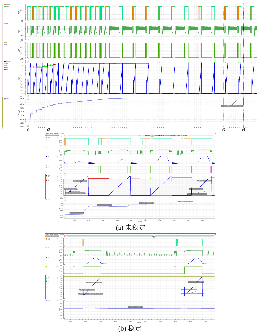
图 4.28 退磁时间动态校准电路波形图
