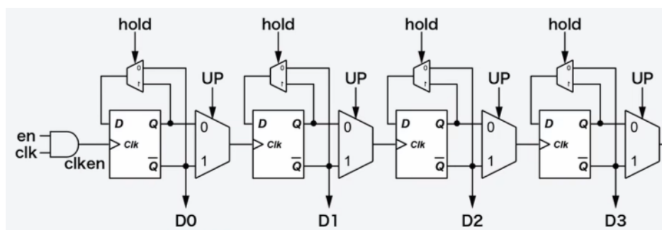
图 4.18 双向计数器电路图
