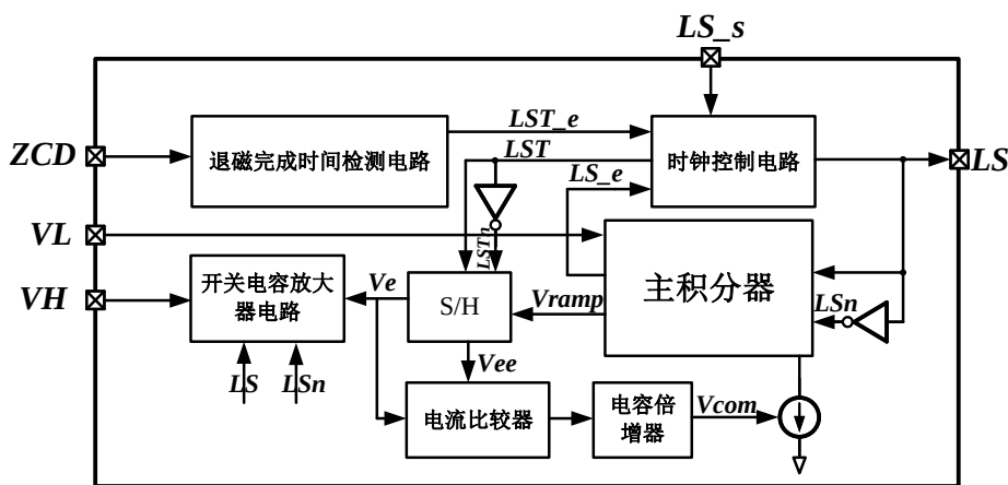
图 4.24 退磁时间动态校准电路框图
