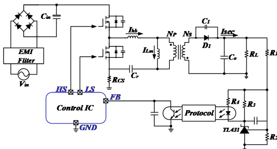
图 2.17 副边反馈电路电路图
