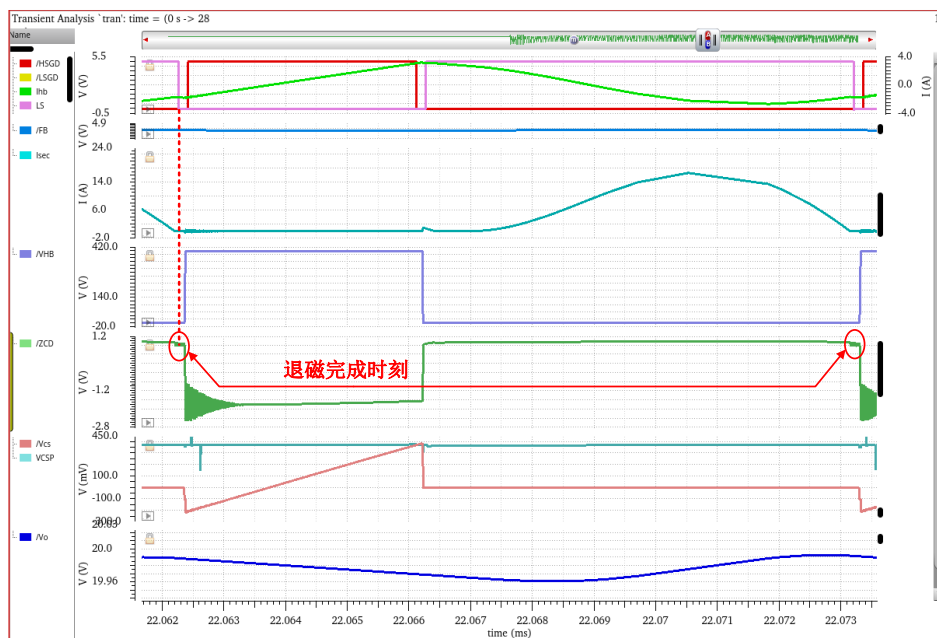
图 4.34 满载电路单周期仿真波形图
