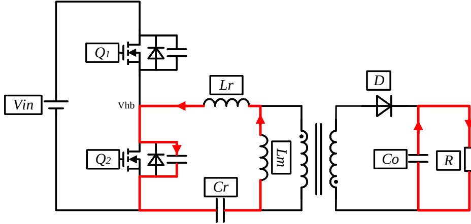
图 2.9 阶段 5 ( t_3 \sim t_4 )
