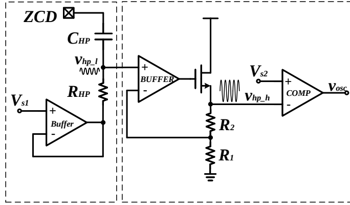
图 4.25 退磁完成时间检测电路
