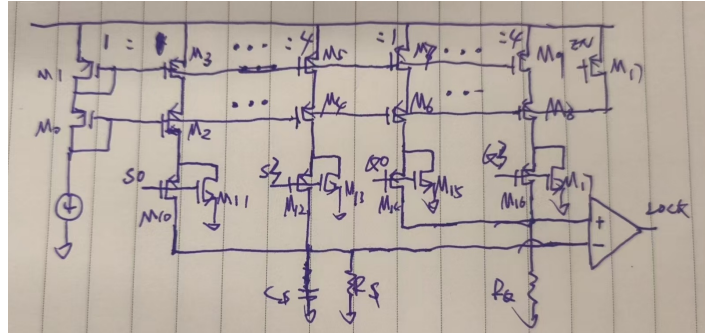
图 4.19 DAC 电路图
