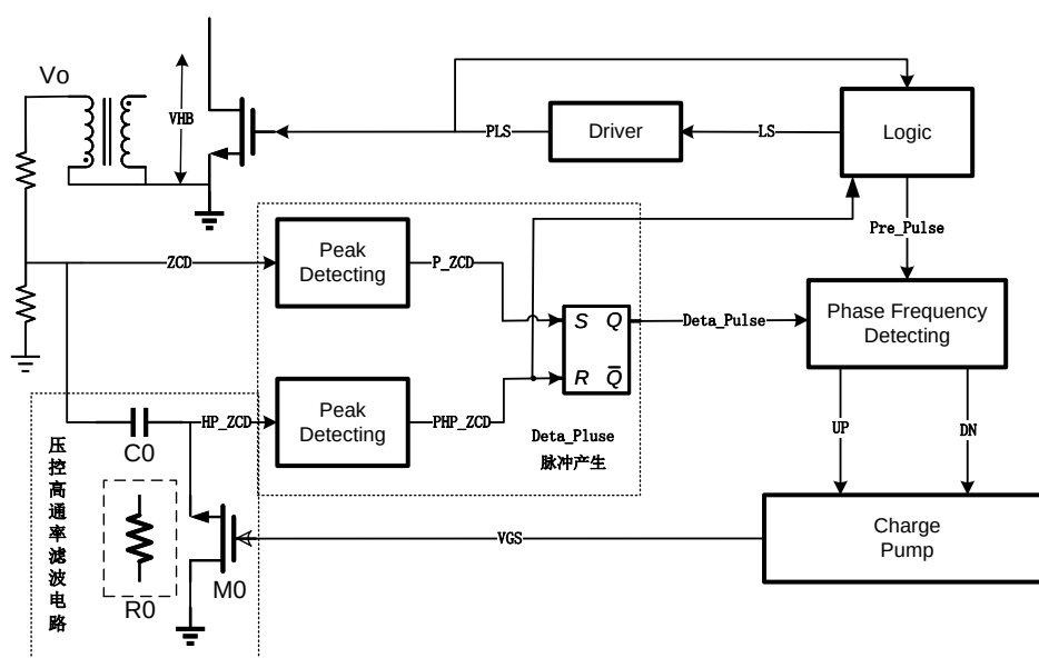
图 4.6 精确谷底导通电路图 1
