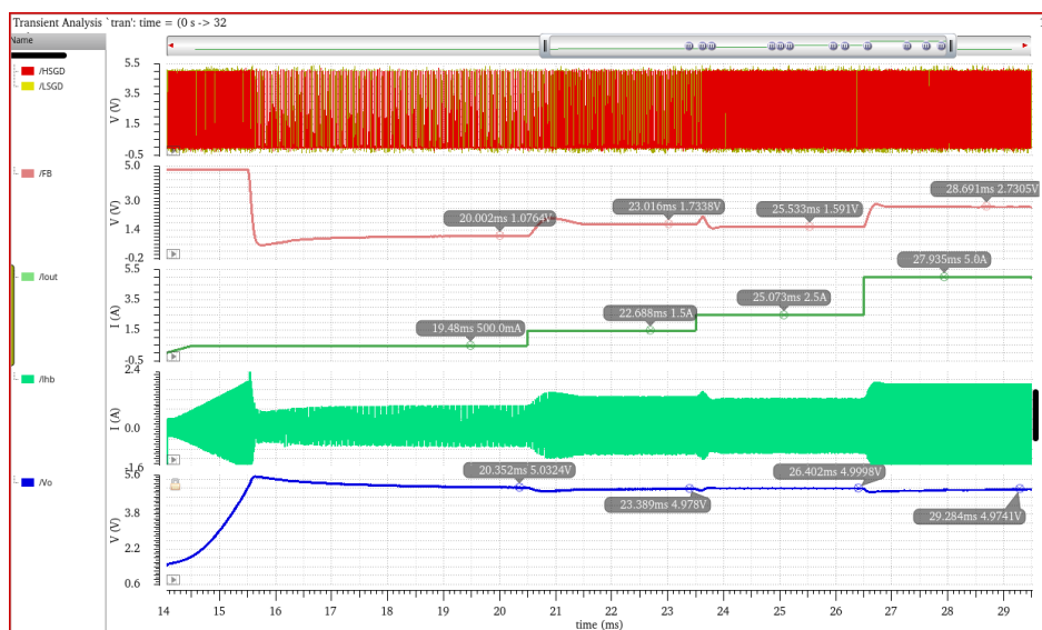
图 4.37 负载调整率仿真波形图
