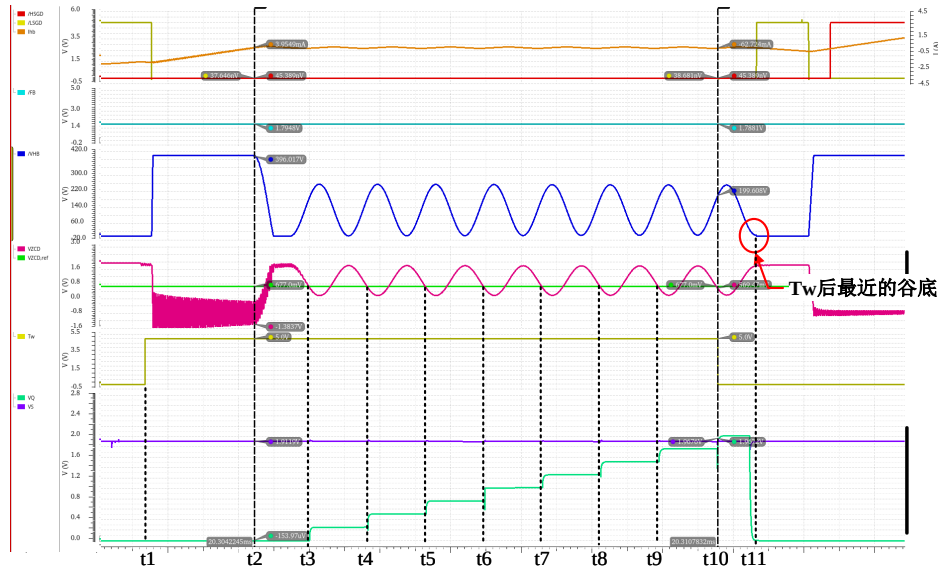
图 4.20 单周期谷值锁定电路波形图
