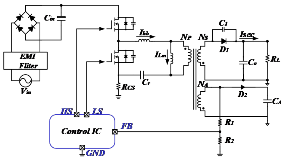
图 2.16 原边反馈电路电路图
