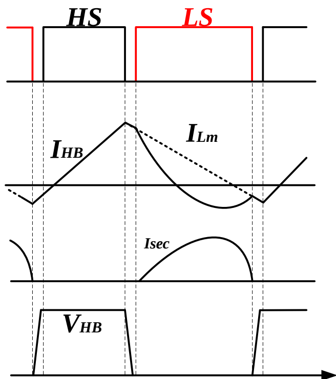
图 2.12 CRM 工作模式波形图
