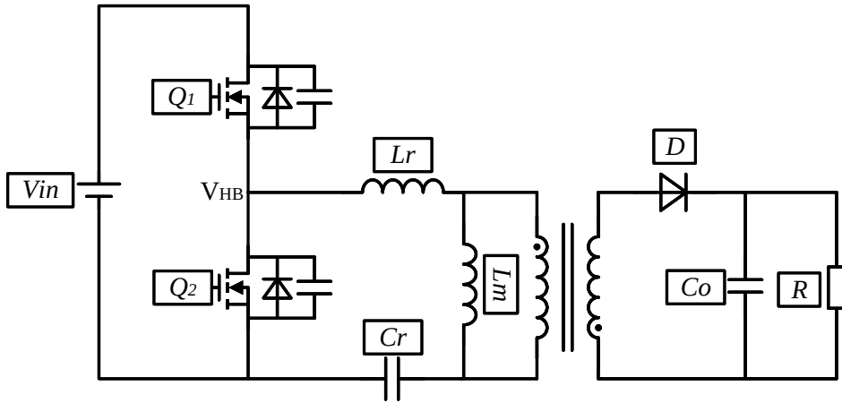
图 2.3 AHB 简化拓扑图
