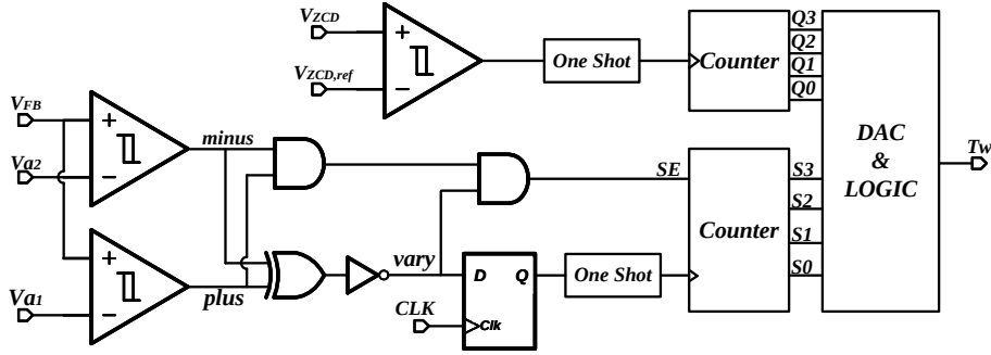
图 4.16 谷值锁定电路 1
