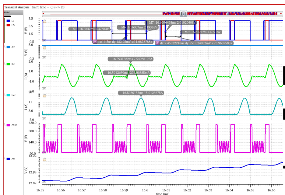
图 4.37 恒流控制模式仿真波形图
