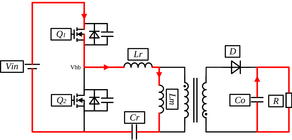
图 2.5 阶段 1 ( t_0 \sim t_1 )
