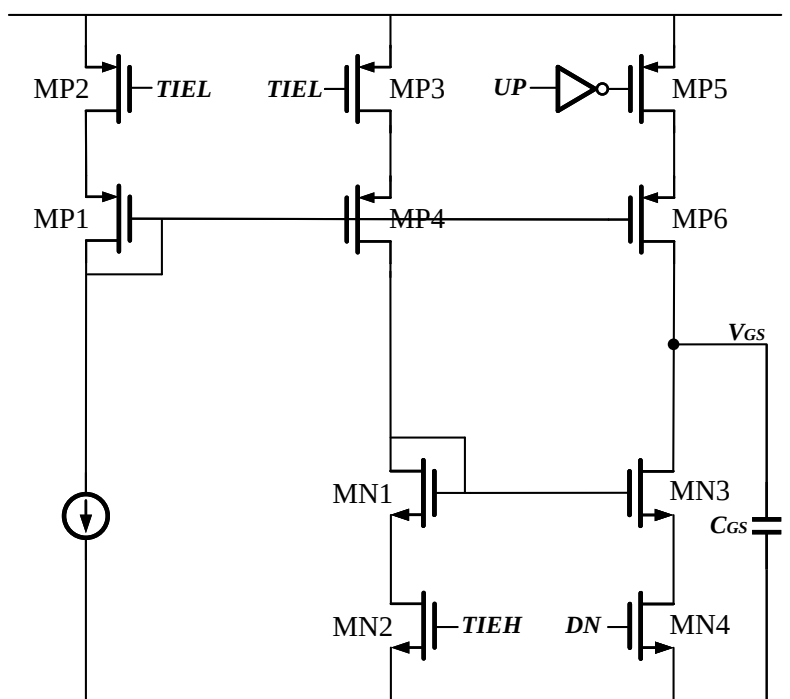
图 4.10 电荷泵电路图
