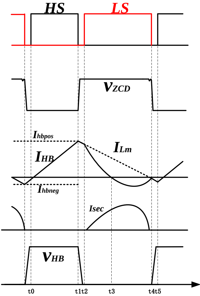
图 2.4 AHBF CRM 工作模式波形图
