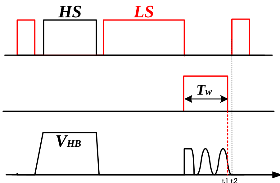
图 4.14 谷值锁定波形 1
