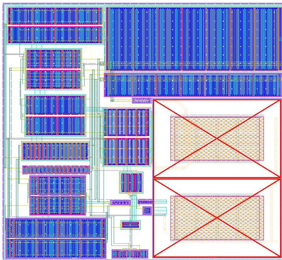
图 5.2 迟滞比较器电路版图
