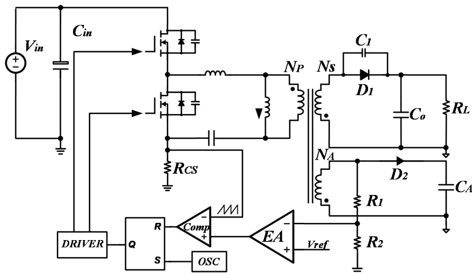
图 2.15 电流工作模式电路图
