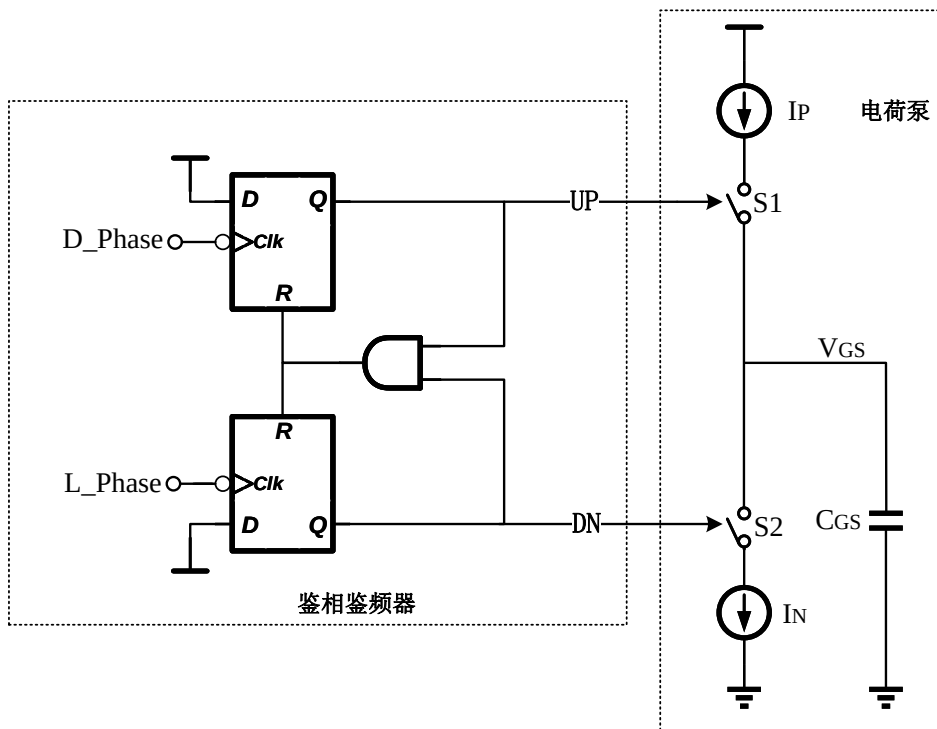
图 4.8 鉴相鉴频器和电荷泵电路图
