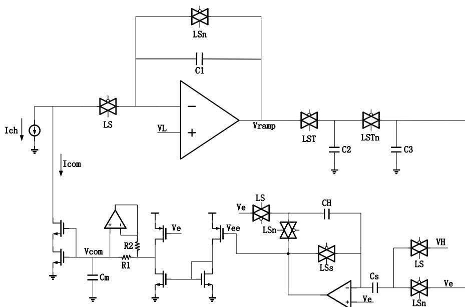
图 4.26 动态校准闭环补偿电路
