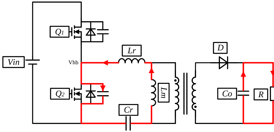
图 2.9 阶段 5 ( t_3 \sim t_4 )
