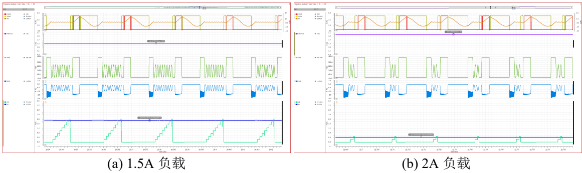
图 4.22 不同负载谷值锁定仿真图
