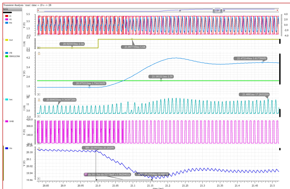
图 4.41 负载 2.5-5A 跳变仿真波形图
