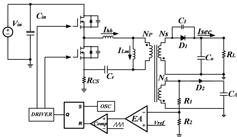
图 2.14 电压工作模式电路图
