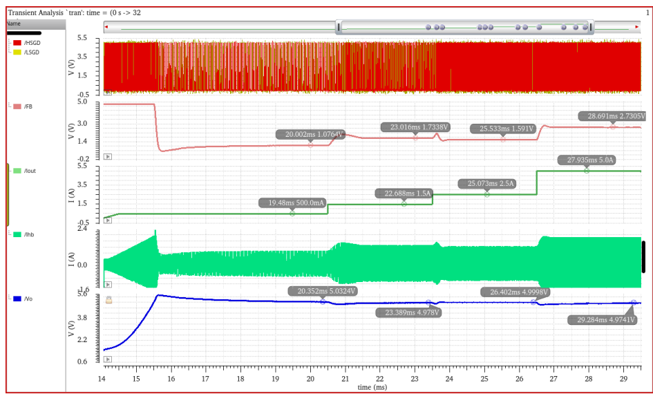
图 4.42 负载调整率仿真波形图
