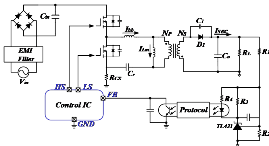
图 2.17 副边反馈电路电路图
