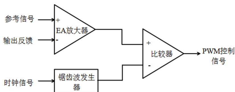
图 2.13 PWM 调制原理图
