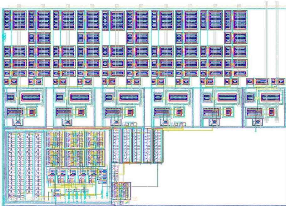
图 5.3 时钟产生电路版图
