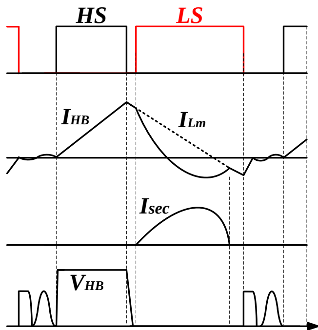
图 2.11 DCM 工作模式波形图
