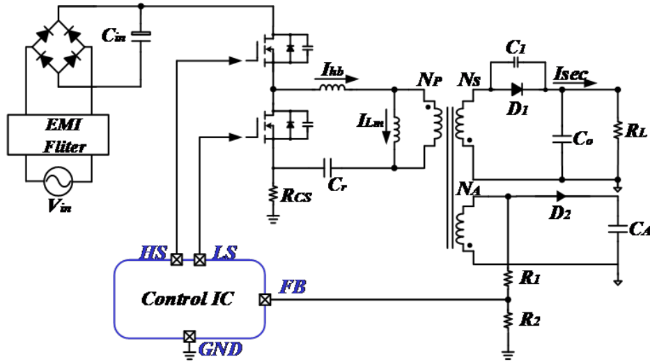
图 2.16 原边反馈电路电路图
