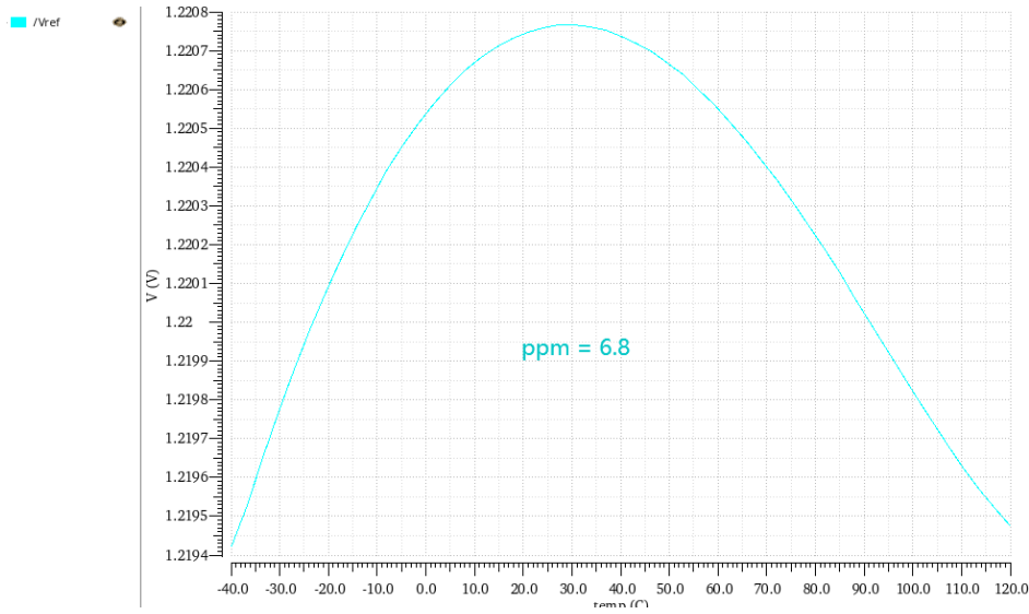
图 4.5 无补偿带隙基准电路仿真波形图
