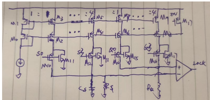
图 4.19 DAC 电路图
