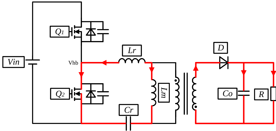
图 2.8 阶段 4 ( t_3 \sim t_4 )
