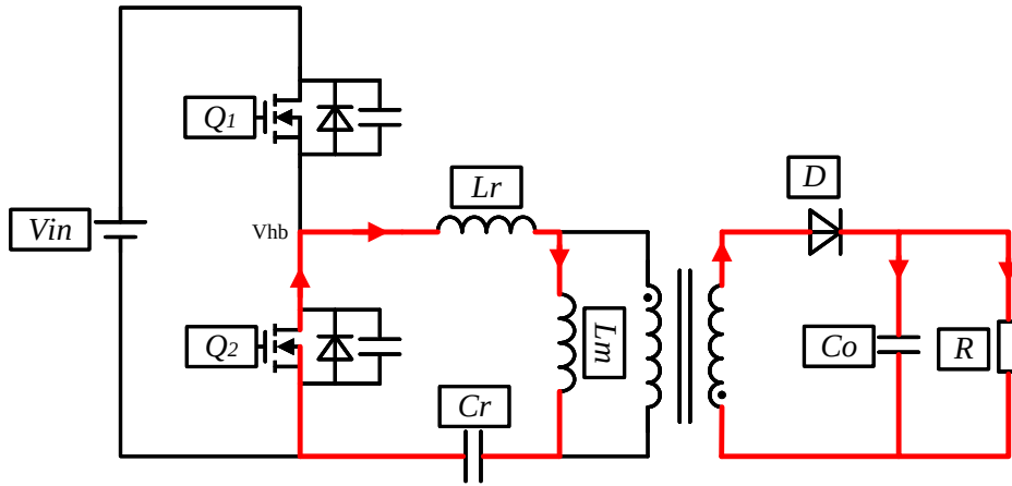
图 2.7 阶段 3 ( t_2 \sim t_3 )
