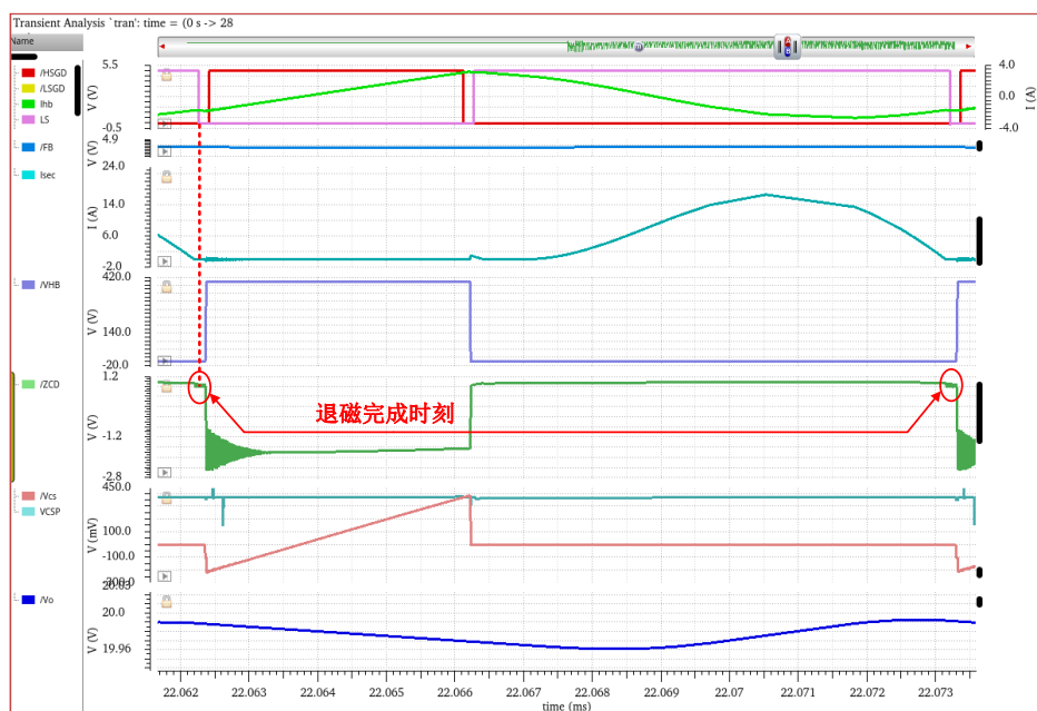
图 4.39 满载电路单周期仿真波形图
