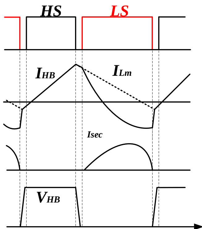
图 2.10 CCM 工作模式波形图
