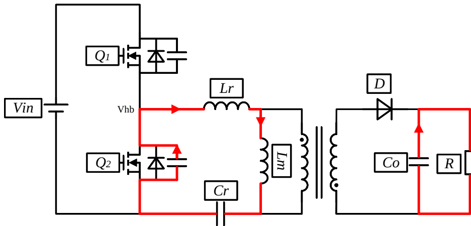
图 2.6 阶段 2 ( t_1 \sim t_2 )
