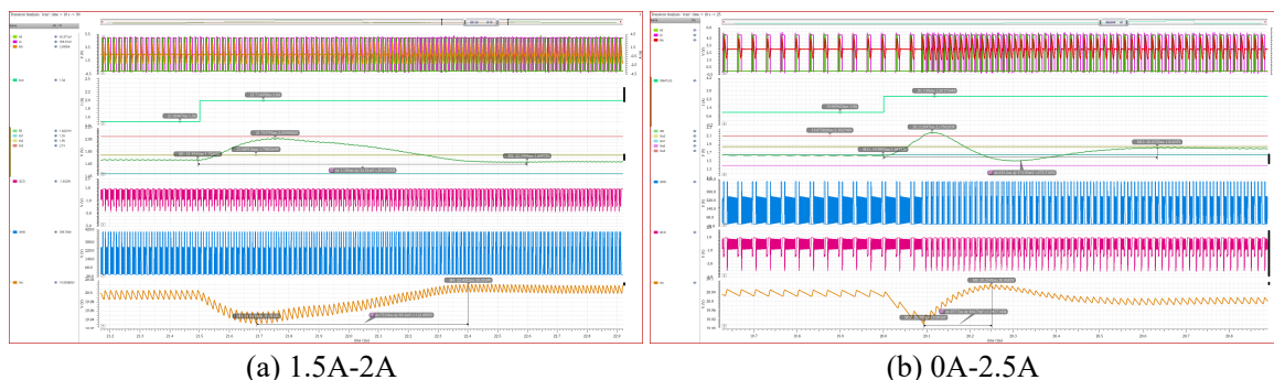
图 4.23 快慢切换的谷值锁定仿真图
