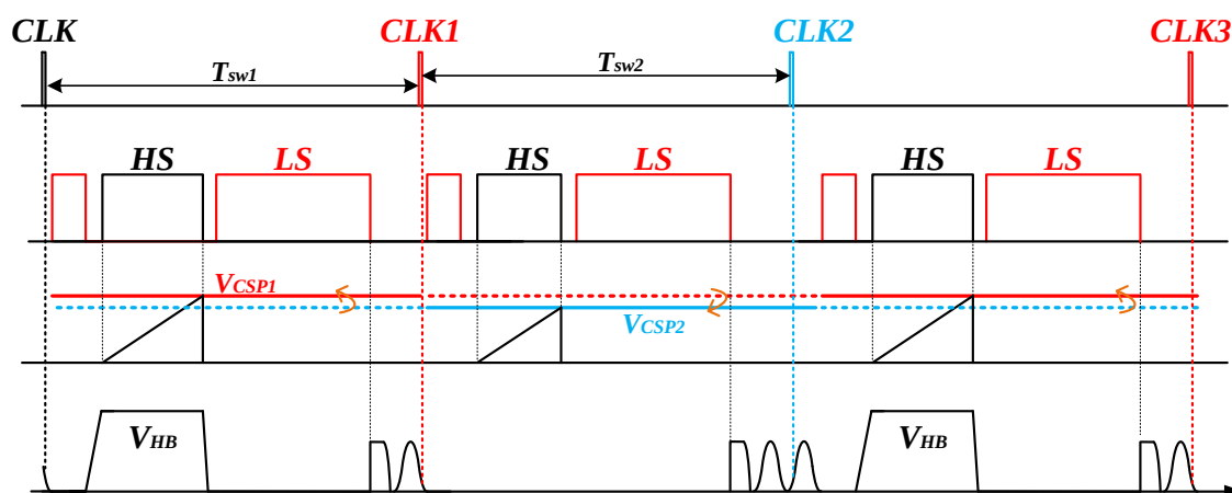
图 4.15 跳谷现象波形图
