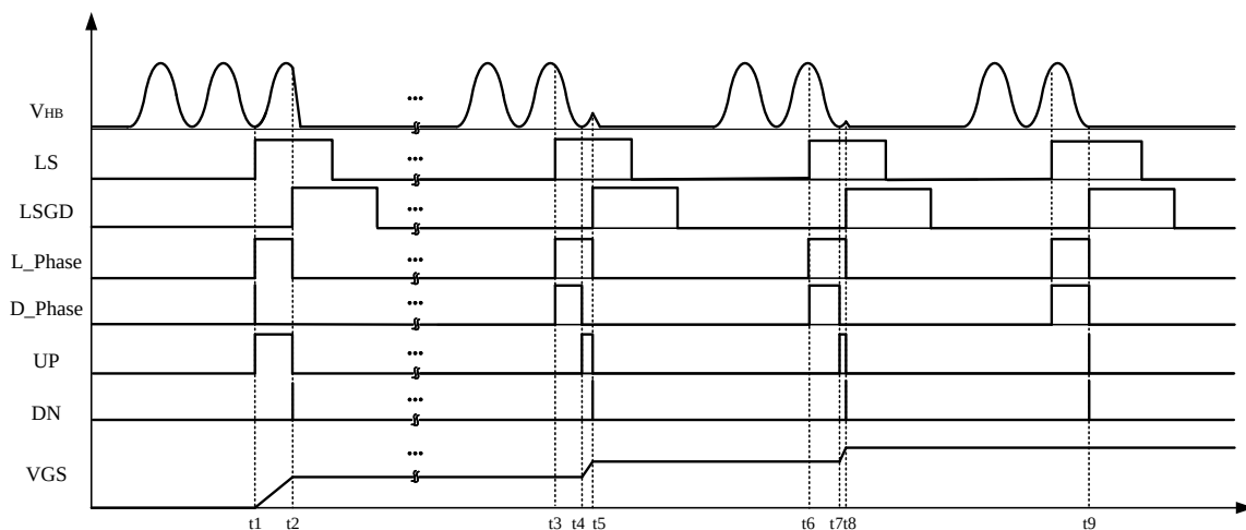
图 4.11 精确谷底导通电路相关波形图
