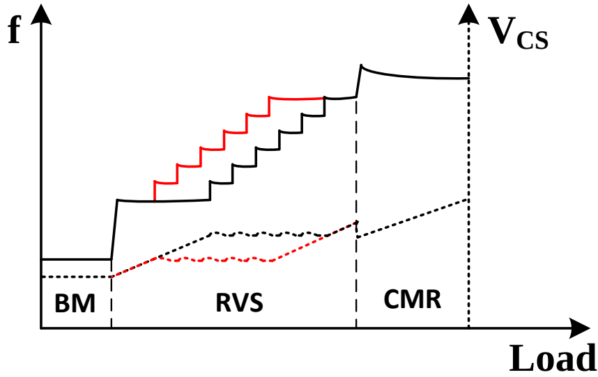
图 3.4 多模式频率变化图
