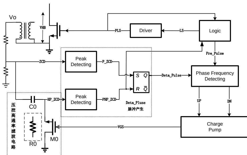
图 4.6 精确谷底导通电路图 1
