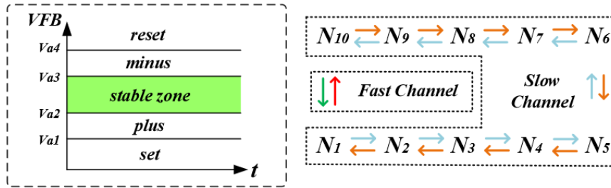
图 4.17 谷值变化策略图
