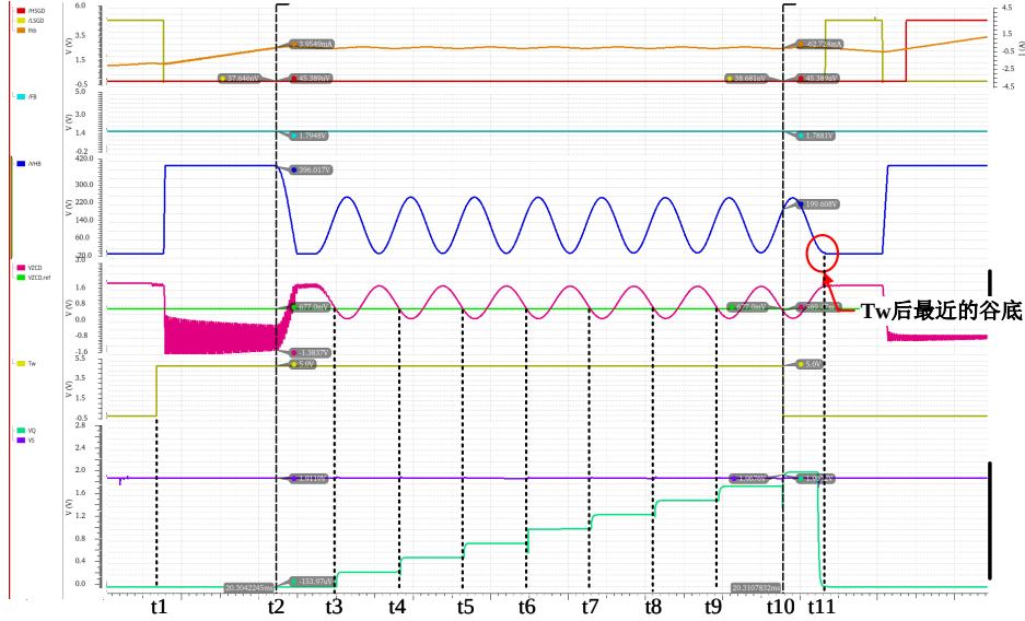
图 4.20 单周期谷值锁定电路波形图
