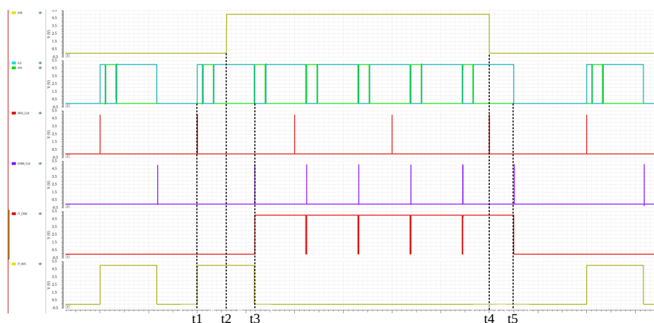
图 4.36 逻辑控制电路具体仿真波形图
