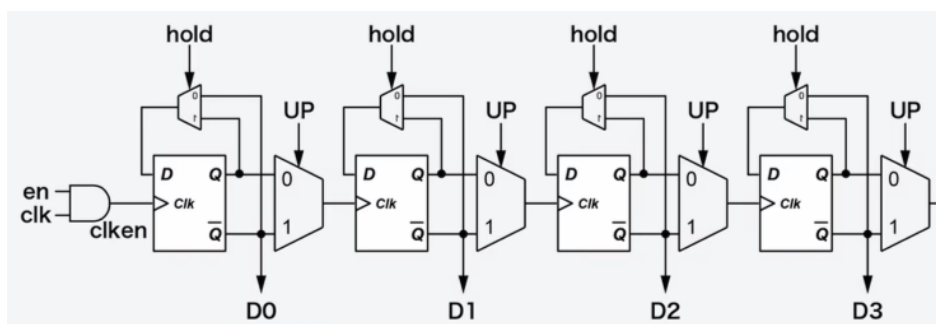
图 4.11 双向计数器电路图
