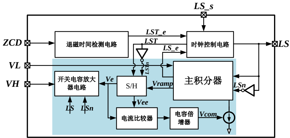
图 4.28 退磁时间动态校准模块框图
