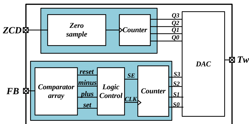
图 3.10 谷值锁定电路框图
