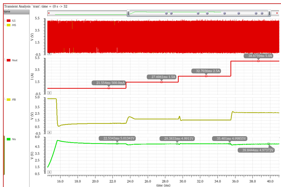
图 5.8 负载调整率仿真波形图
