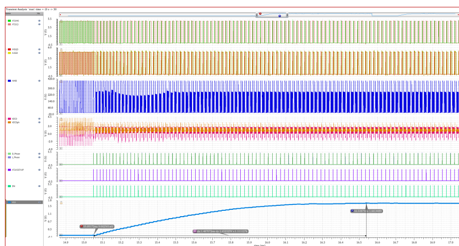
图 4.26 精确谷底导通电路相关波形仿真图
