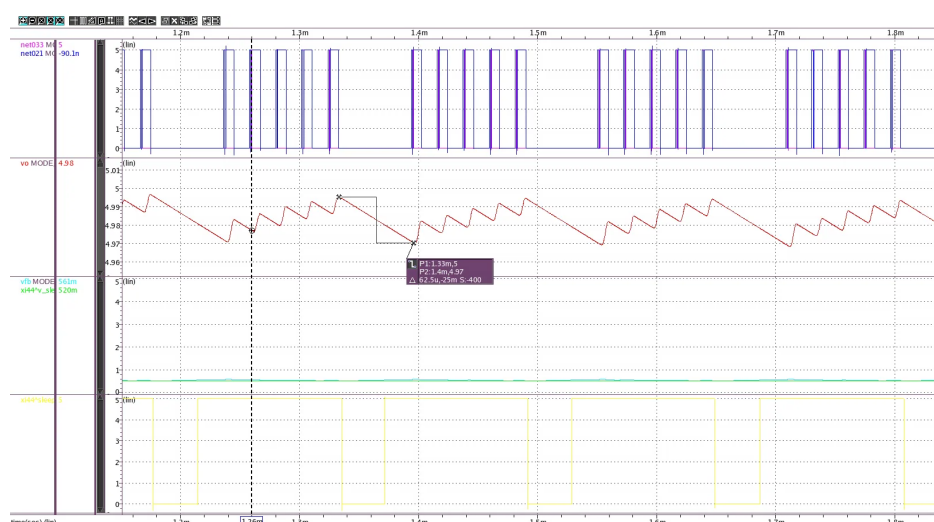
图 5.6 空载电路仿真波形图
