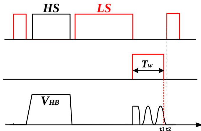
图 3.7 谷值锁定波形 1
