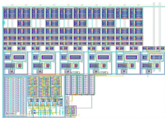
图 5.11 时钟产生电路版图
