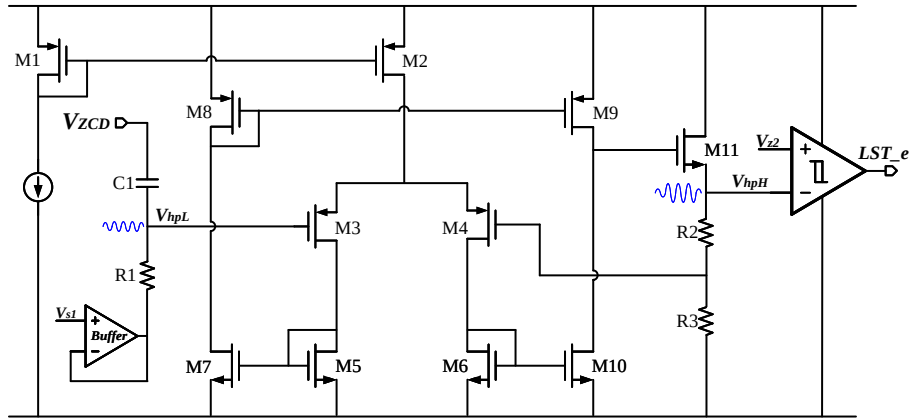
图 4.29 退磁完成时间检测电路
