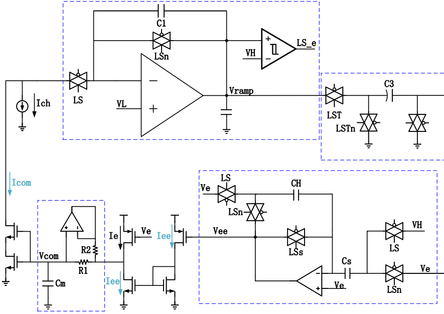
图 4.30 动态校准闭环补偿电路
