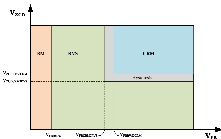
图 3.5 多模式切换图
