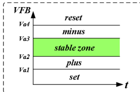
图 3.9 谷值变化策略图
