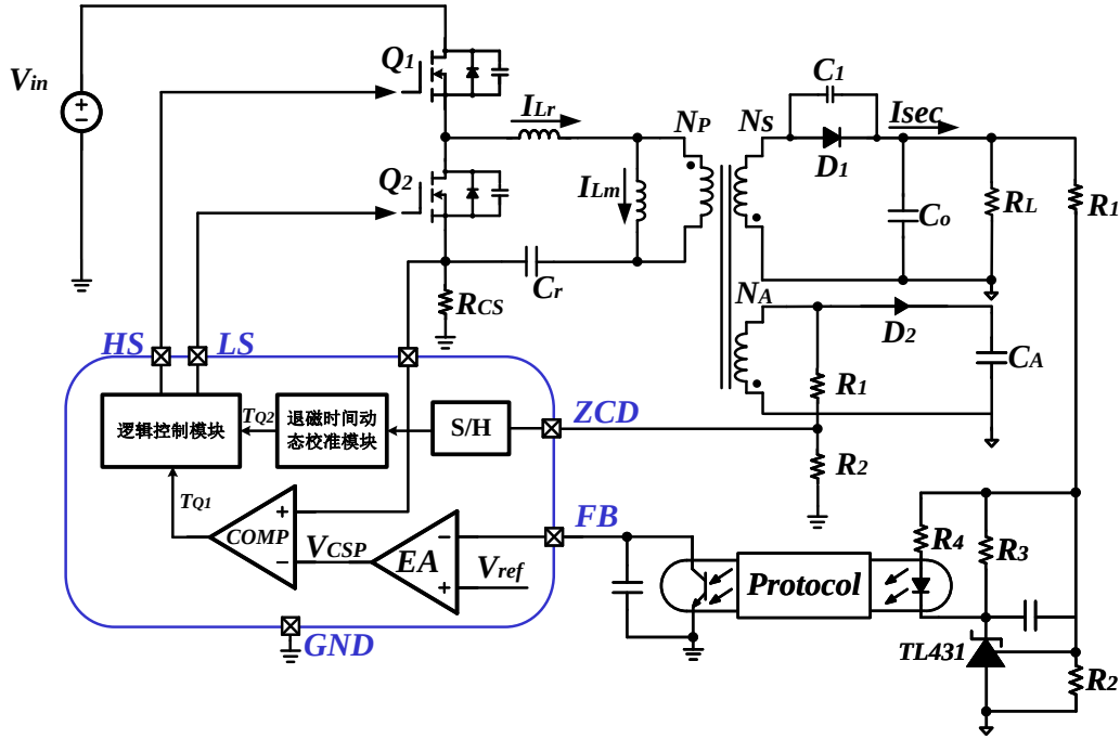
图 3.14 退磁时间动态校准技术框图
