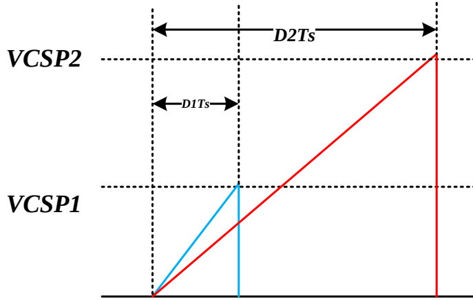
图 4.35 不同输出电压下的峰值电流电压波形
