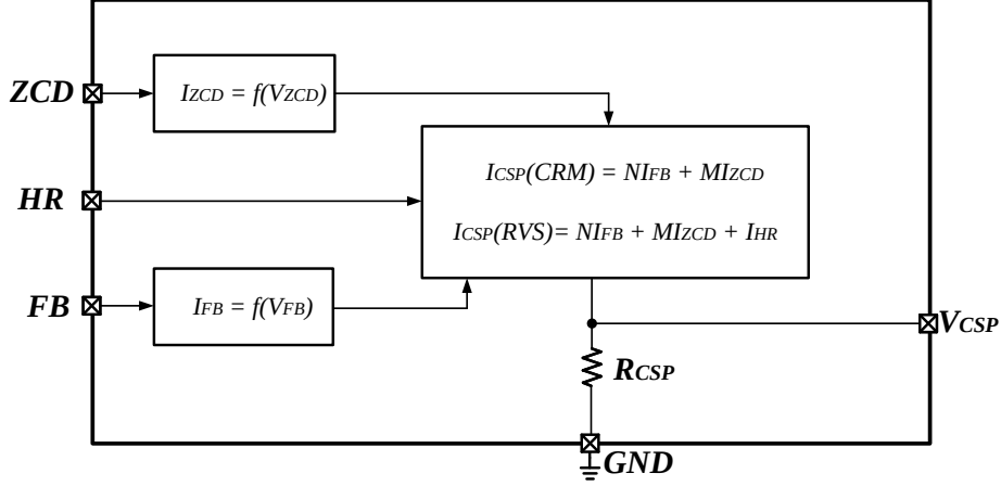
图 4.34 峰值电流控制电路框图
