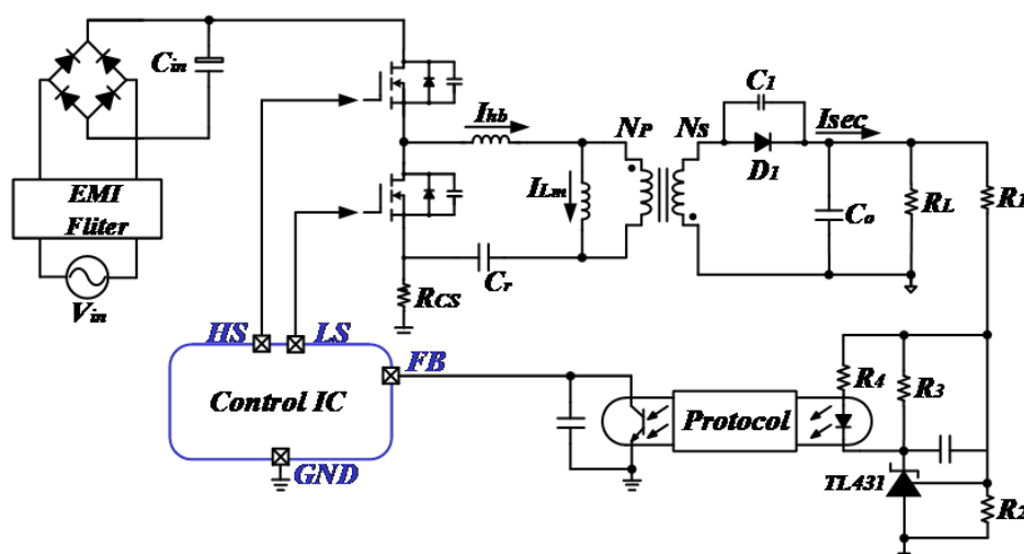
图 2.13 副边反馈电路电路图
