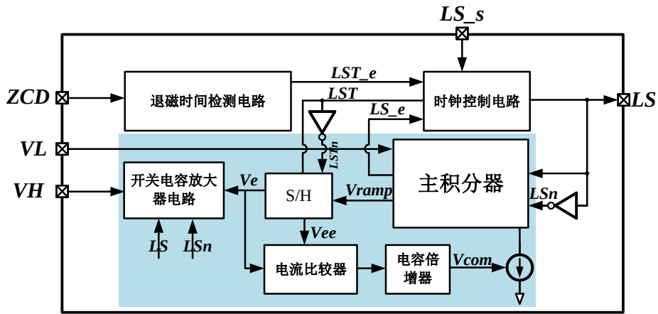
图 4.28 退磁时间动态校准电路框图
