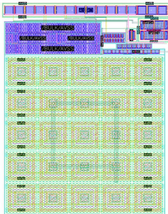
图 5.9 带隙基准电路版图
