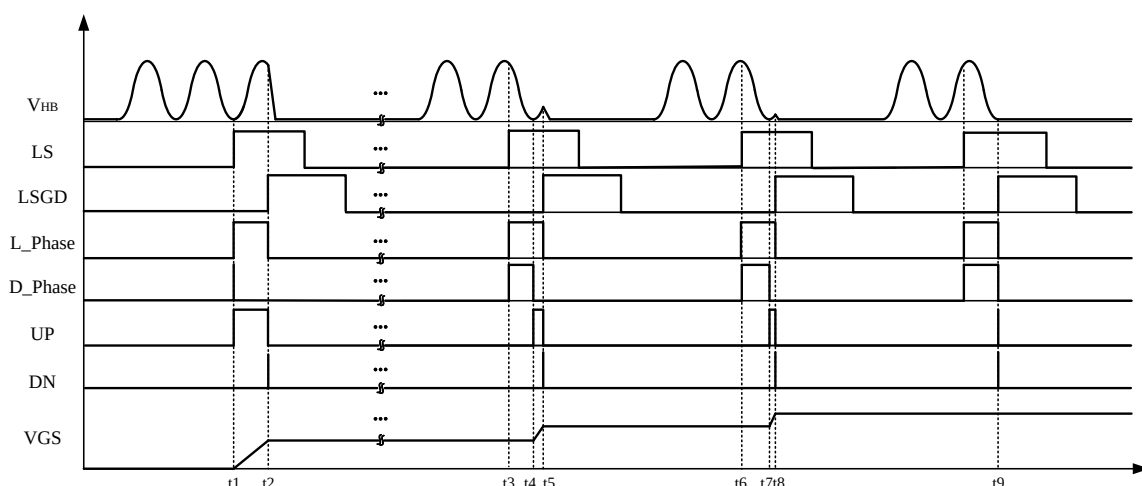
图 4.25 精确谷底导通电路相关波形图
