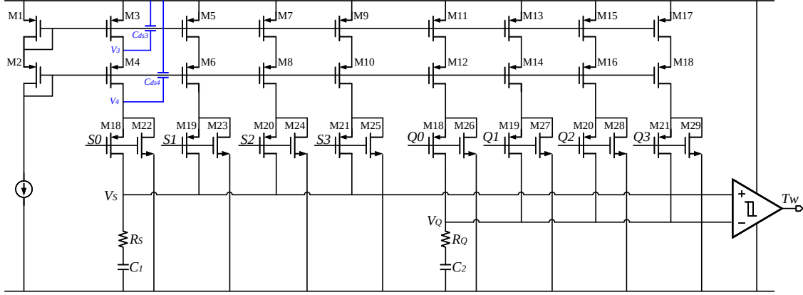
图 4.13 DAC 电路图
