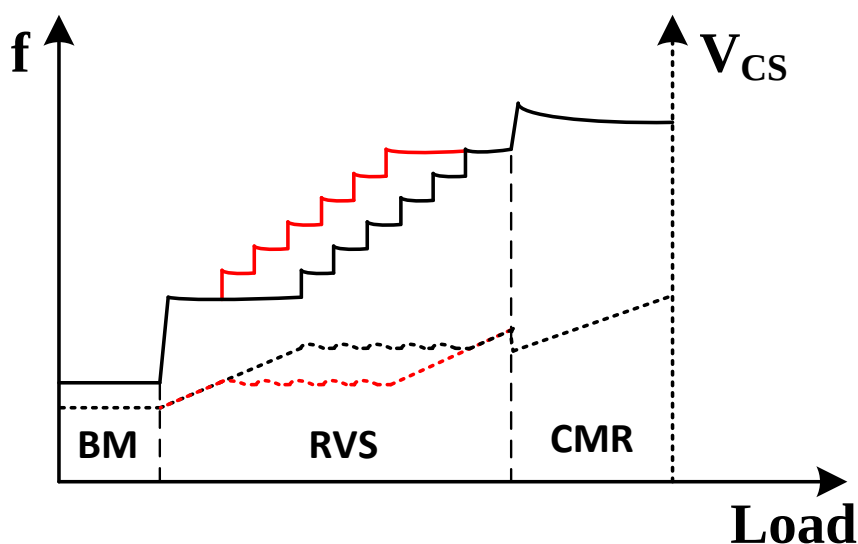
图 3.6 多模式频率变化图
