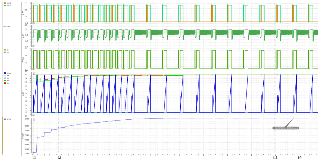
图 4.32 退磁时间动态校准电路仿真波形图
