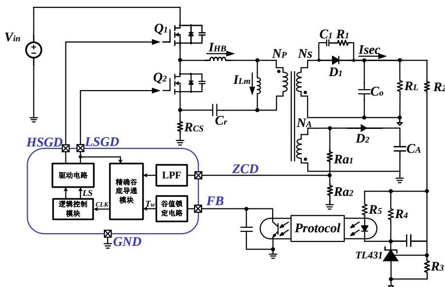
图 3.15 精确谷底导通技术框图
