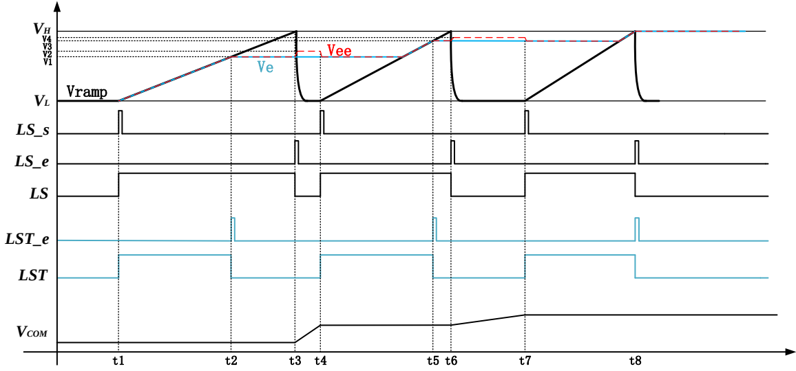
图 4.31 动态校准闭环补偿波形示意图
