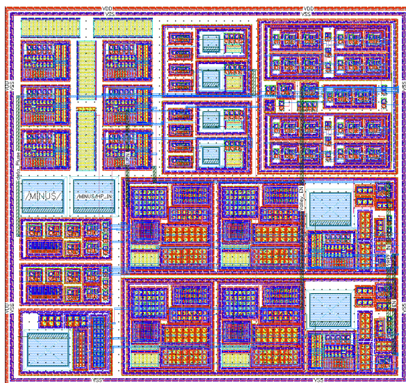
图 5.10 精确谷底导通电路版图
