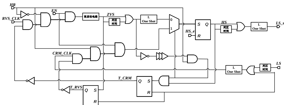
图 4.38 逻辑控制电路原理图
