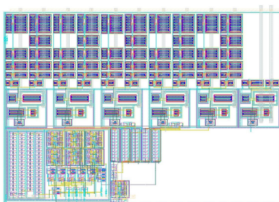
图 5.10 时钟产生电路版图
