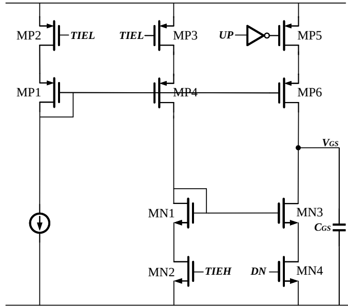
图 4.23 电荷泵电路图
