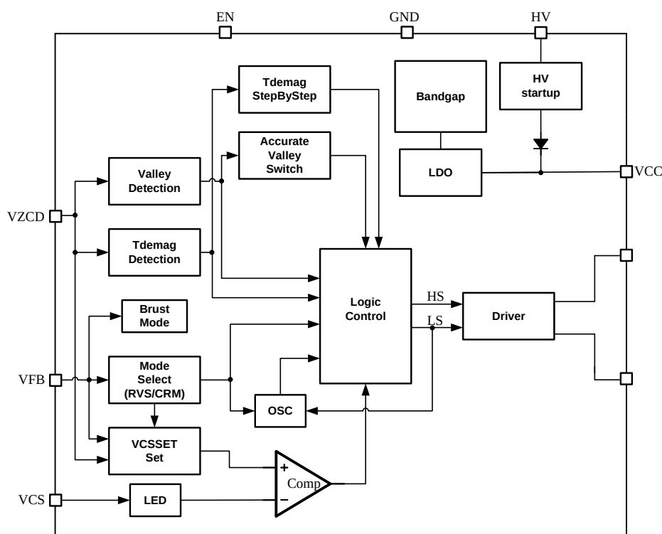
图 3.2 芯片内部结构图
