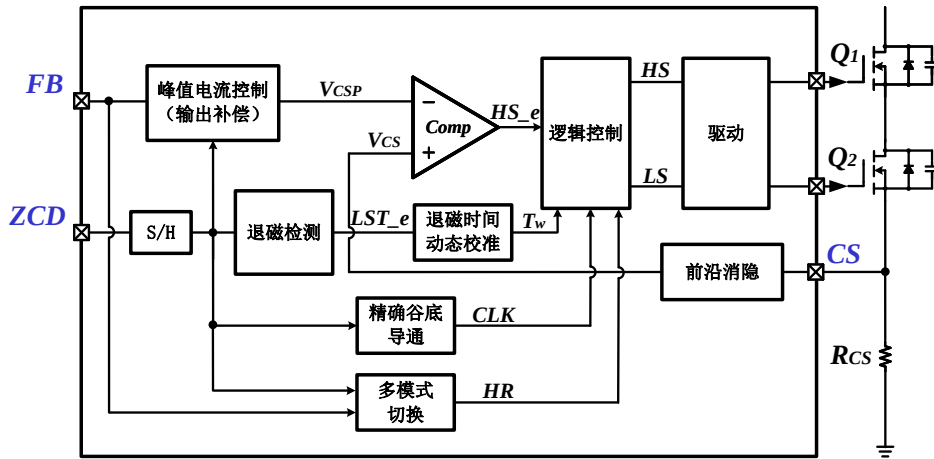
图 3.13 恒压控制模式框图
