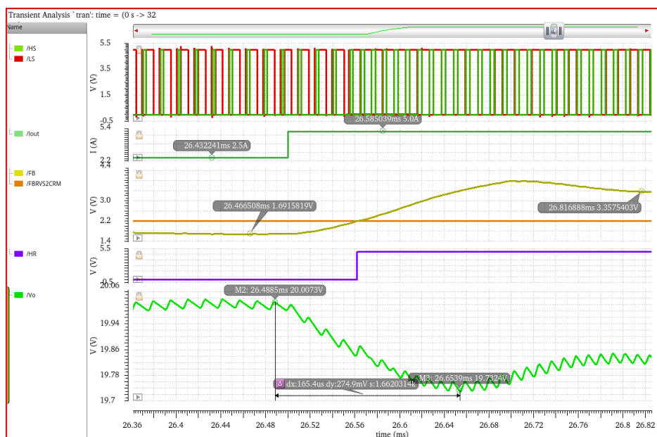
图 5.6 负载 2.5-5A 跳变仿真波形图
