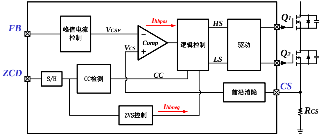
图 3.11 恒流控制模式框图
