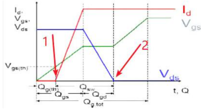
图 3.3 功率管开通损耗波形图
