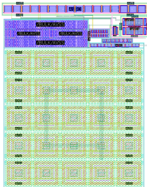
图 5.8 带隙基准电路版图
