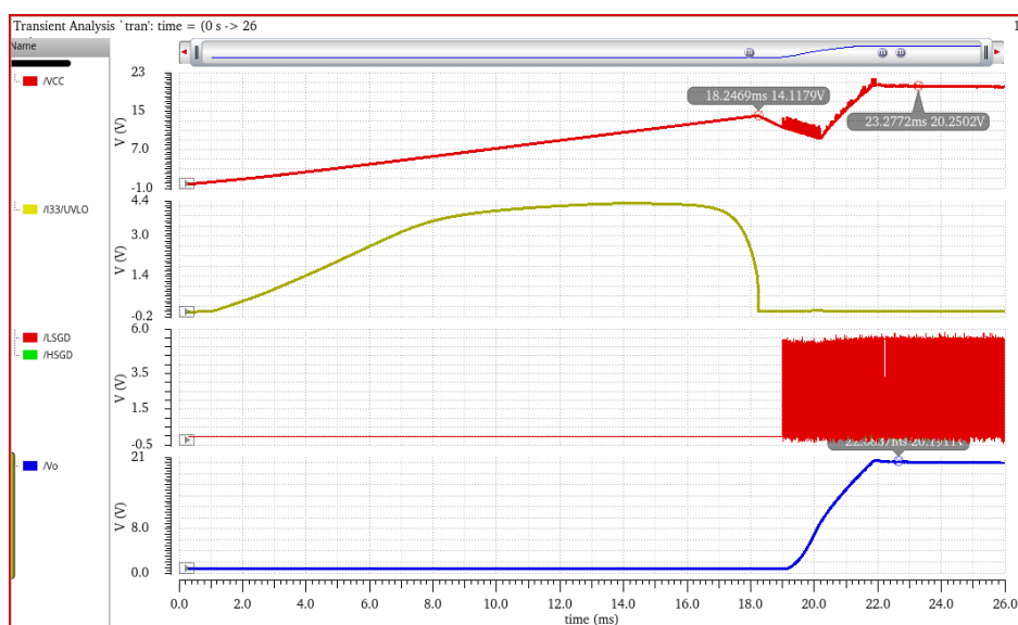
图 5.1 启动阶段仿真波形图
