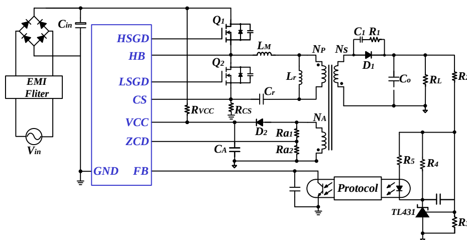
图 3.1 非对称半桥反激式外围拓扑结构图
