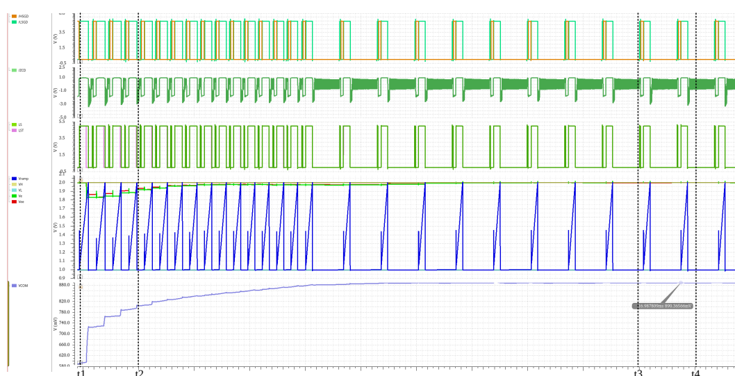
图 4.31 退磁时间动态校准电路 f 仿真波形图
