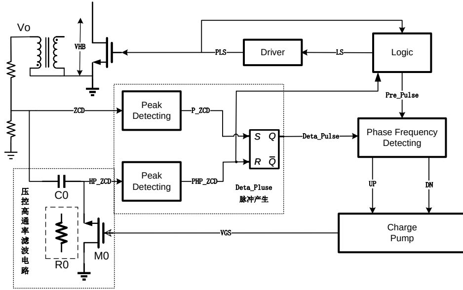
图 4.16 精确谷底导通电路图 1
