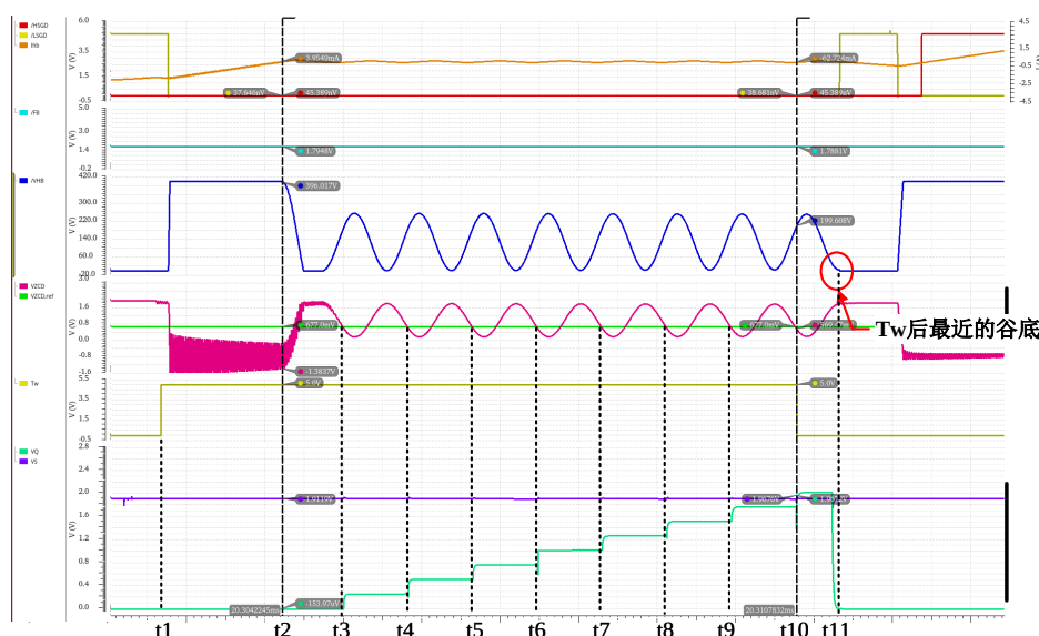
图 4.12 单周期谷值锁定电路波形图
