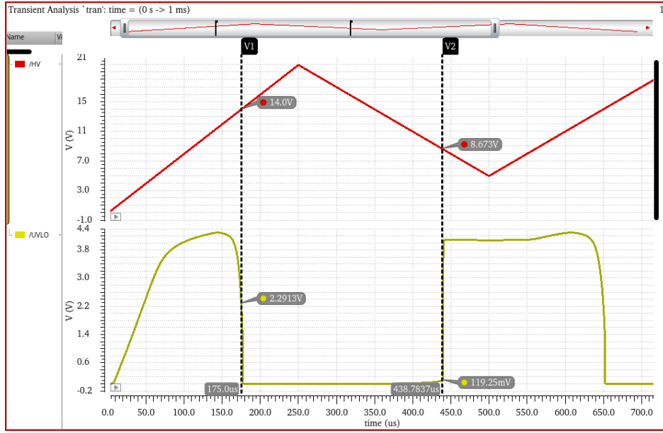
图 4.2 欠压锁定 UVLO 电路仿真图
