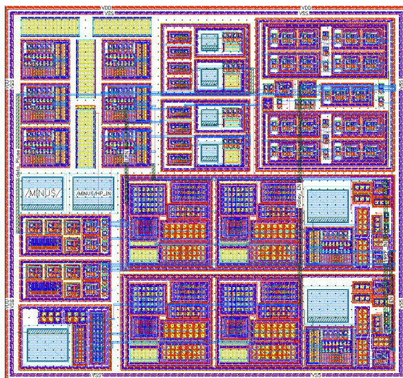
图 5.2 精确谷底导通电路版图
