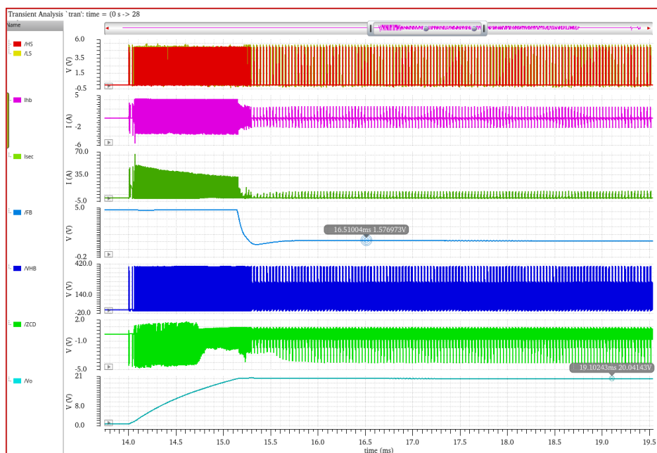
图 4.40 轻载电路仿真波形图
