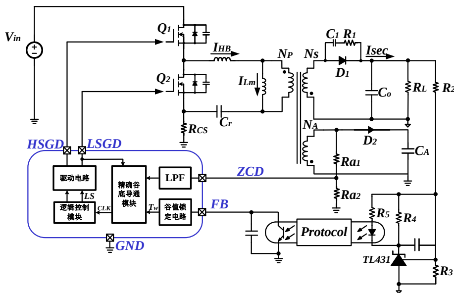
图 3.12 精确谷底导通技术框图
