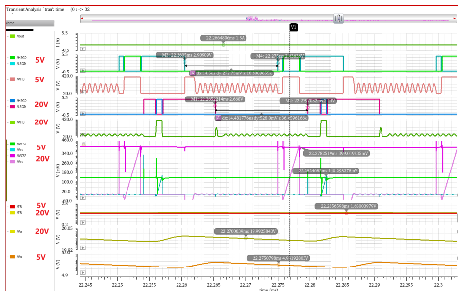
图 4.33 宽输出电压补偿峰值电流控制电路仿真波形图
