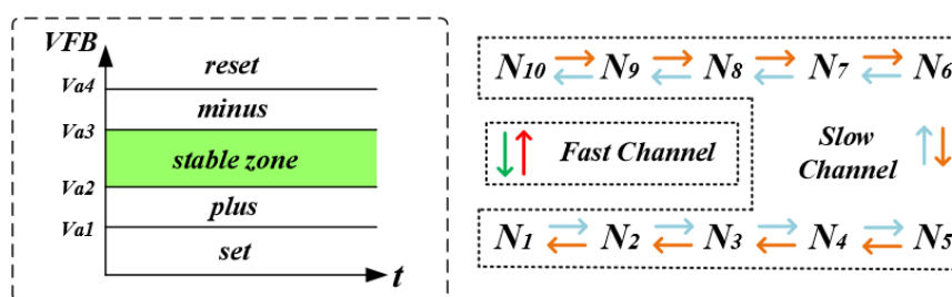
图 4.9 谷值变化策略图
