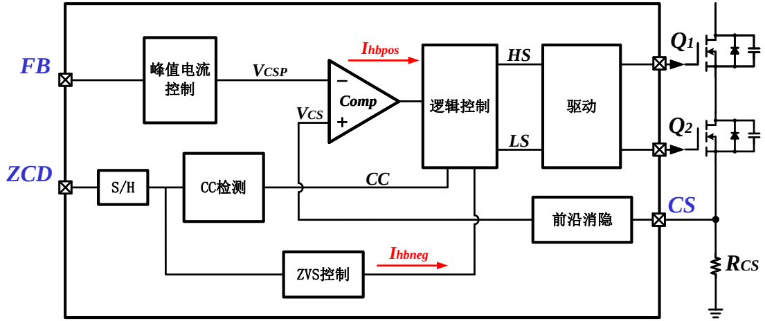
图 3.8 恒流控制模式框图
