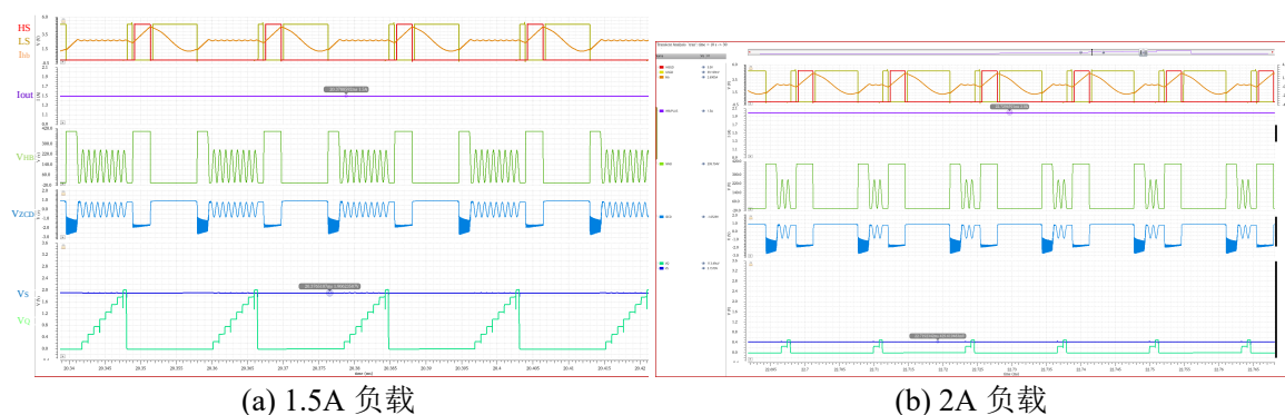
图 4.14 不同负载谷值锁定仿真图
