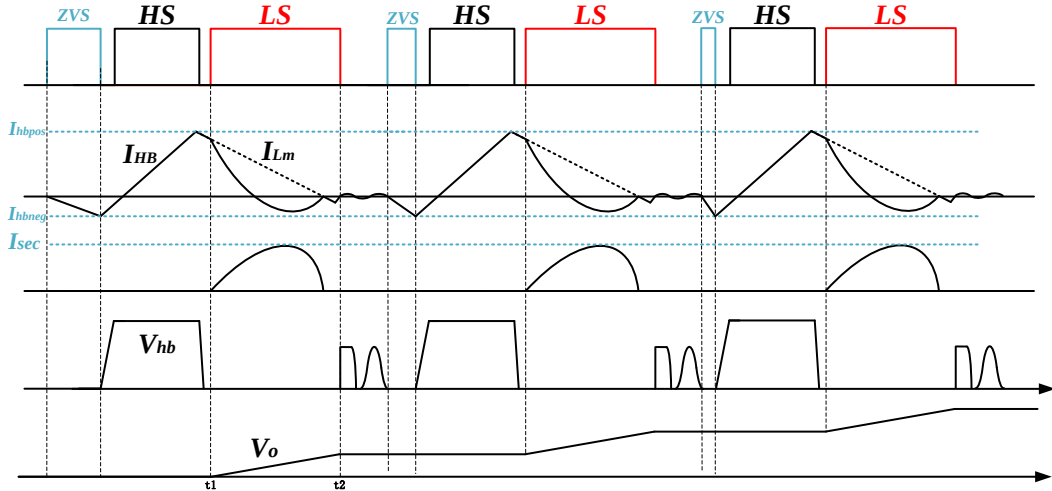
图 3.9 恒流控制模式波形图
