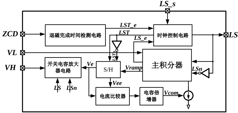
图 4.24 退磁时间动态校准电路框图
