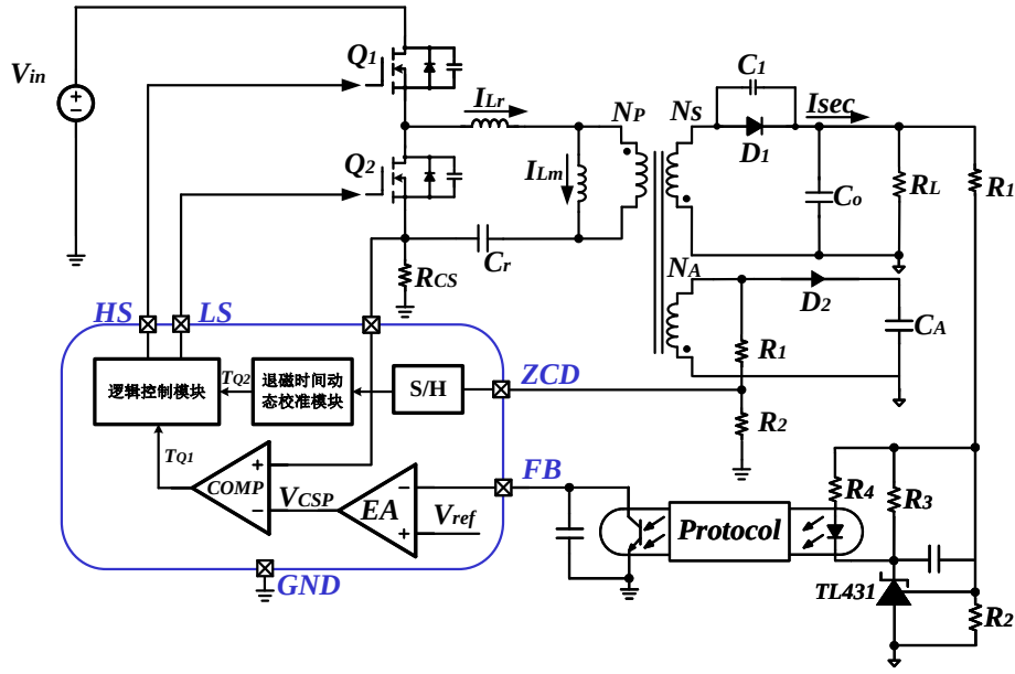
图 3.11 退磁时间动态校准技术框图
