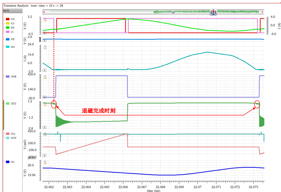
图 4.39 满载电路单周期仿真波形图
