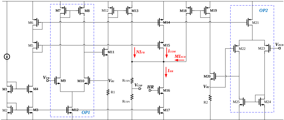
图 4.32 峰值控制电路电路图
