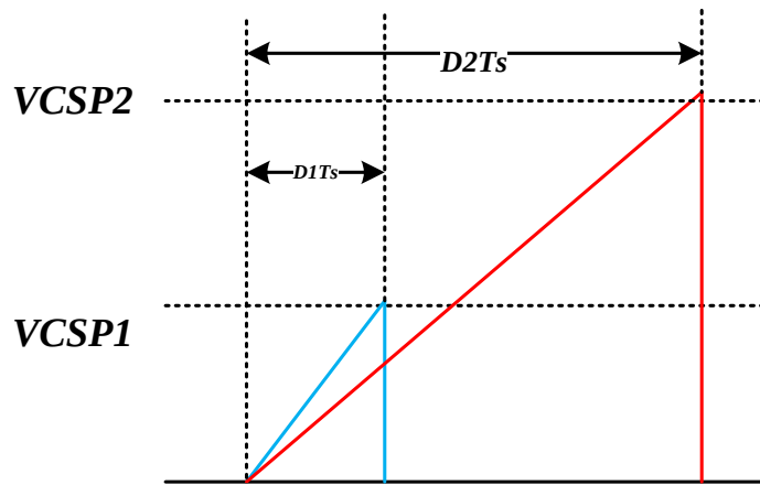
图 4.31 不同输出电压下的峰值电流电压波形
