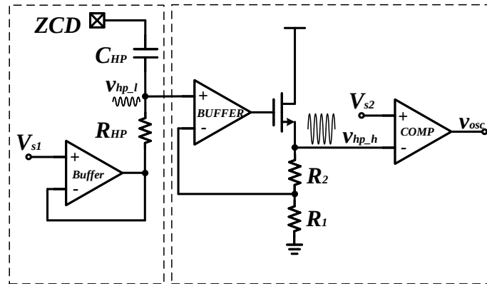
图 4.25 退磁完成时间检测电路
