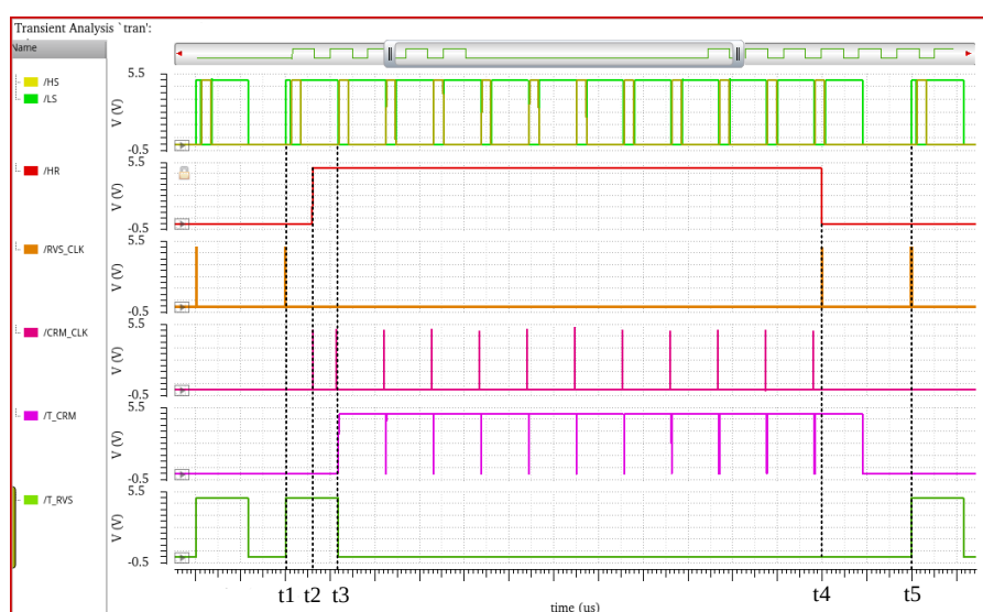
图 4.36 逻辑控制电路具体仿真波形图
