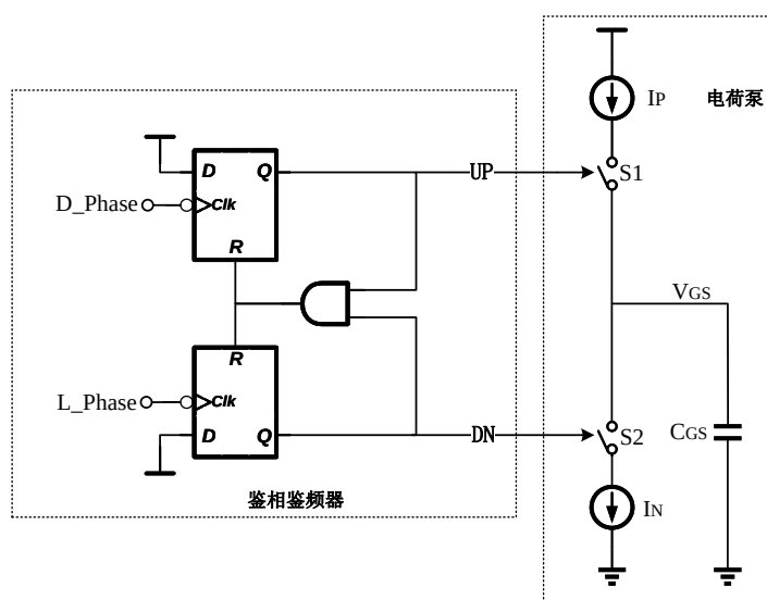
图 4.18 鉴相鉴频器和电荷泵电路图
