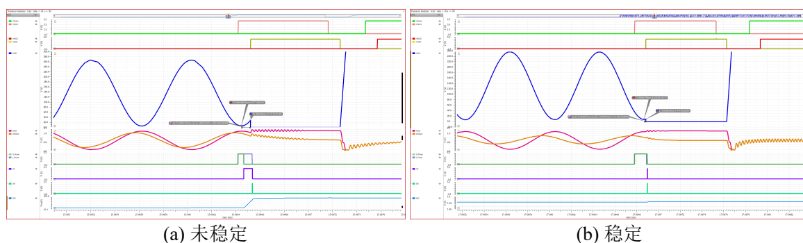
图 4.23 谷底导通放大仿真图
