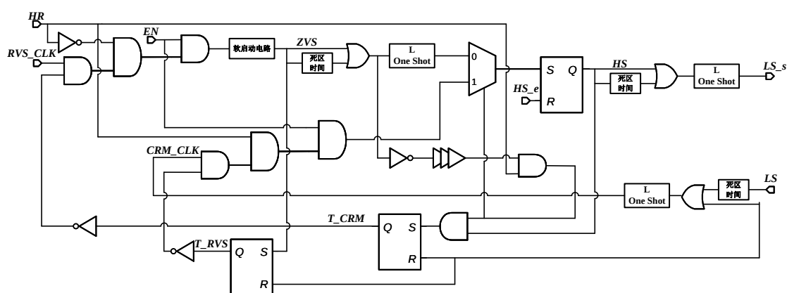
图 4.34 逻辑控制电路原理图
