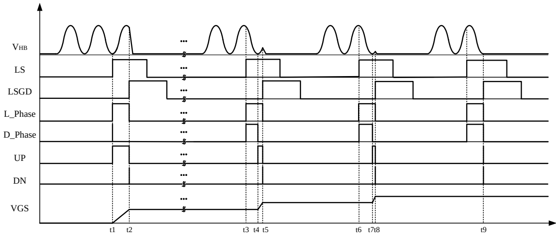
图 4.21 精确谷底导通电路相关波形图
