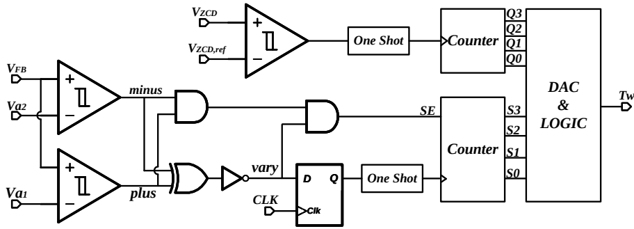
图 4.8 谷值锁定电路 1
