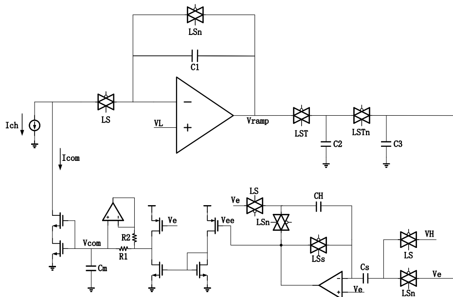
图 4.26 动态校准闭环补偿电路
