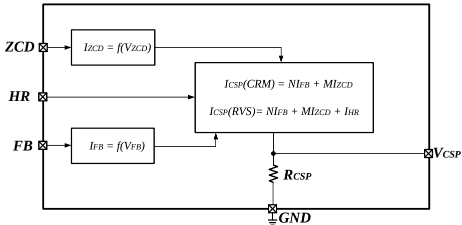
图 4.30 峰值电流控制电路框图
