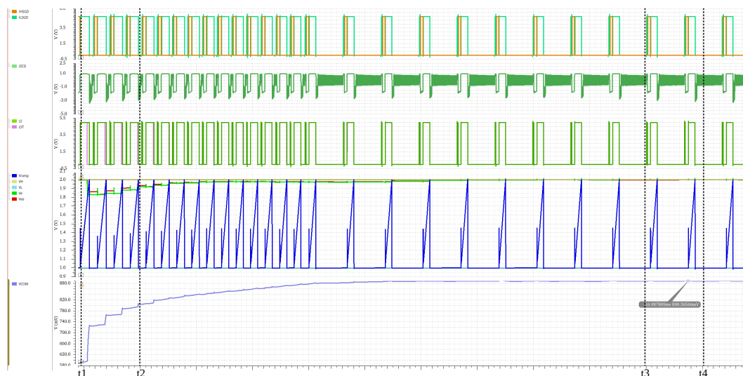
图 4.28 退磁时间动态校准电路 f 仿真波形图
