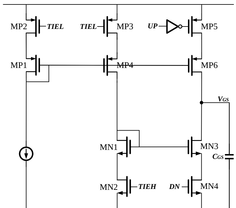
图 4.20 电荷泵电路图
