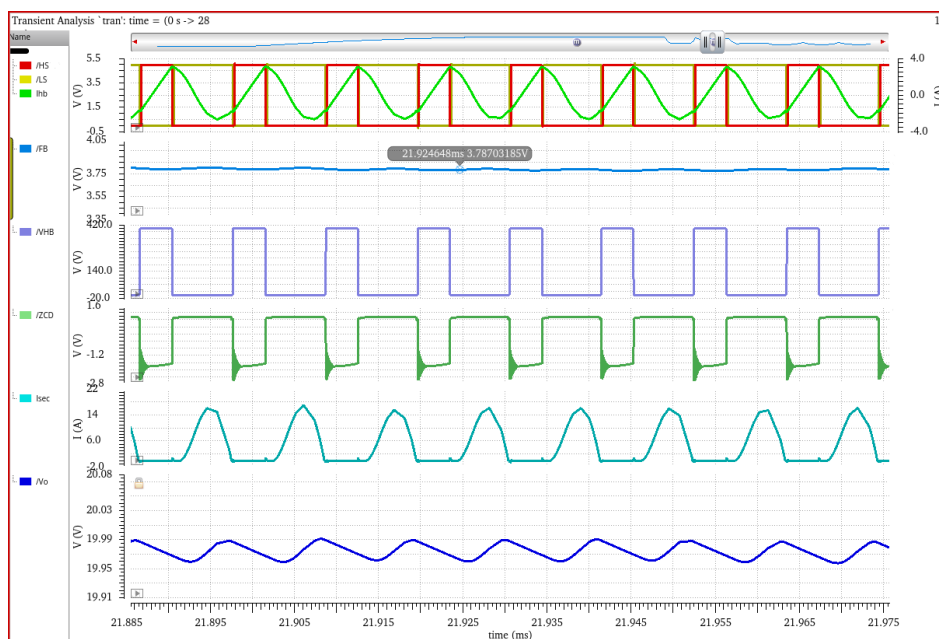
图 4.38 满载电路仿真波形图
