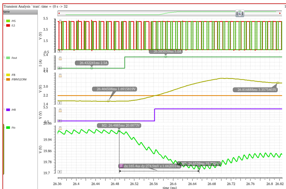
图 4.41 负载 2.5-5A 跳变仿真波形图
