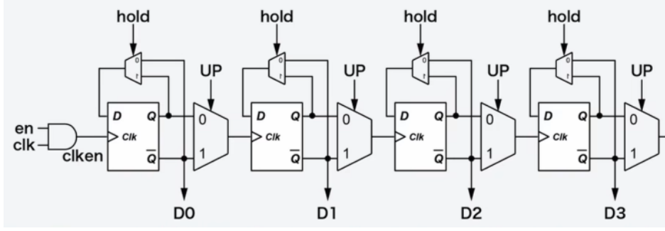
图 4.10 双向计数器电路图
