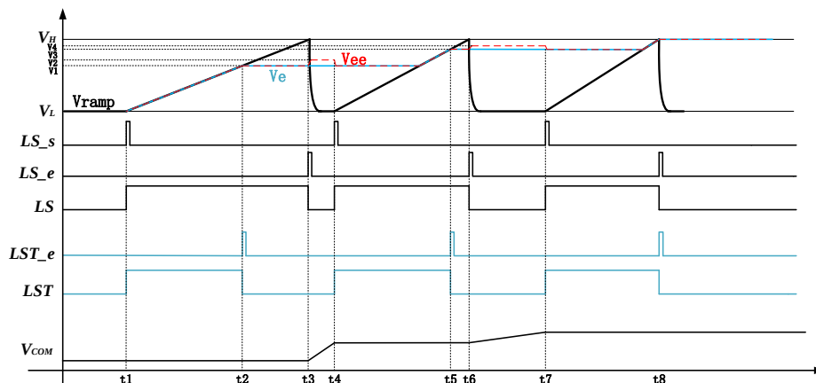
图 4.27 动态校准闭环补偿波形示意图
