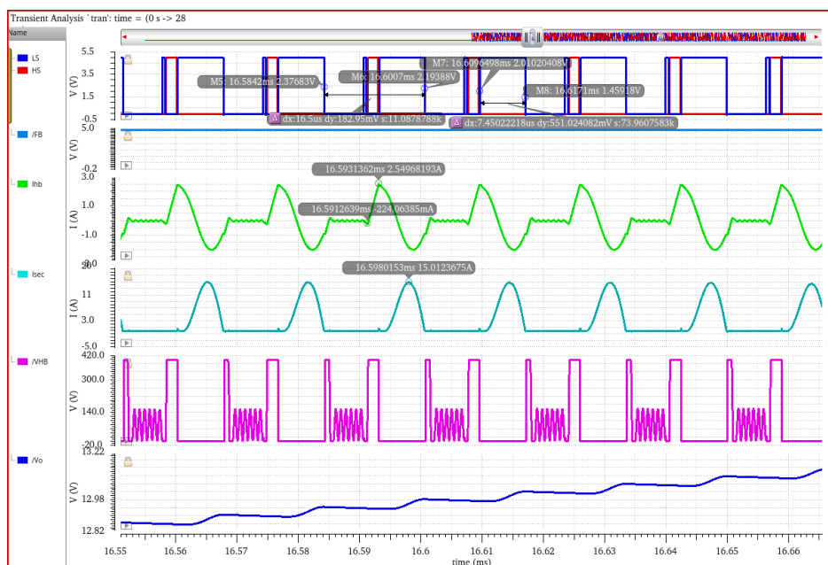
图 4.37 恒流控制模式仿真波形图
