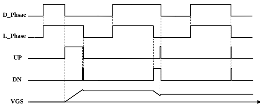
图 4.19 鉴相鉴频器电荷泵波形图
