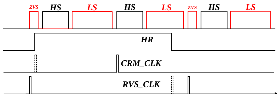
图 4.35 不同工作模式切换波形图
