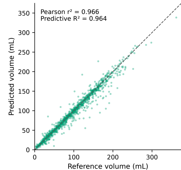
nnU-Net
