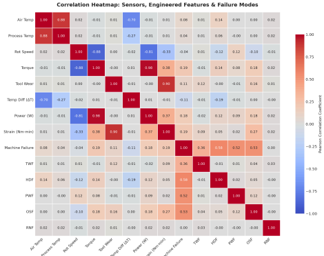
Fig. 3. 센서 특성, 도메인 파생 변수 및 고장 타겟 간 피어슨 상관계수 히트맵
