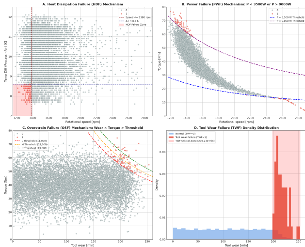
Fig. 2. 4대 물리적 고장 메커니즘의 수학적 경계 조건 실증 (A: 방열 고장, B: 전력 이상 곡선, C: 과부하 한계선, D: 공구 마모 고위험 구간)
