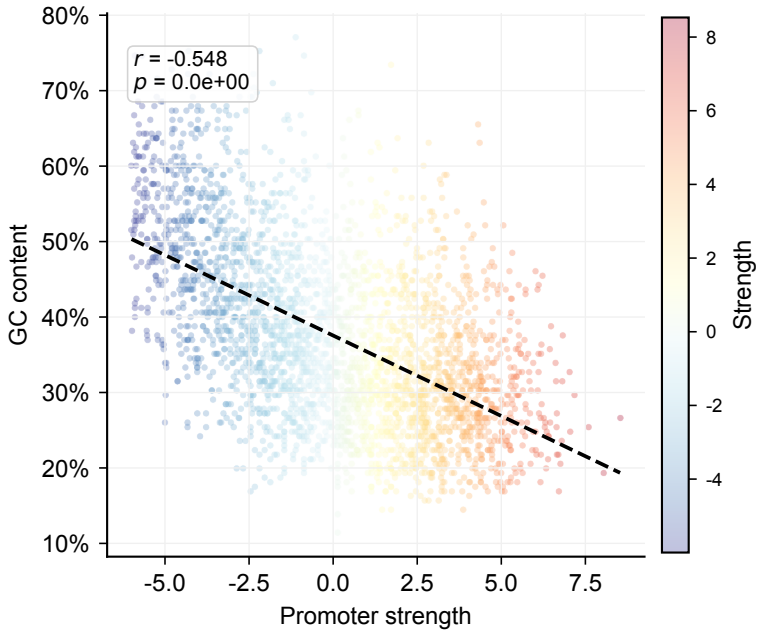
E. coli — scatter
