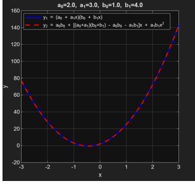
图 1: Karatsuba 恒等式
