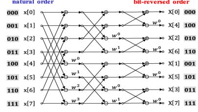
图 3: 蝶形运算 (Butterfly) —— radix-2 Cooley-Tukey 的核心单元
