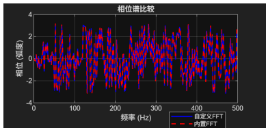
图 6: FFT 演示
