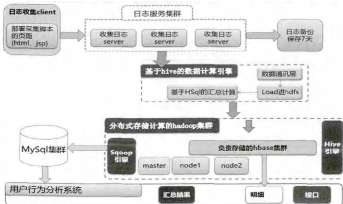
图2 用户行为采集和分析系统整体架构
