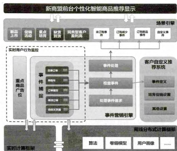
图1 新商盟基于用户行为的事件营销体系总体架构
