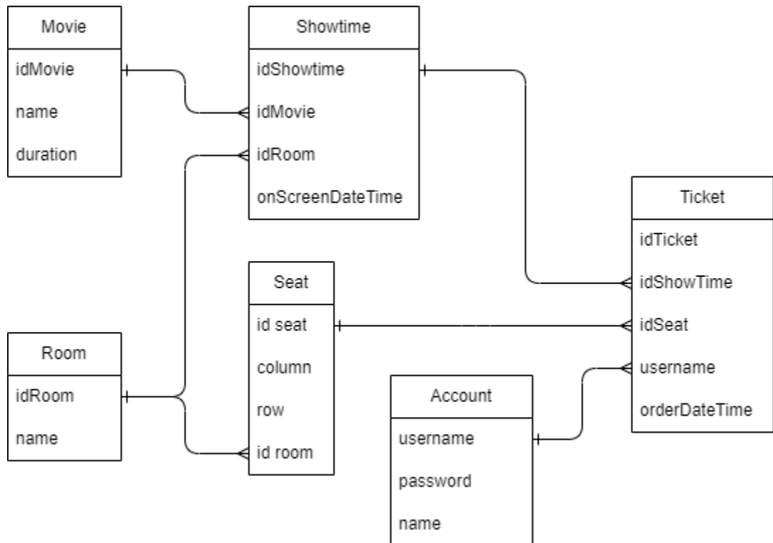
Hình 2-1 Mô hình quan hệ
