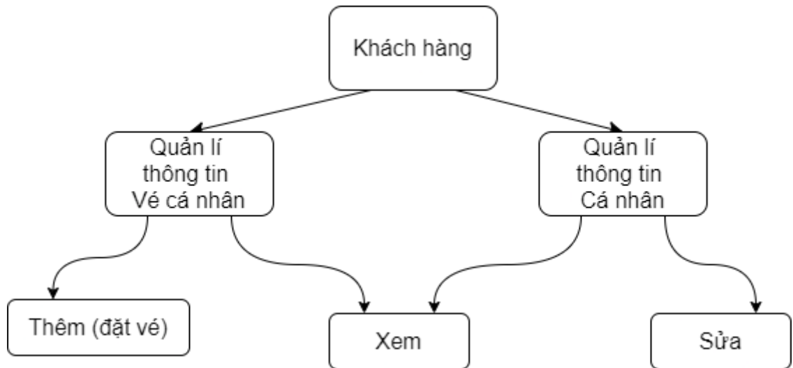
Hình 1-2 Các chức năng dành cho Khách hàng
