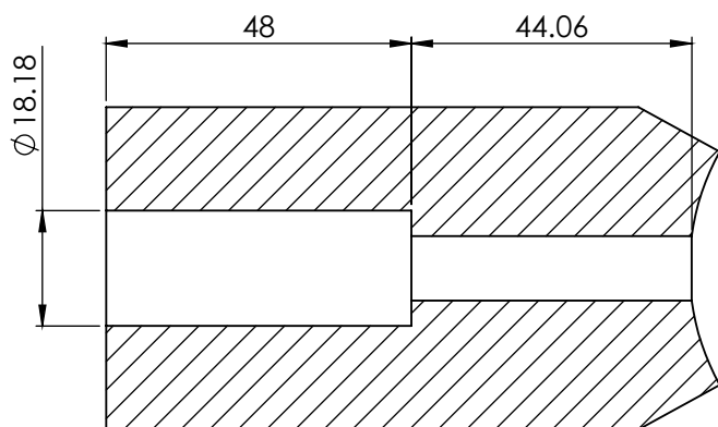
SECCIÓN C-C ESCALA 1 : 1
