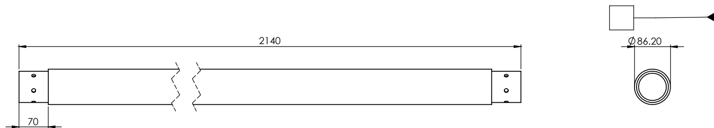
Subensamble Tubo 3"
