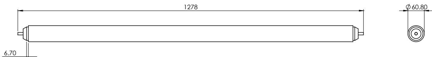
Subensamble Tubo 2"
