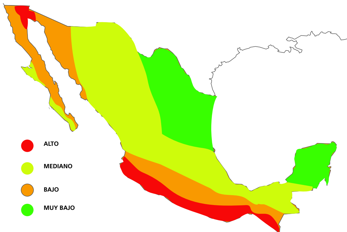
Figura3: Mapa de regiones y zonas sísmicas,
