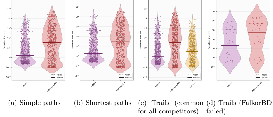
Fig. 6: Performance on Wikidata
