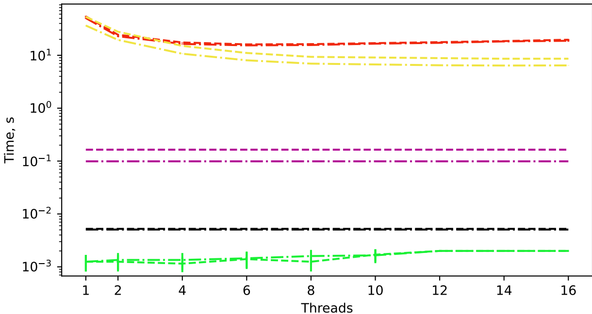
SSSP, gr_30_30, un+reordered
