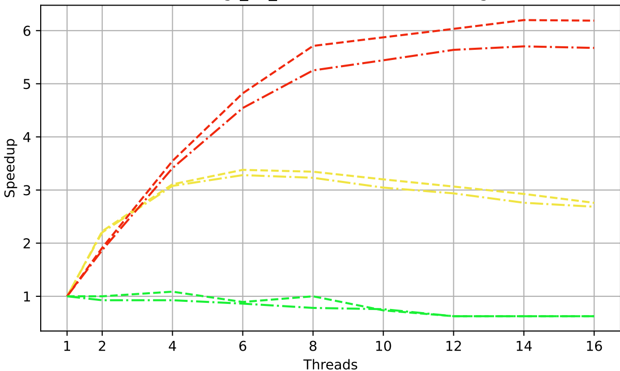
SSSP, gr_30_30, un++reordered, scaling
