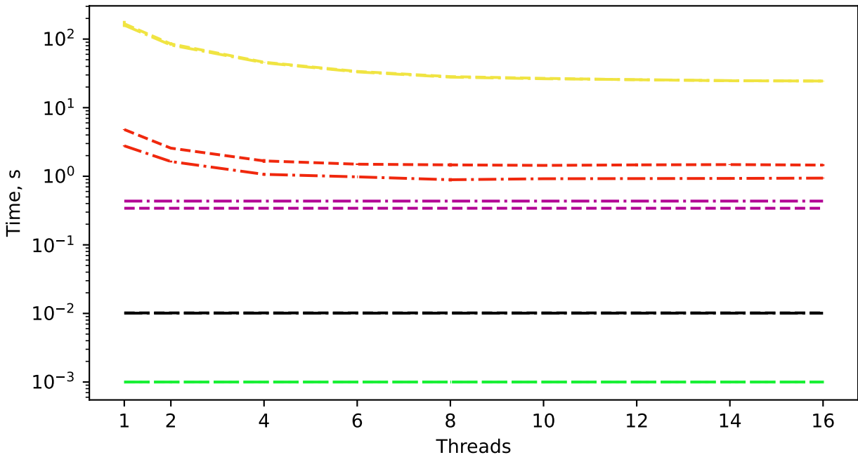
SSSP, Trefethen2000, un+reordered
