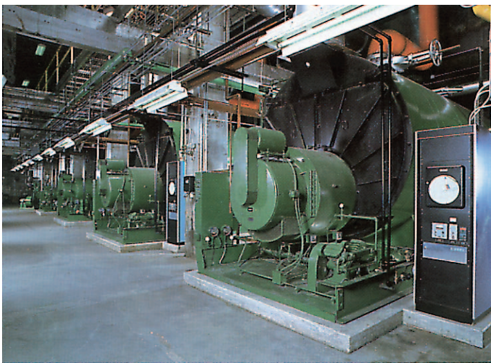
Merchandise Mart Calderas de Vapor de Baja Presión, Quemadores de Gas Natural/#2 Oil
