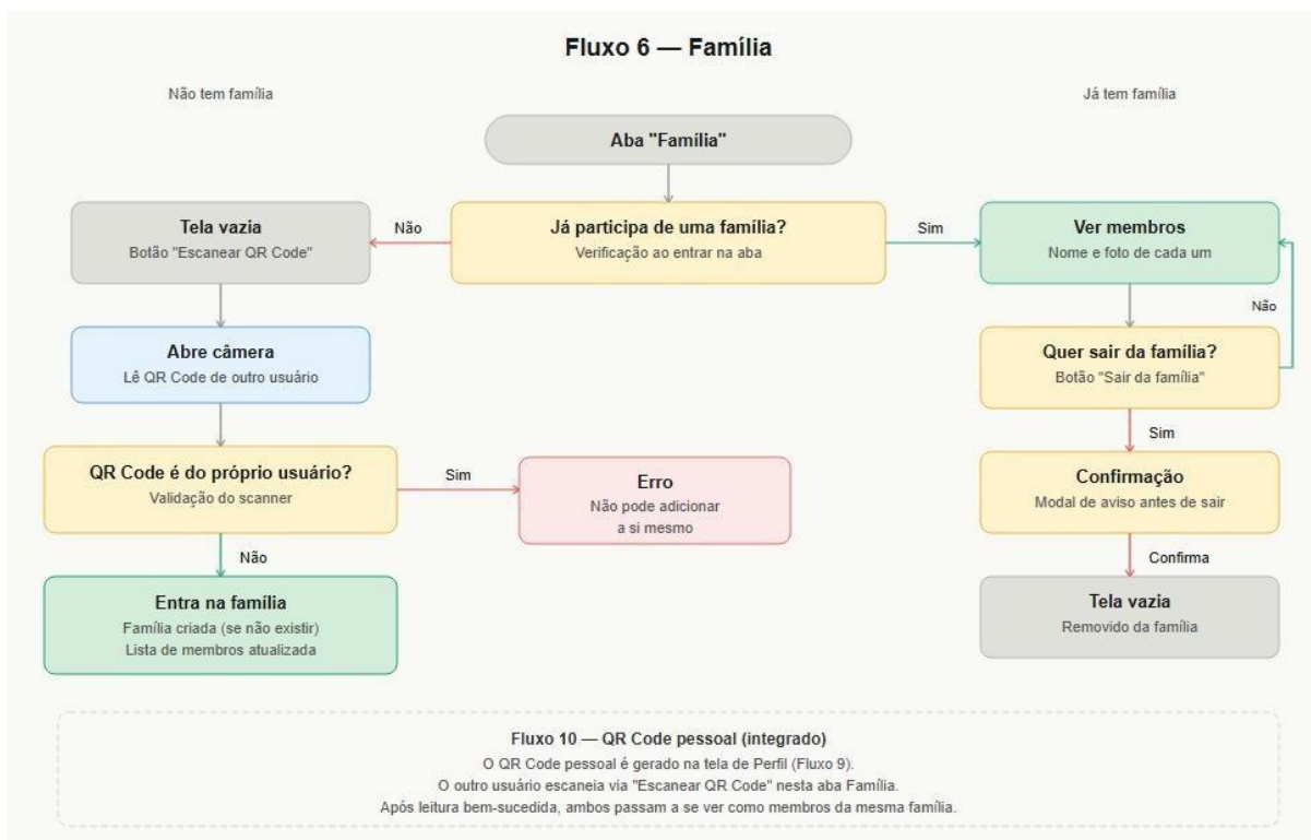
Figura 18: Fluxo família
