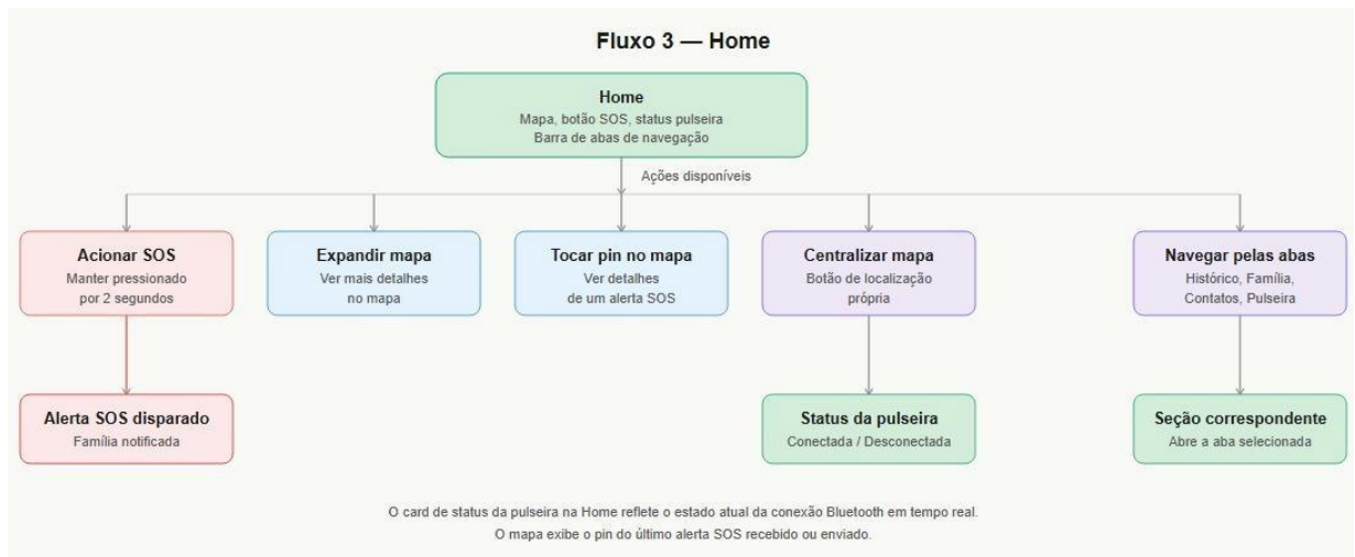
Figura 15: Fluxo home
