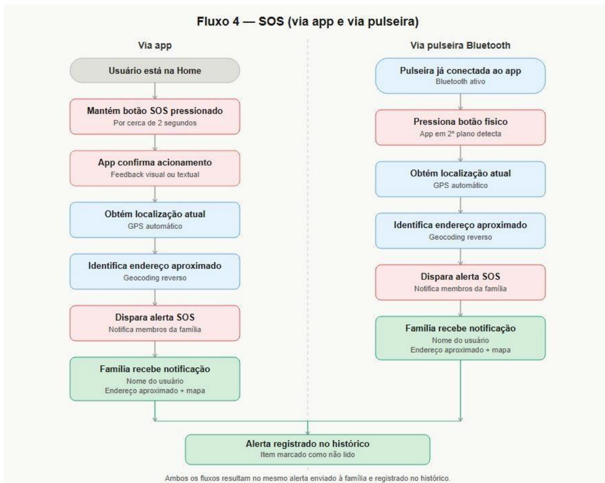
Figura 16: Fluxo SOS
