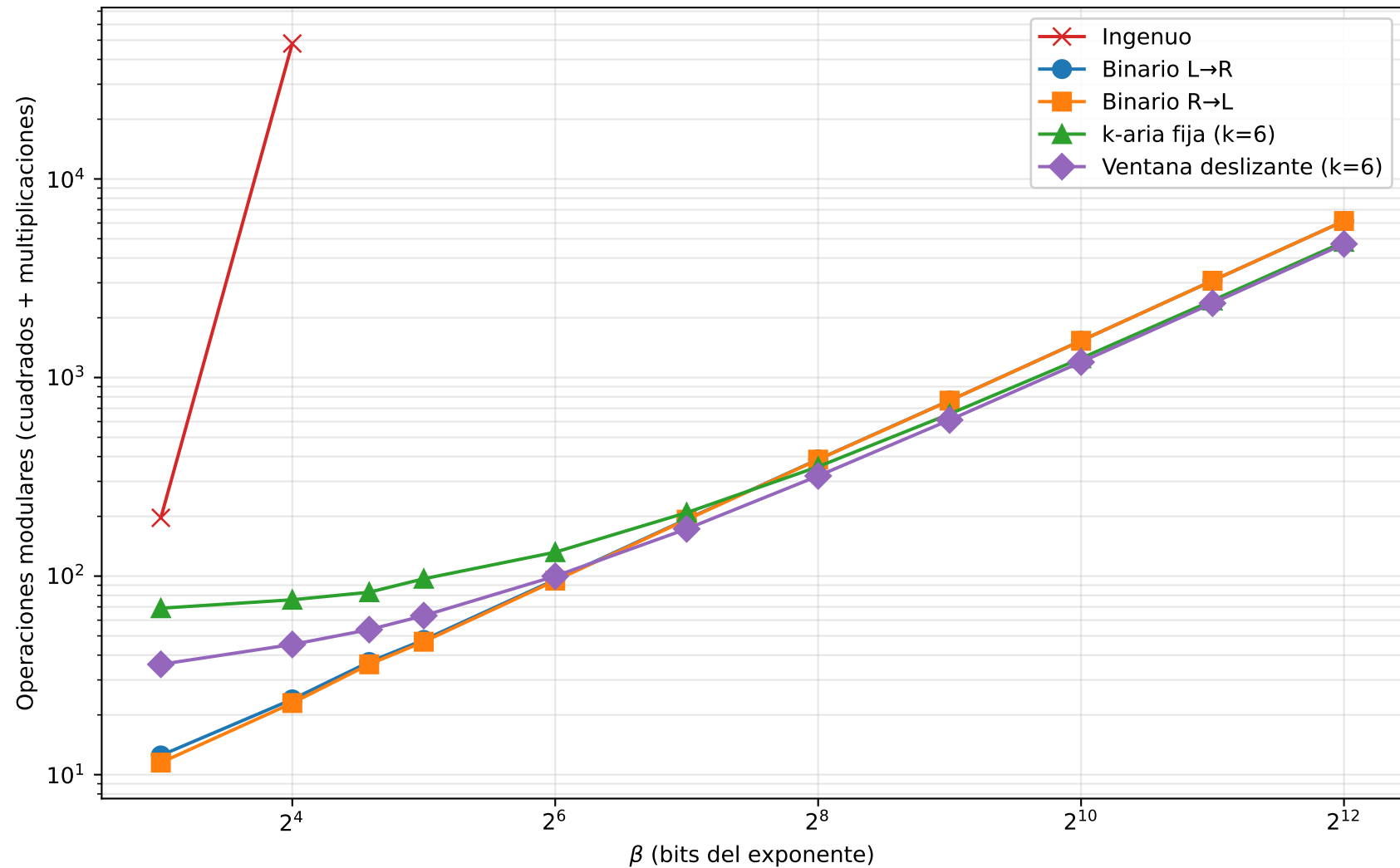
Figura 1. Escalabilidad: operaciones vs. tamaño del exponente
