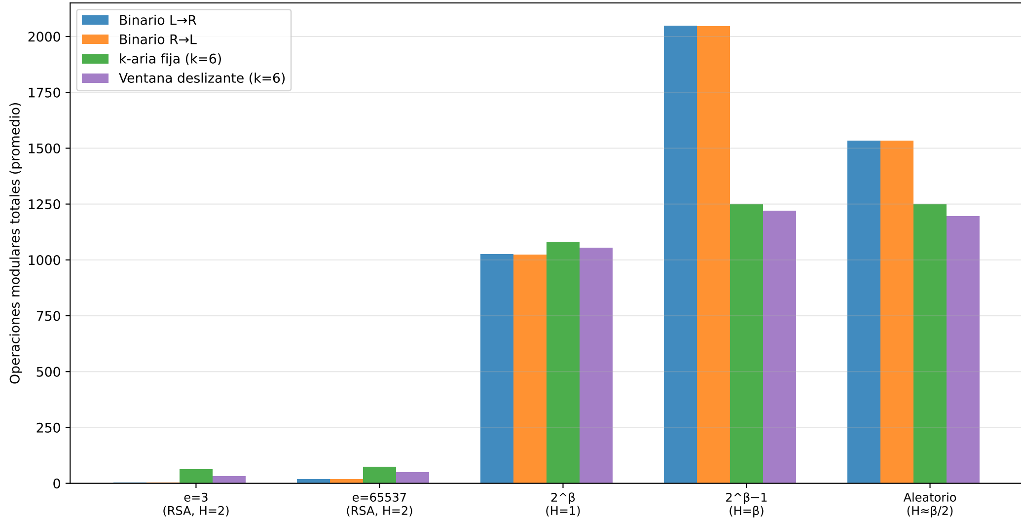
Figura 5. Operaciones por tipo de exponente ( \beta = 1024 bits del módulo)
