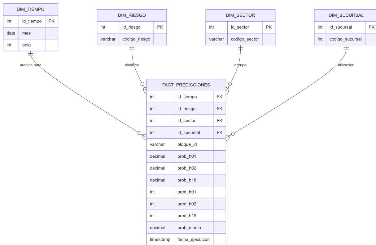
Figure A.5: Esquema estrella de la tabla fact_predicciones . Almacena las probabilidades y predicciones binarias para los 18 horizontes temporales, generadas por el modelo seleccionado.
