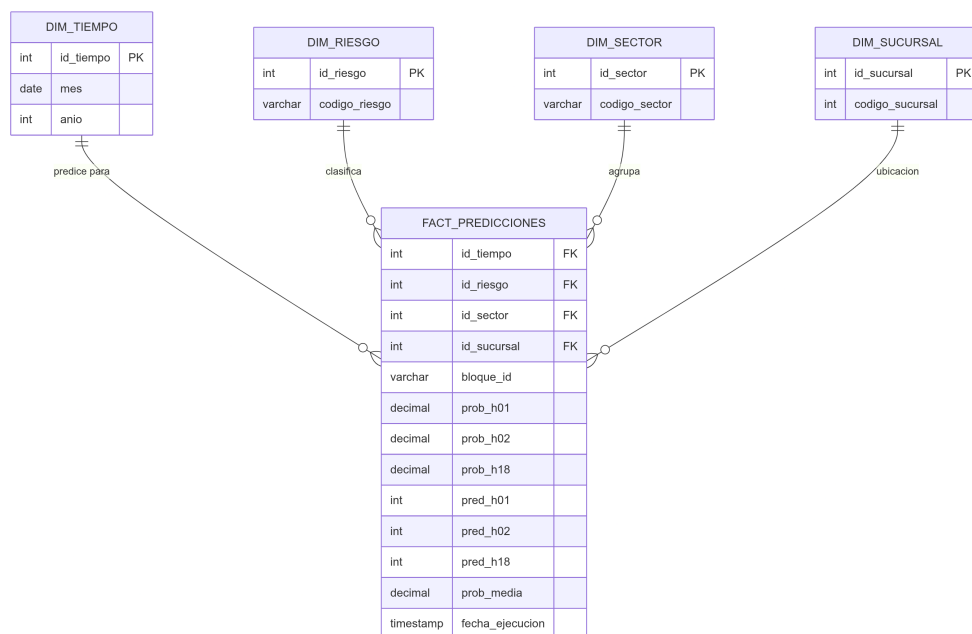
Figure A.5: Esquema estrella de la tabla fact_predictions . Almacena las probabilidades y predicciones binarias para los 18 horizontes temporales, generadas por el modelo seleccionado.
