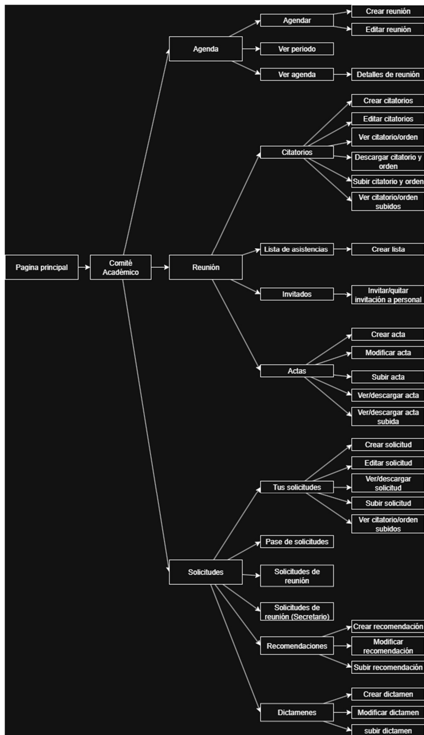
Figura 3 Diagrama de vistas
