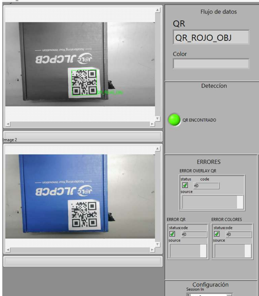
Ilustración 1. Frontal PANEL LABVIEW
