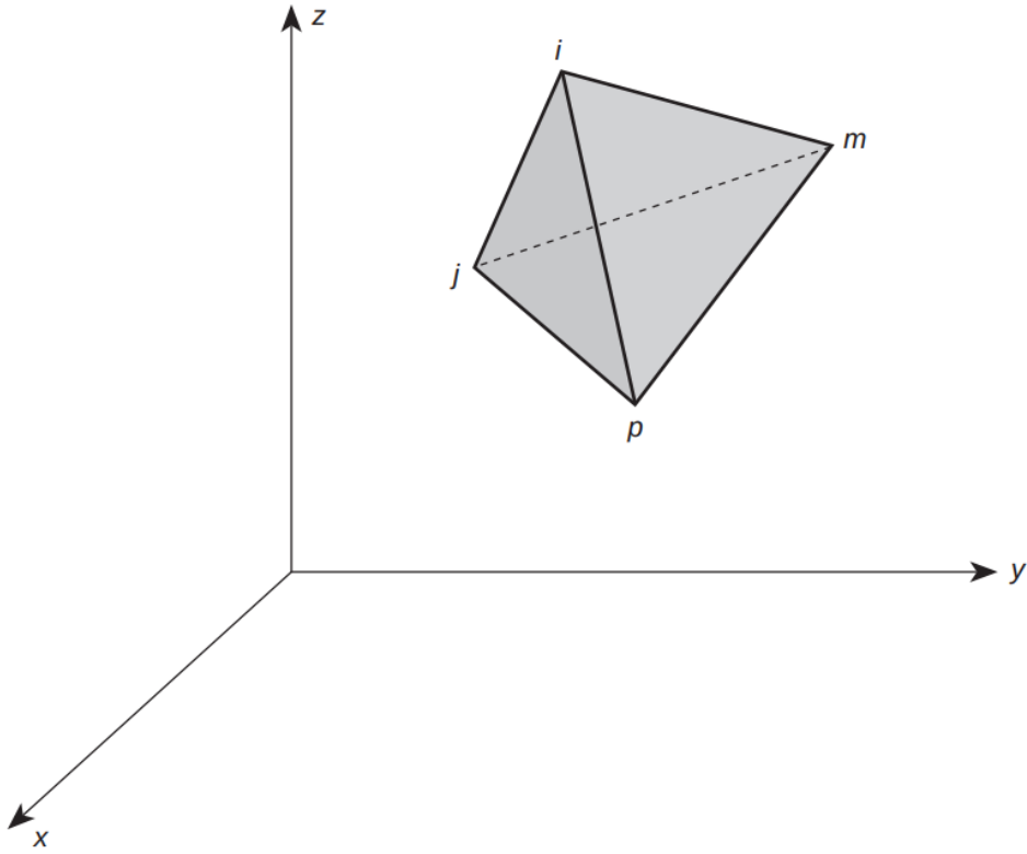
Рис.2. Тетраэдральный элемент.
