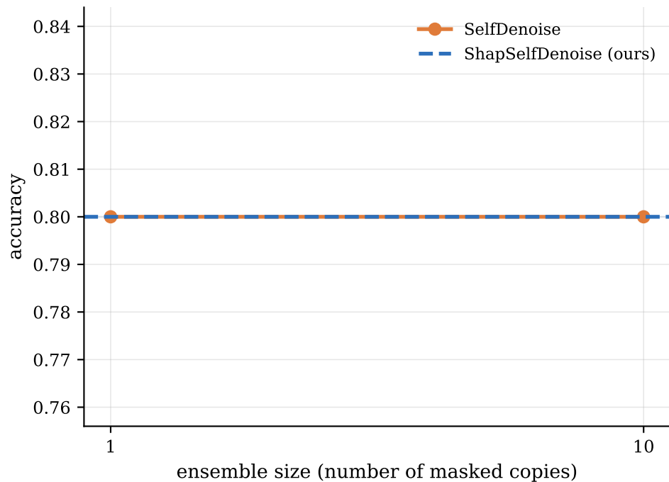
AG News
