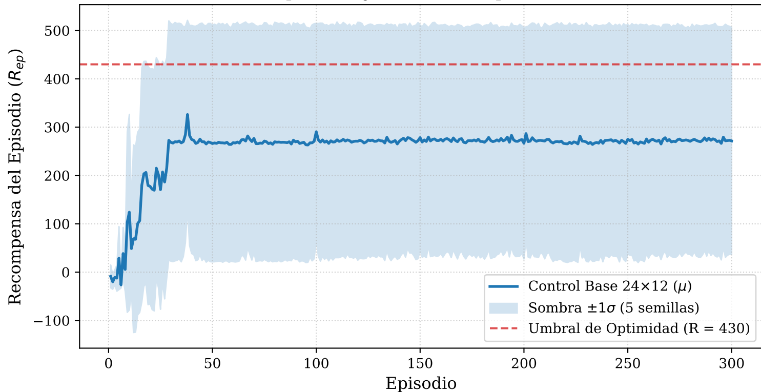
Curva de Aprendizaje R-STDP (Arquitectura 24×12)
