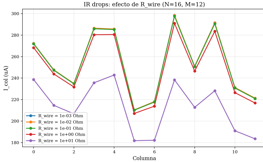
Figura 9.10: Perfil de corriente por columna para distintos valores de resistencia de línea R_{wire} . A mayor resistencia, mayor no-uniformidad en la lectura.
