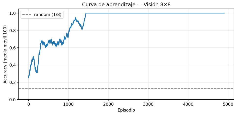
Figura 9.14: Curva de aprendizaje del clasificador sobre los ocho patrones, semilla 0. Media móvil de 100 episodios; la línea discontinua marca el nivel aleatorio 1/8.
