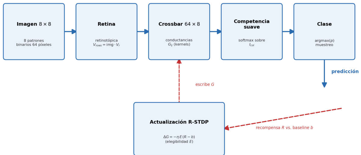
Figura 9.13: Arquitectura del clasificador neuromórfico. La imagen se codifica en voltajes de fila, se propaga por el crossbar 64 \times 8 , y la corriente de cada columna se normaliza en una distribución de probabilidad sobre las clases.
