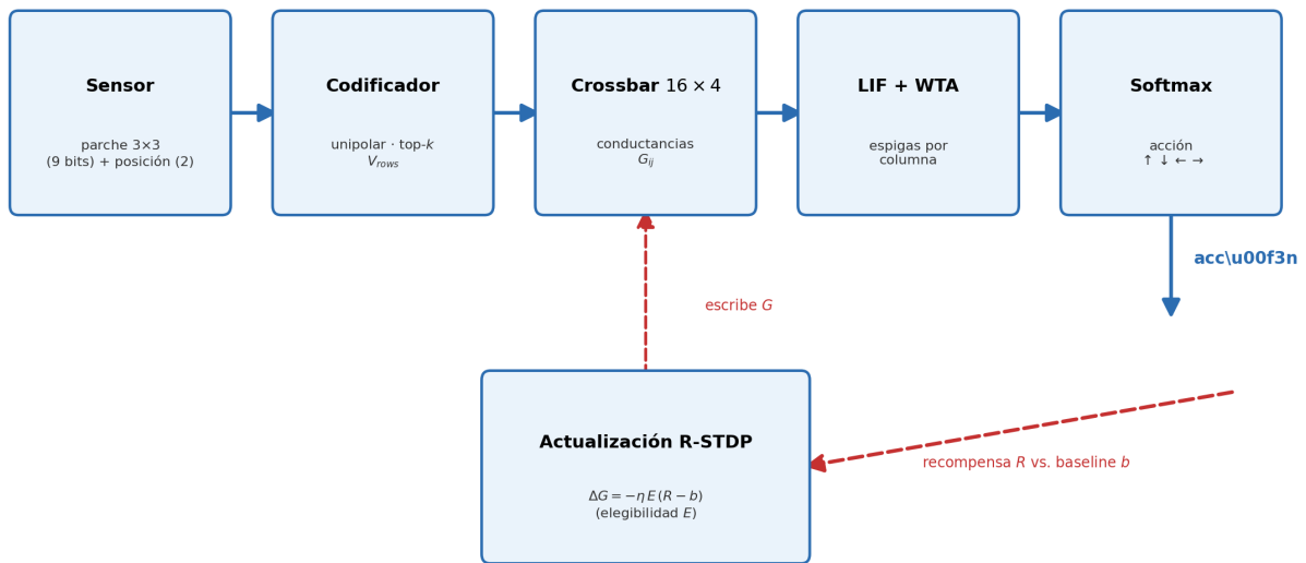
Figura 9.19: Arquitectura del agente de navegación. El mismo crossbar R-STDP de las etapas anteriores, con N = 16 filas y M = 4 columnas, procesa el parche sensorial 3 \times 3 y la posición para producir la acción.
