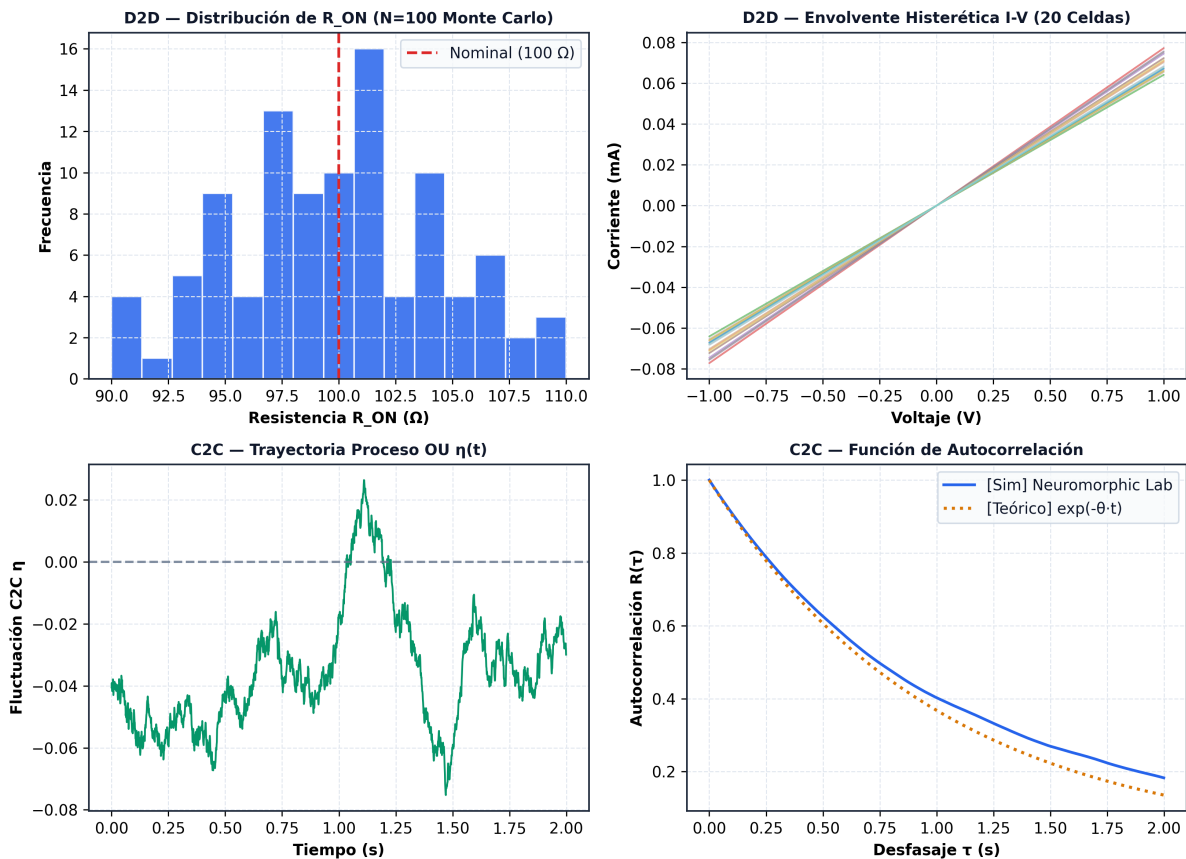
Figura 3.6: Caracterización cuantitativa de variabilidad D2D (test KS) y variabilidad temporal C2C (proceso estocástico).
