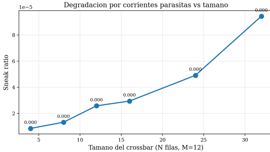
Figura 9.8: Crecimiento monótono del sneak ratio al escalar el arreglo crossbar desde N = 4 hasta N = 32 filas, con M = 12 columnas fijas.
