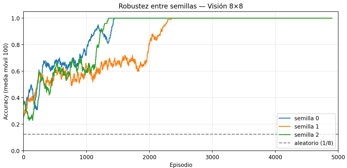
Figura 9.15: Robustez entre semillas: las tres corridas independientes (5000 episodios cada una) convergen a 100 % de acierto sobre los ocho patrones.
