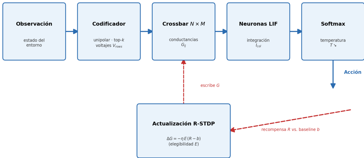
Figura 9.11: Arquitectura del agente neuromórfico. La observación se codifica en voltajes de fila, se propaga por el crossbar, se integra en neuronas LIF, y se decodifica en una acción. El aprendizaje se aplica al final del episodio.
