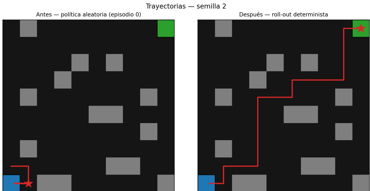
Figura 9.17: Trayectorias sobre el entorno de la semilla 2. Izquierda: episodio 0 con política aleatoria. Derecha: roll-out determinístico de la política aprendida, que alcanza la meta en 19 pasos.
