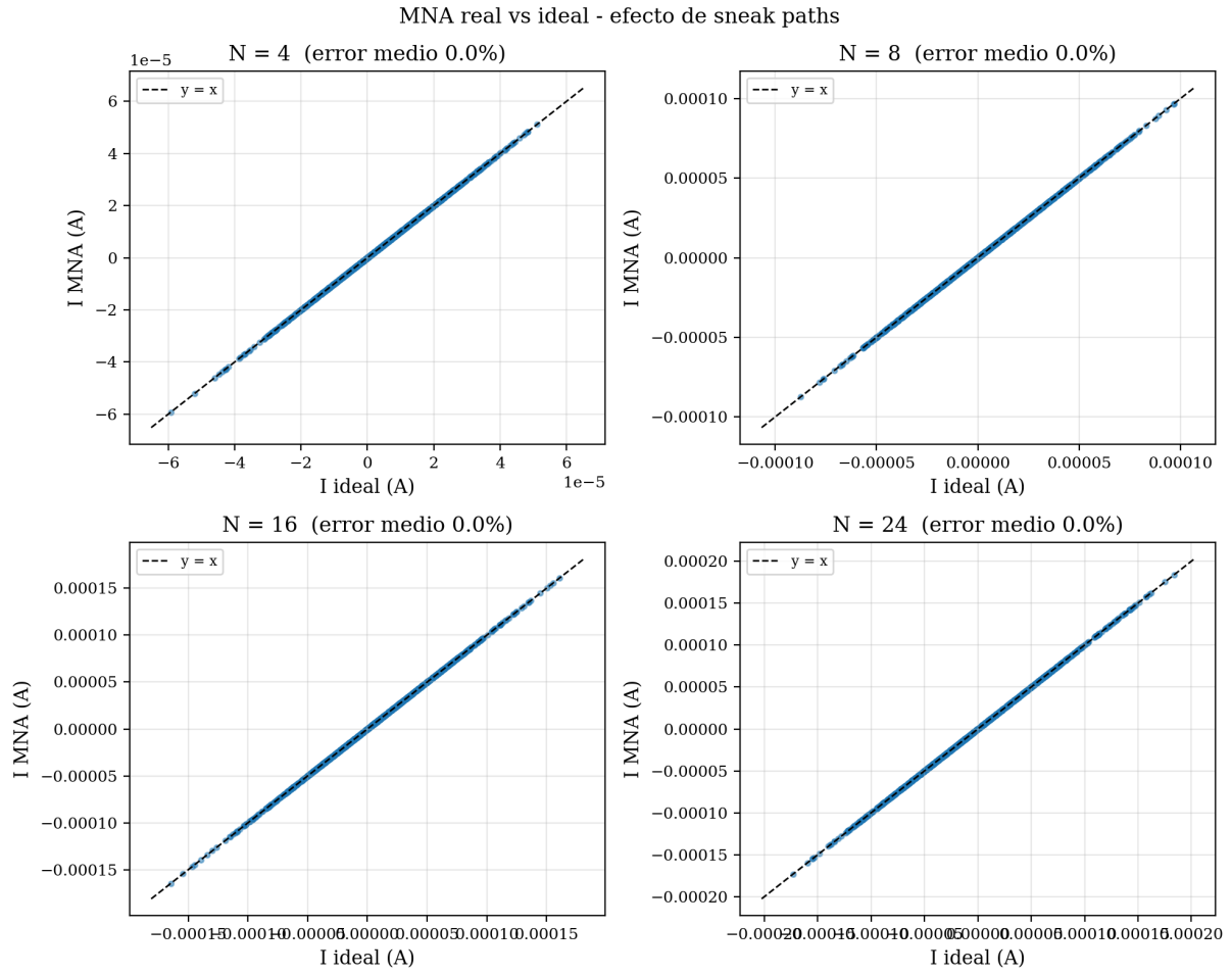
Figura 9.9: Comparación entre corrientes calculadas por el solver MNA completo y el modelo ideal I = G \cdot V para cuatro tamaños de arreglo. La desviación respecto a la recta identidad refleja el impacto acumulado de las corrientes parásitas.
