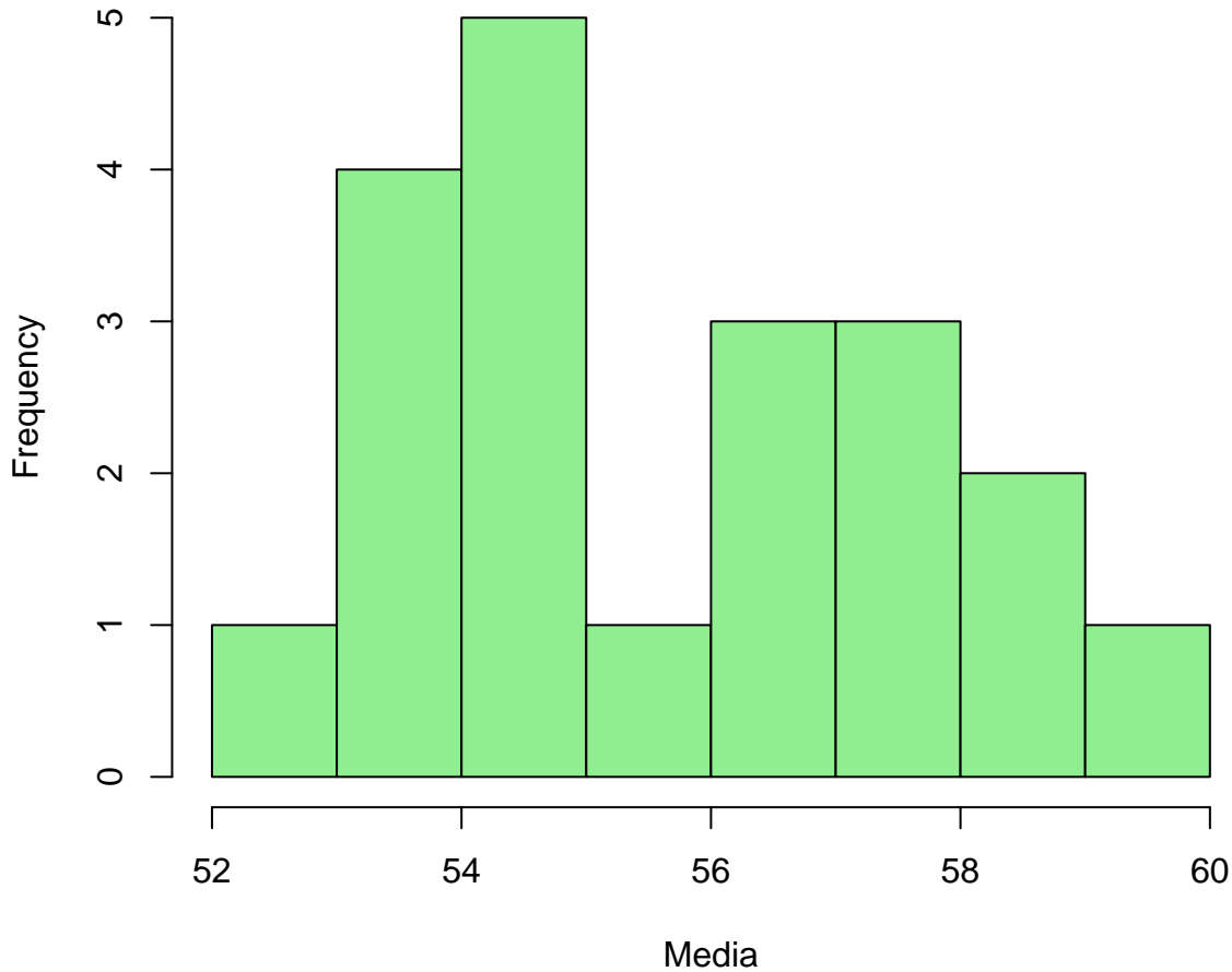
Histograma de medias (20 muestras tamaño 10)
