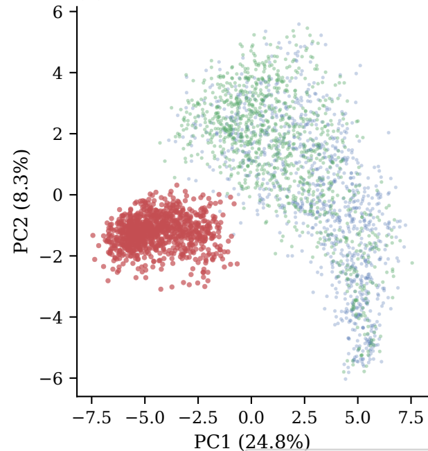
(A) PCA
