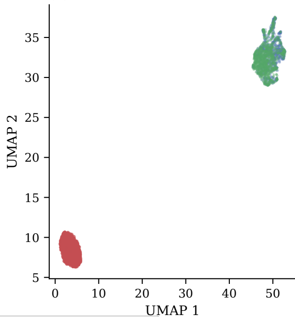
(B) UMAP
