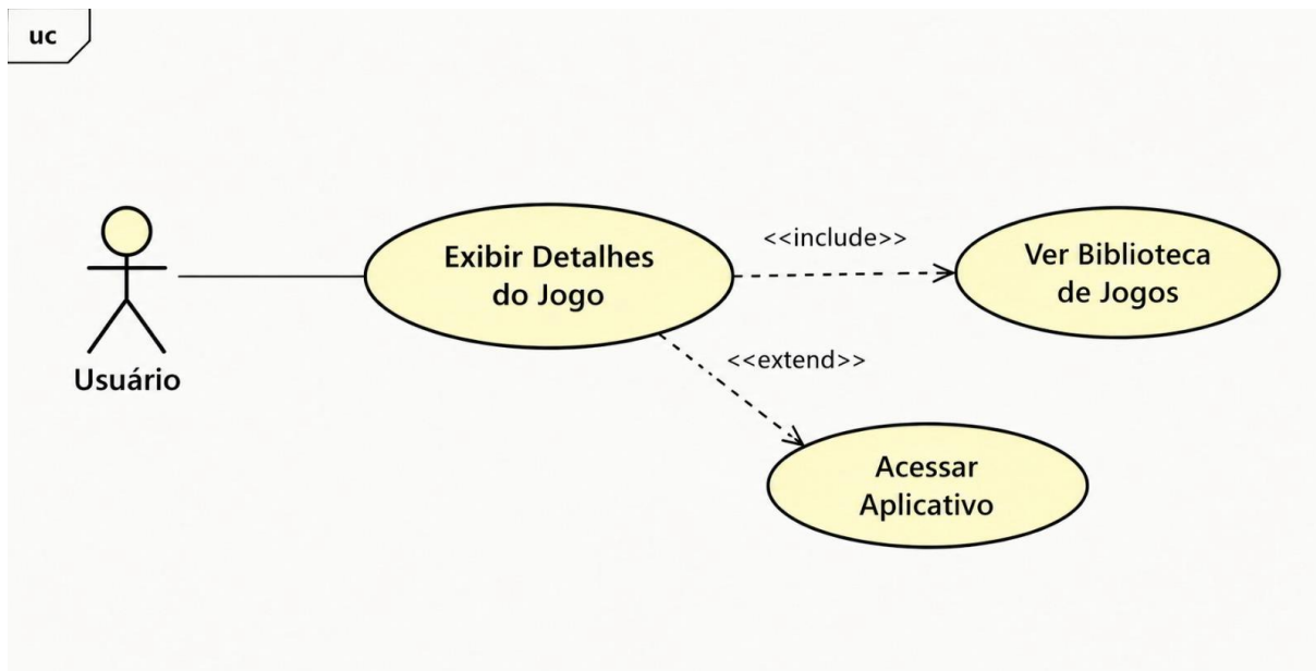
Figura 9 — Diagrama de Caso de Uso: Exibir Detalhes do Jogo (RF09)
