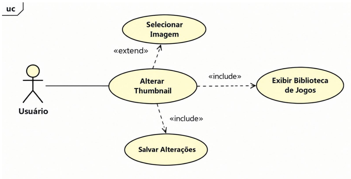
Figura 11 — Diagrama de Caso de Uso: Alterar Thumbnail (RF11)
