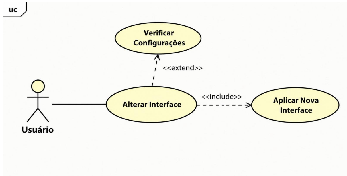
Figura 10 — Diagrama de Caso de Uso: Alterar Interface (RF10)
