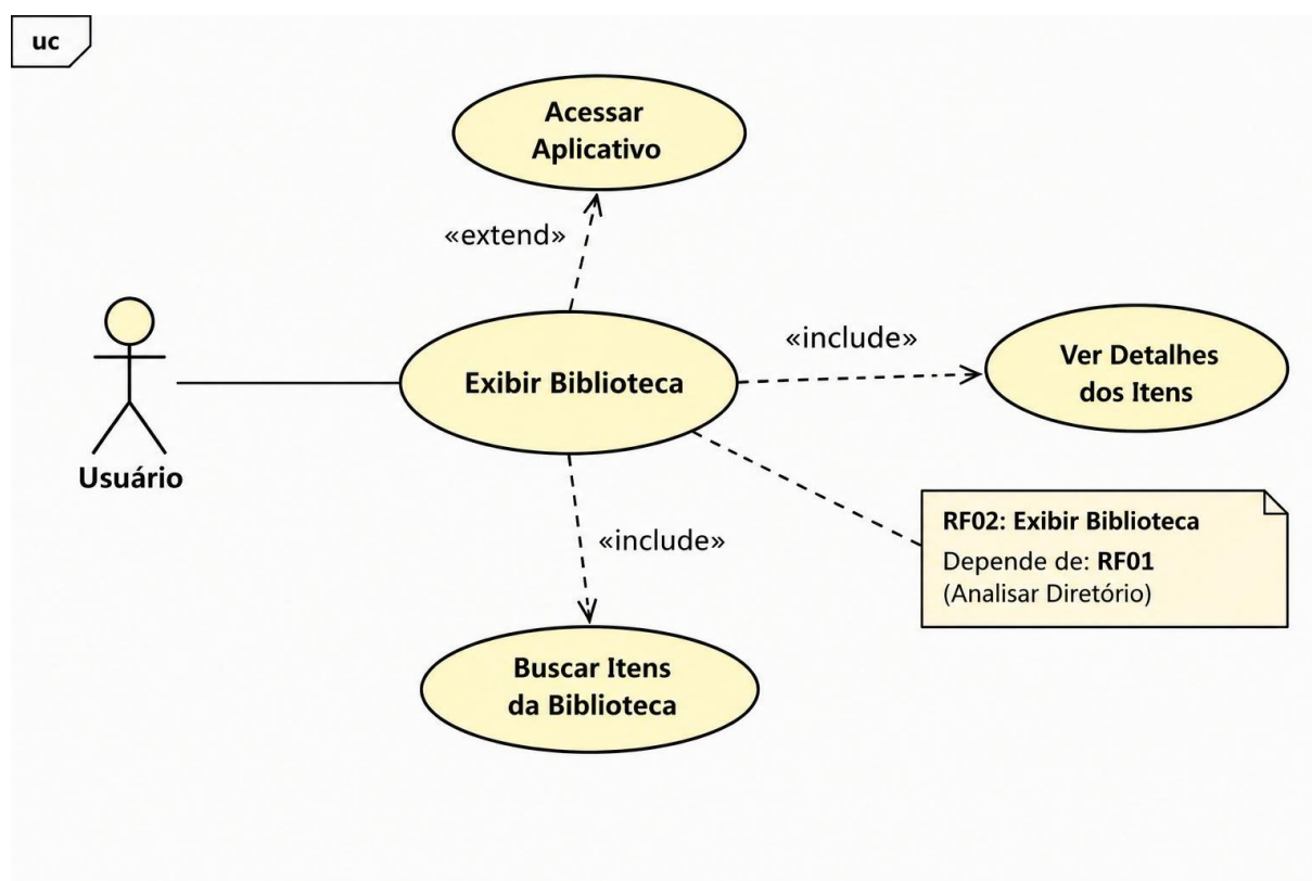
Figura 2 — Diagrama de Caso de Uso: Exibir Biblioteca (RF02)
