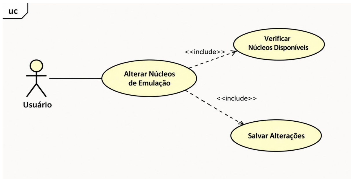
Figura 7 — Diagrama de Caso de Uso: Alterar Núcleos de Emulação (RF07)
