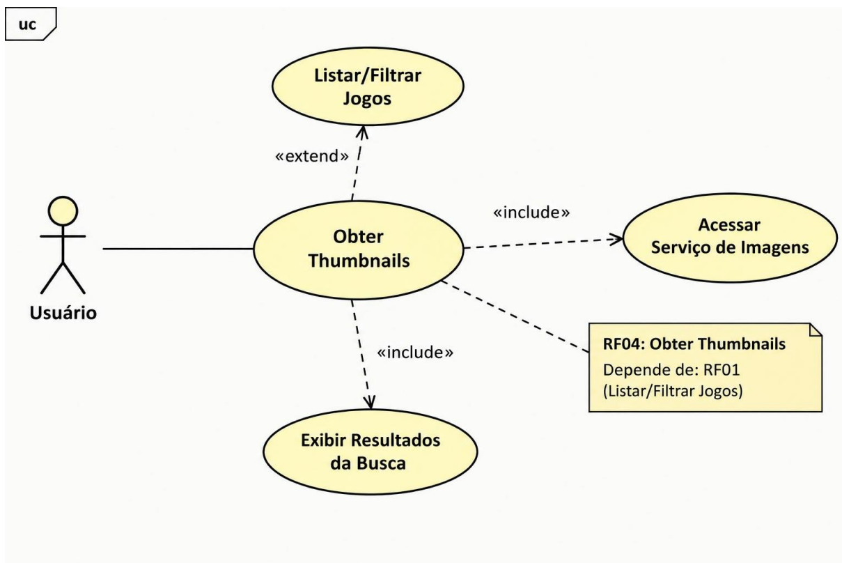
Figura 4 — Diagrama de Caso de Uso: Obter Thumbnails (RF04)
