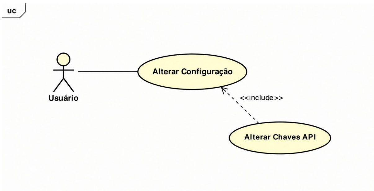
Figura 6 — Diagrama de Caso de Uso: Alterar Chaves API (RF06)
