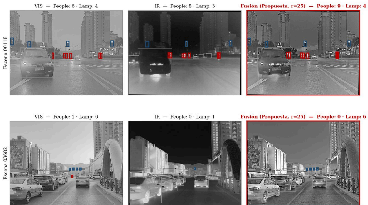
Figura 7. Detecciones del modelo 3nico VIS+IR sobre las escenas 00118 y 03682 de M3FD (conf \geq 0,30 ).
